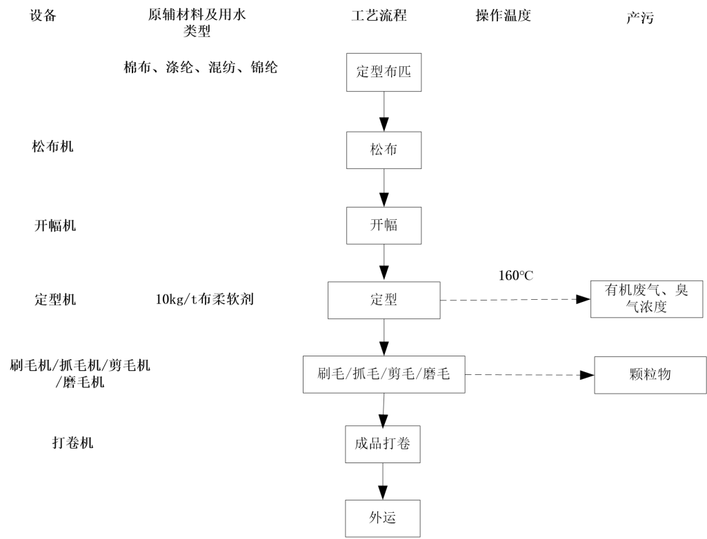
定型布生产工艺流程
