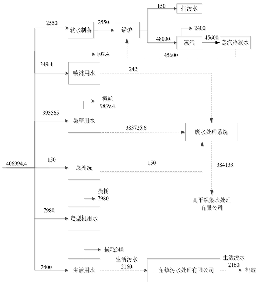
图 3.2-11 技改扩建前水平衡图
