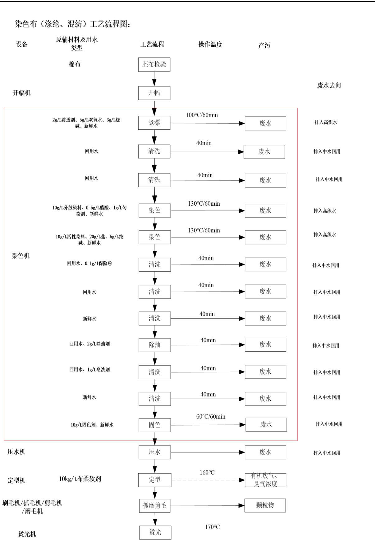
图 4.2-2 染色布混纺涤纶生产工艺流程
