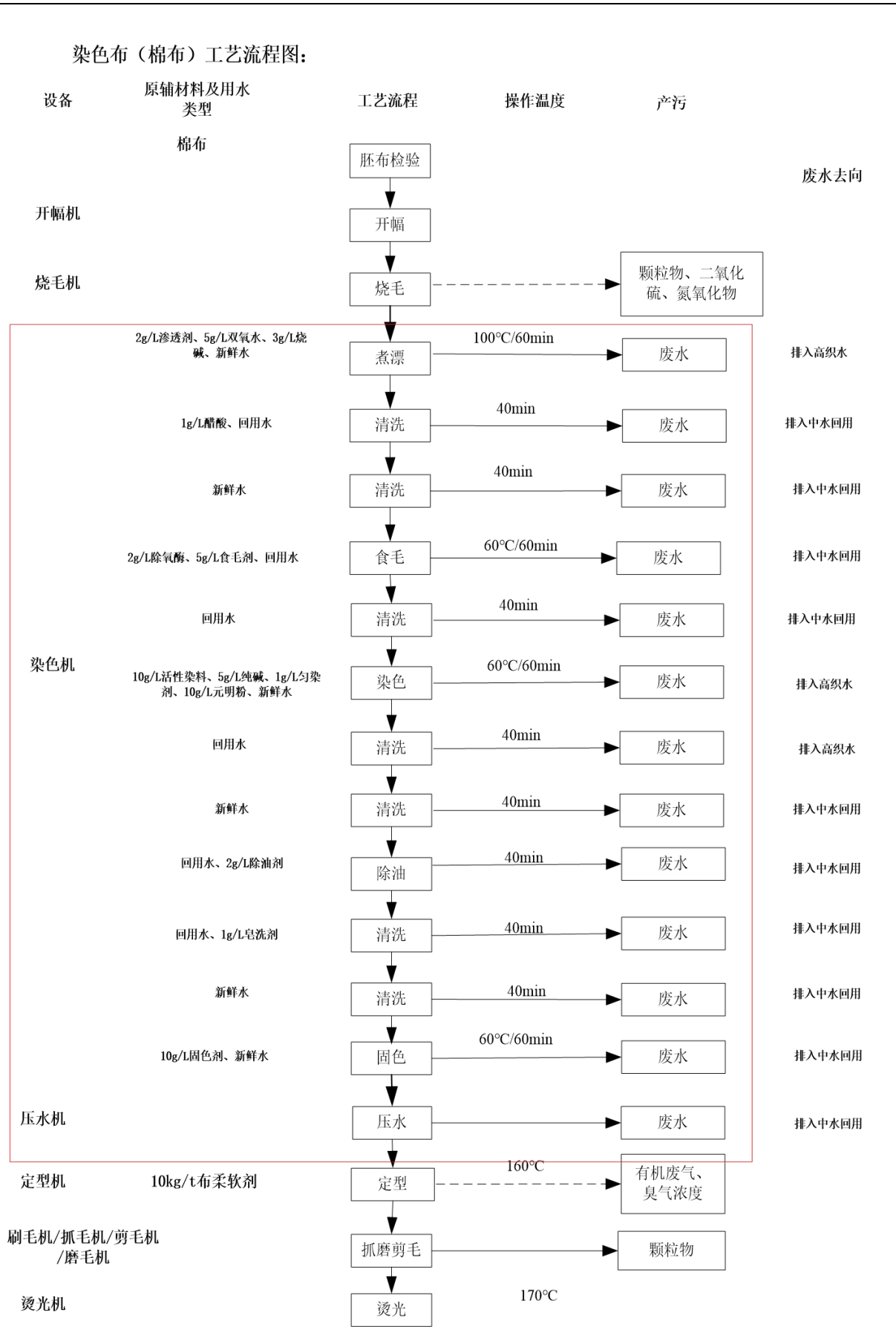
图 4.2-1 染色布棉布生产工艺流程
