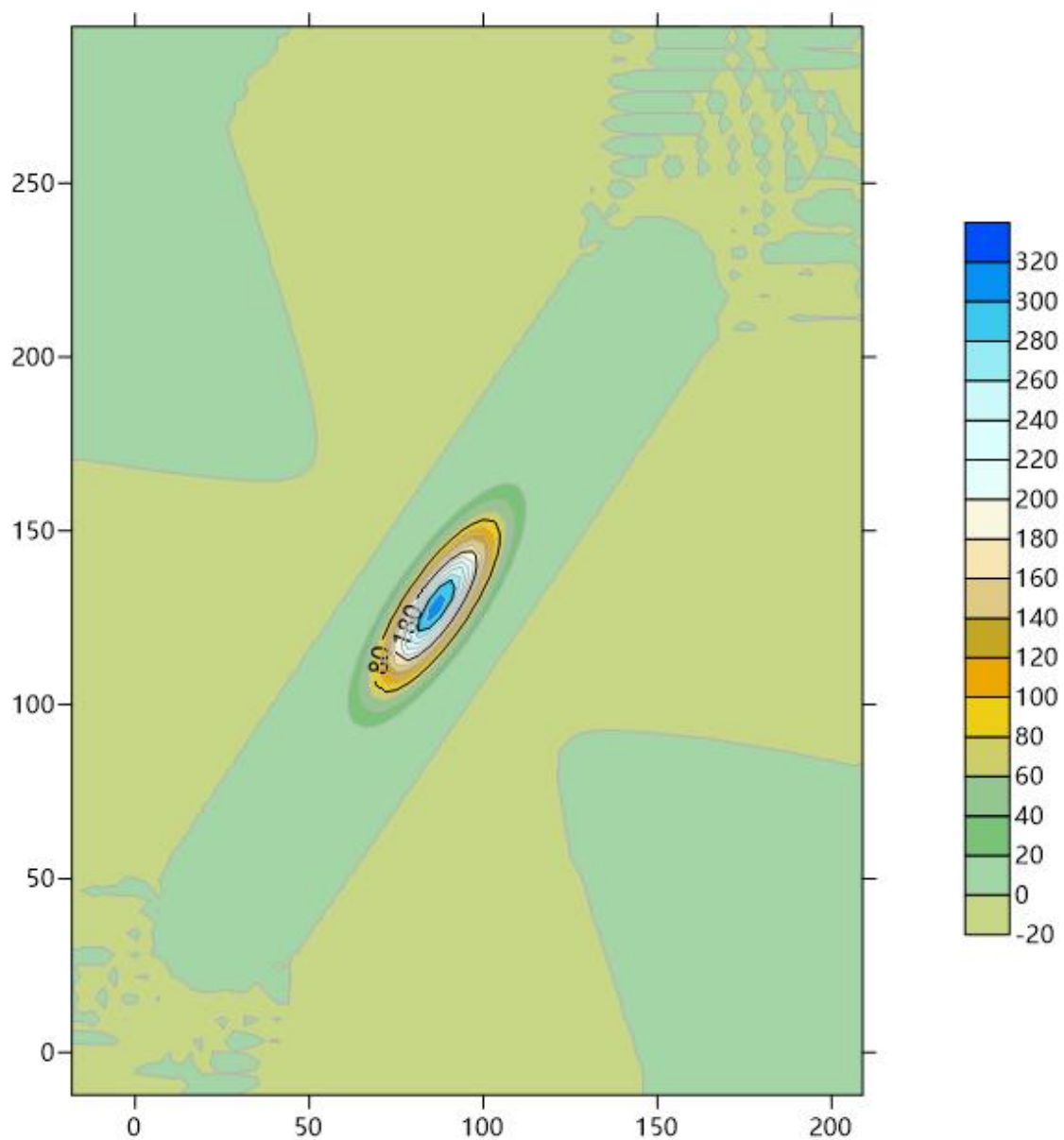
图 6.5-9 假定事故状态下地下水中污染物 COD Mn 5000d 的运移情况
