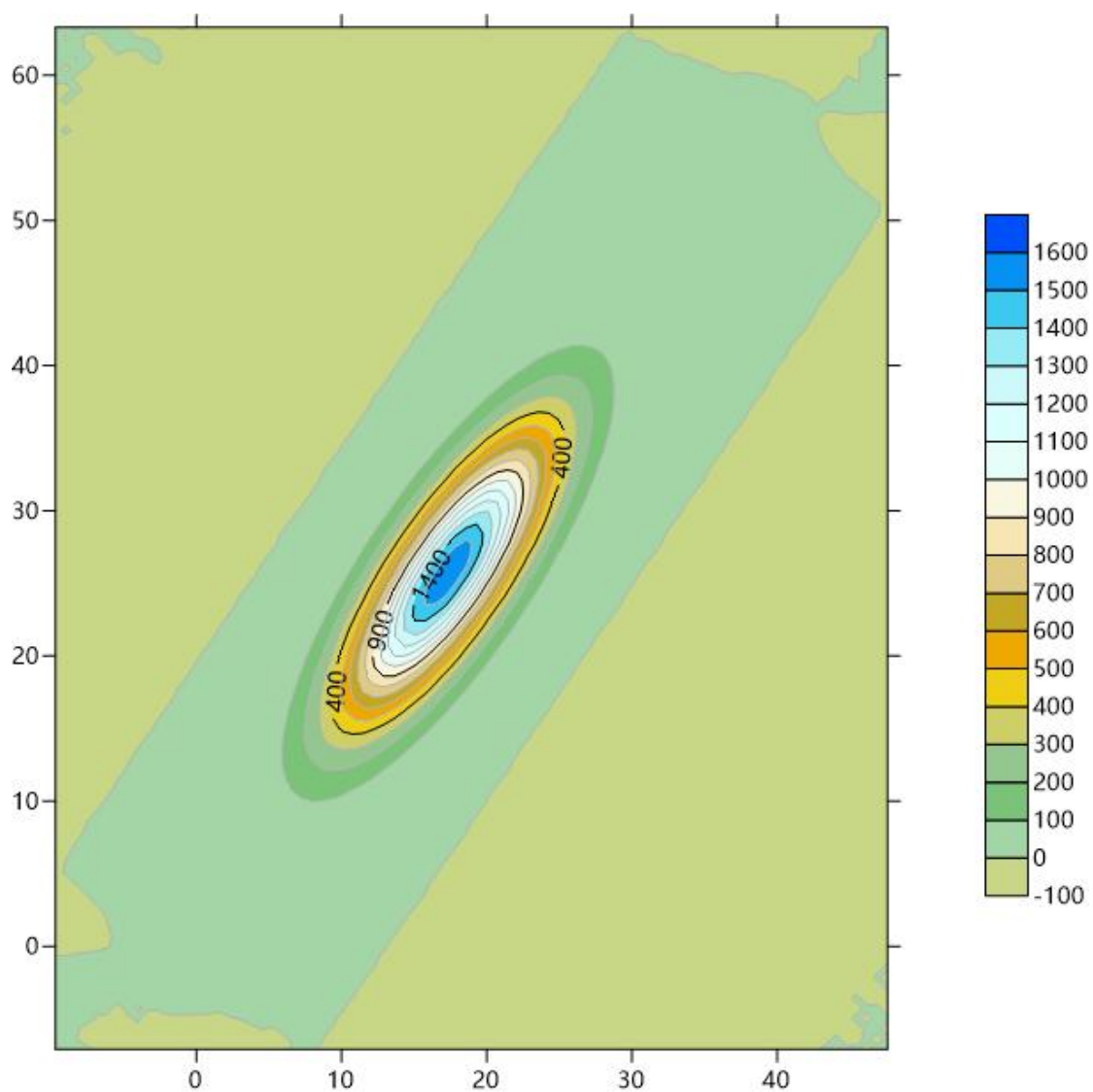
图 6.5-8 假定事故状态下地下水中污染物 CODMn1000d 的运移情况
