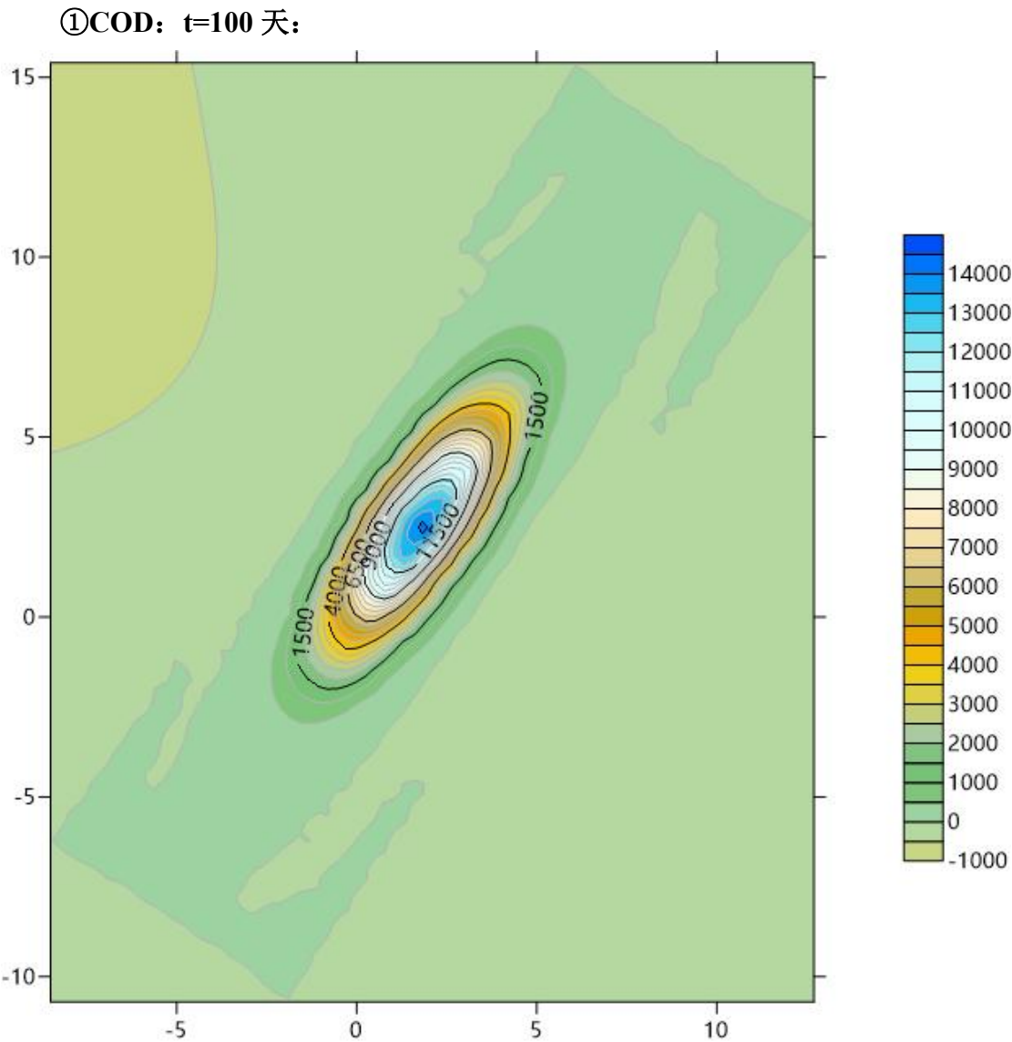
图 6.5-7 假定事故状态下地下水中污染物 COD Mn 100d 的运移情况
