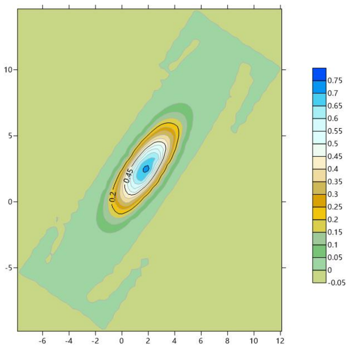
图 6.5-13 假定事故状态下地下水中污染物镉 100d 的运移情况
