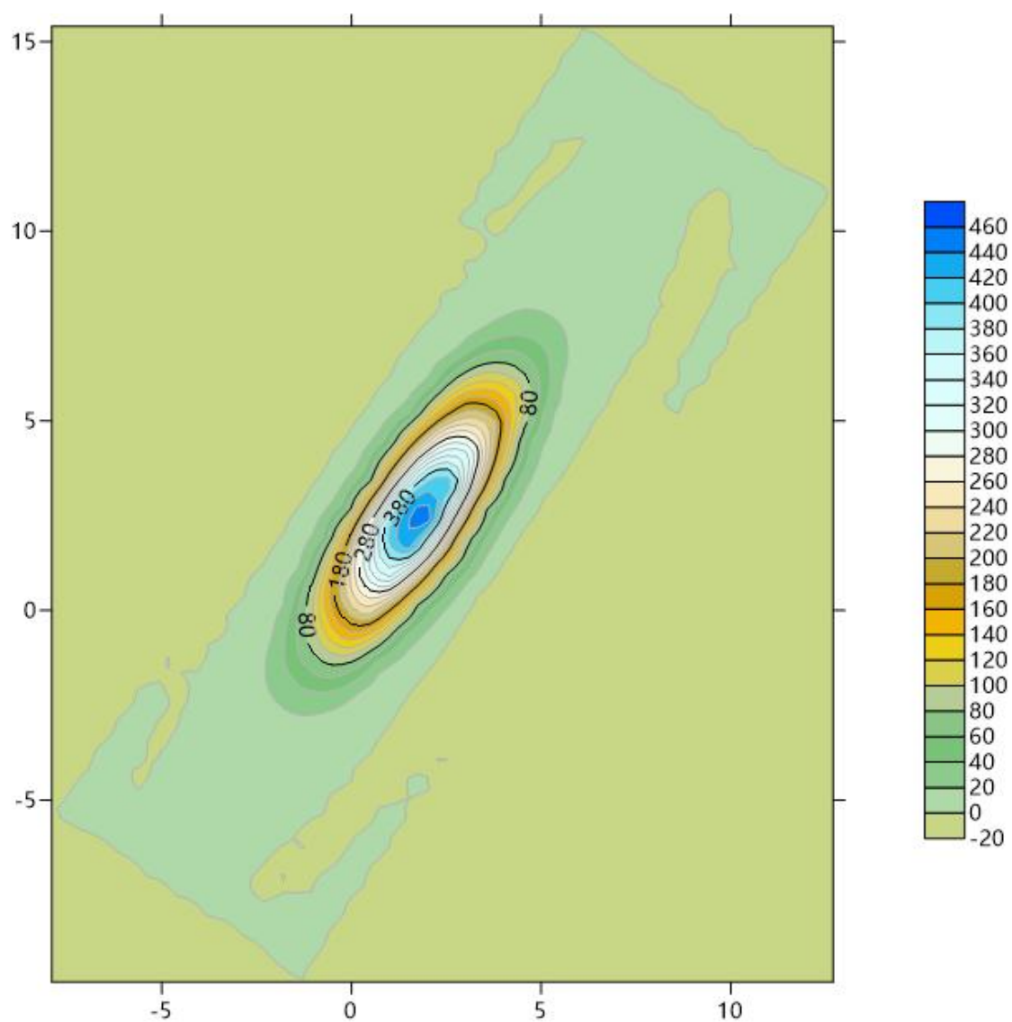
图 6.5-10 假定事故状态下地下水中污染物氨氮 100d 的运移情况
