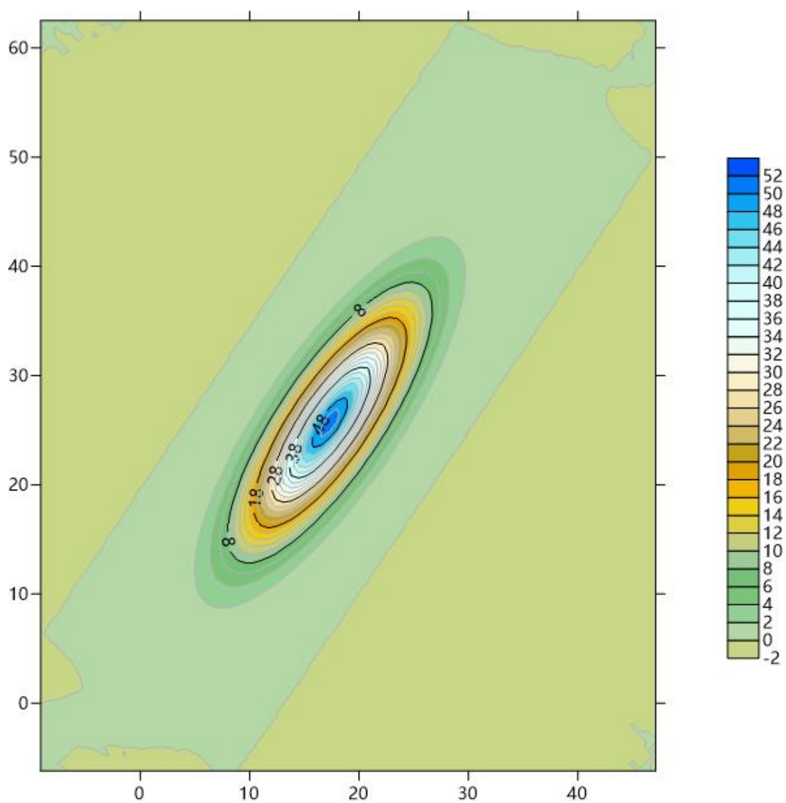
图 6.5-11 假定事故状态下地下水中污染物氨氮 1000d 的运移情况
