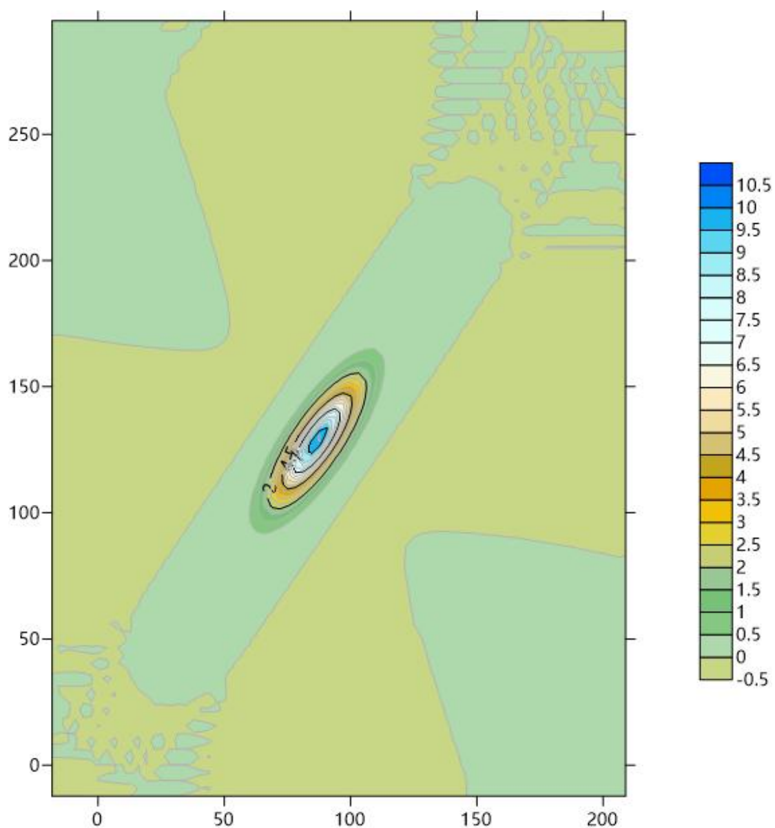
图 6.5-12 假定事故状态下地下水中污染物氨氮 5000d 的运移情况
