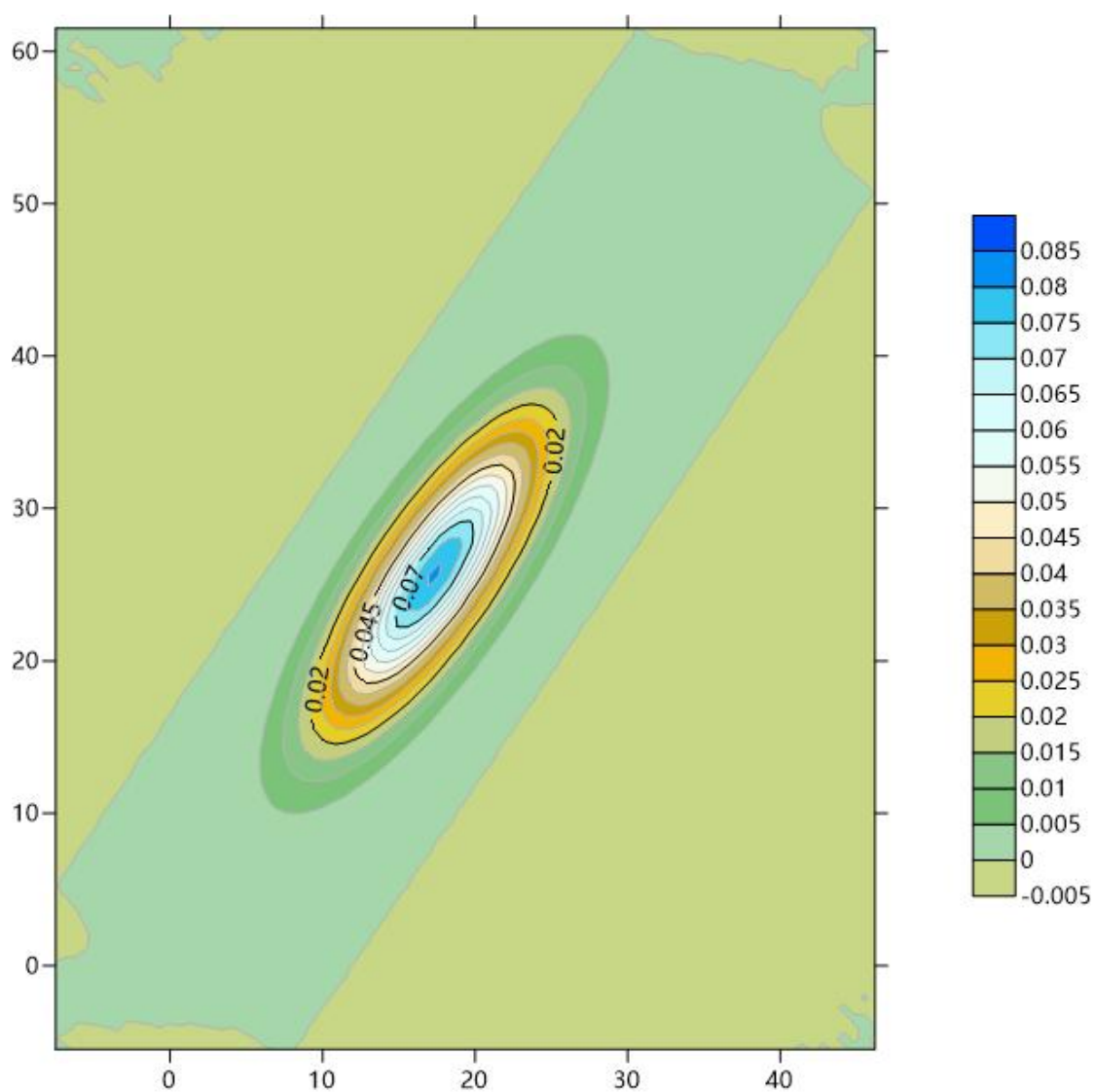
图 6.5-14 假定事故状态下地下水中污染物锑 1000d 的运移情况
