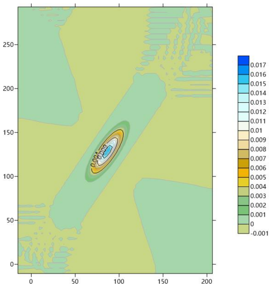
图 6.5-15 假定事故状态下地下水中污染物锑 5000d 的运移情况
