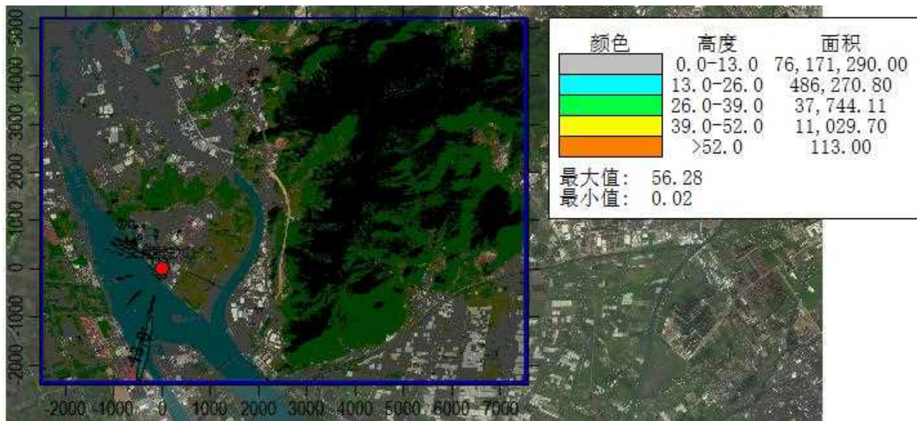
图 5.1-10 TSP 日均浓度贡献值分布图(单位: \mu\text{g}/\text{m}^3 )
