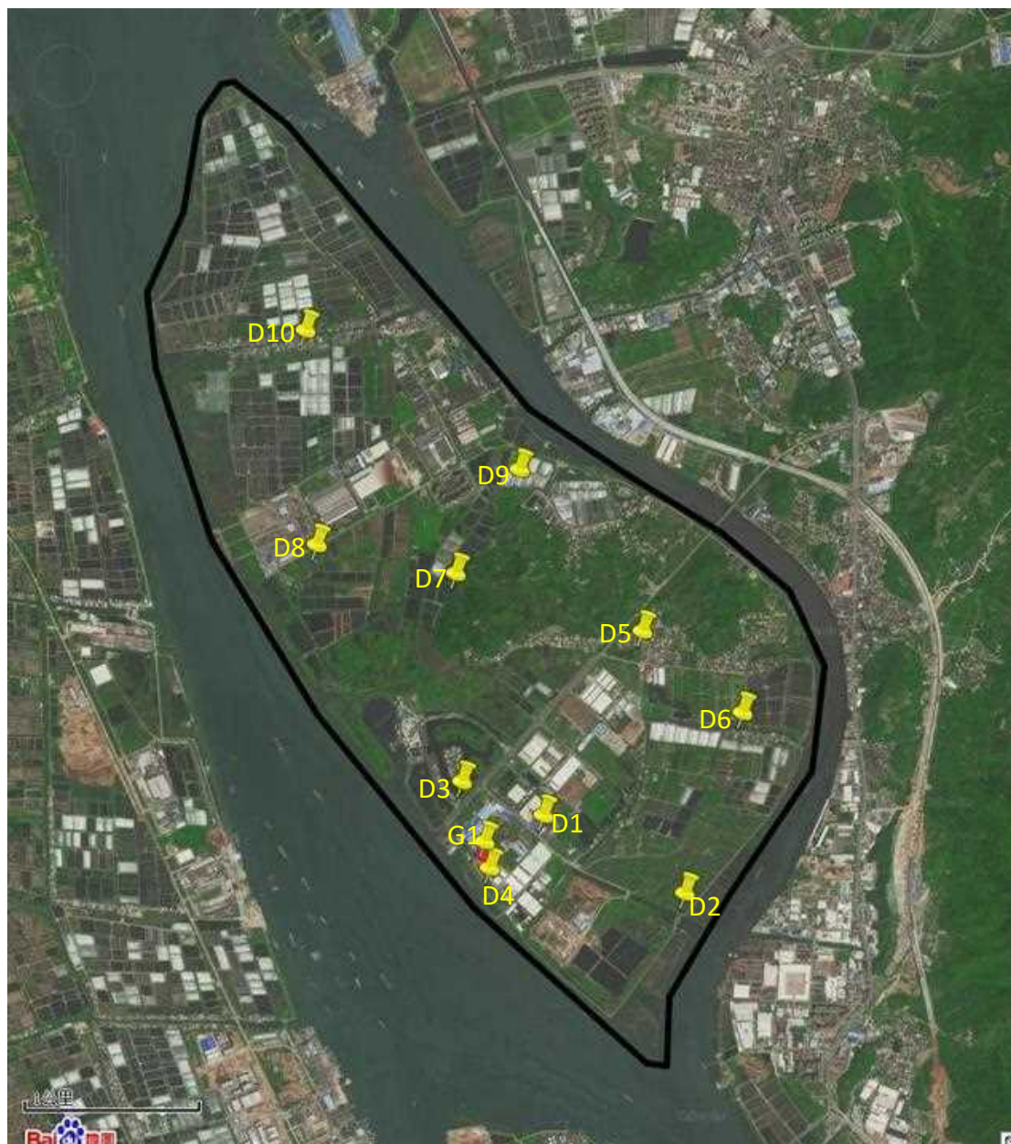
图 4.6-3 地下水监测布点图
