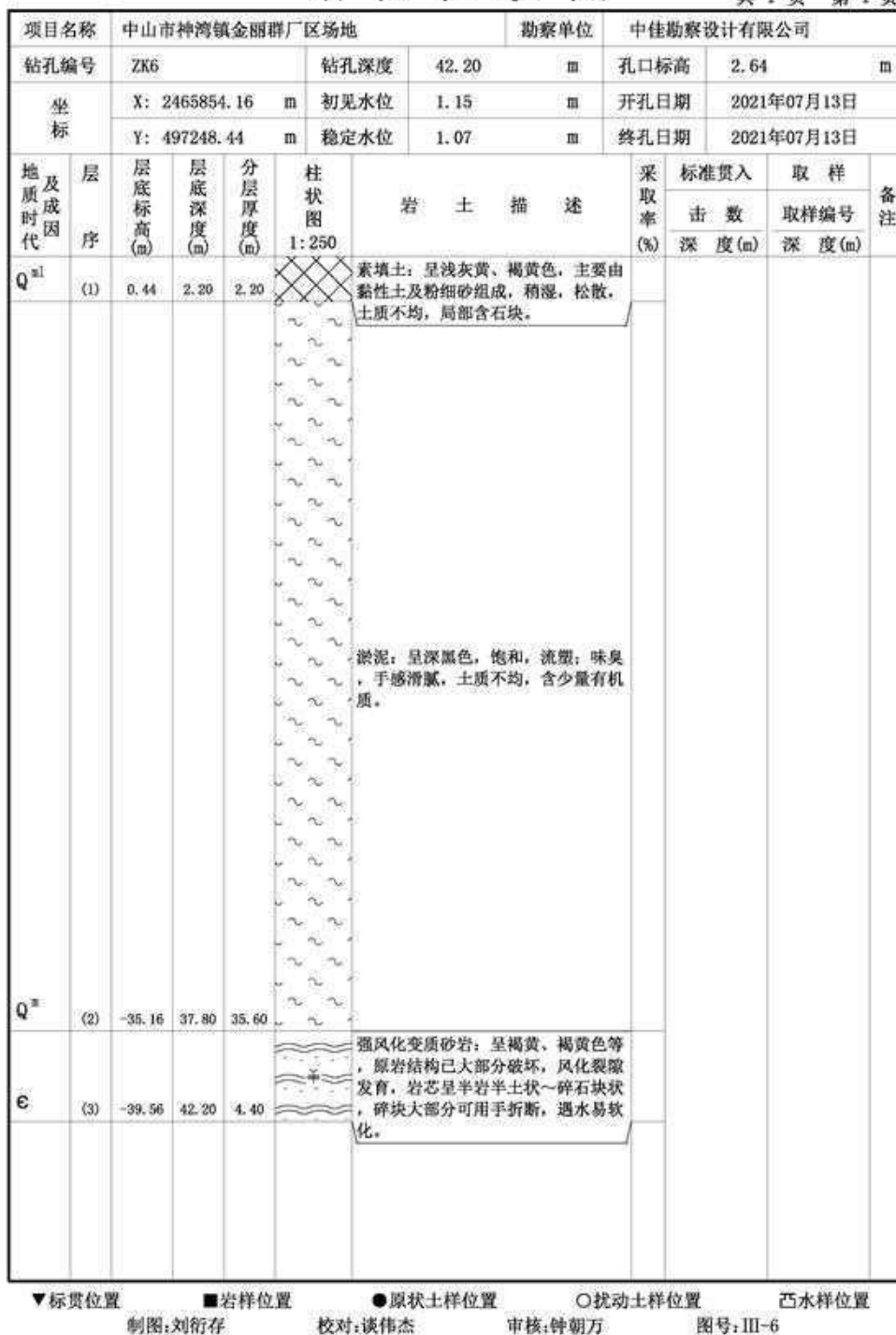
图 5.5-16 项目钻孔柱状图 (ZK6)
