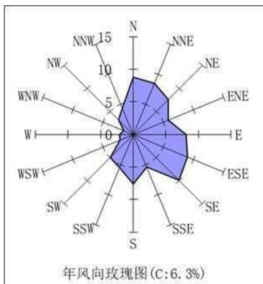
图 5.1-1 中山气象站风向玫瑰图（2003~2022 年）
