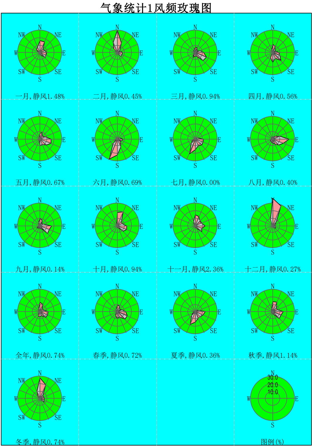
图 5.1-5 中山市 2022 年风频玫瑰图
