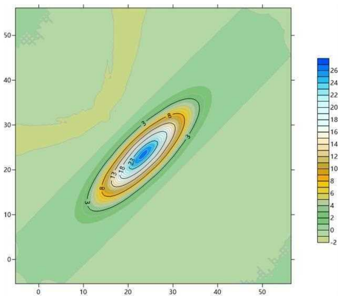
5.5.5.6. 假定事故状态下地下水中污染物 \text{COD}_{\text{Mn}1000\text{d}} 的运移情况
