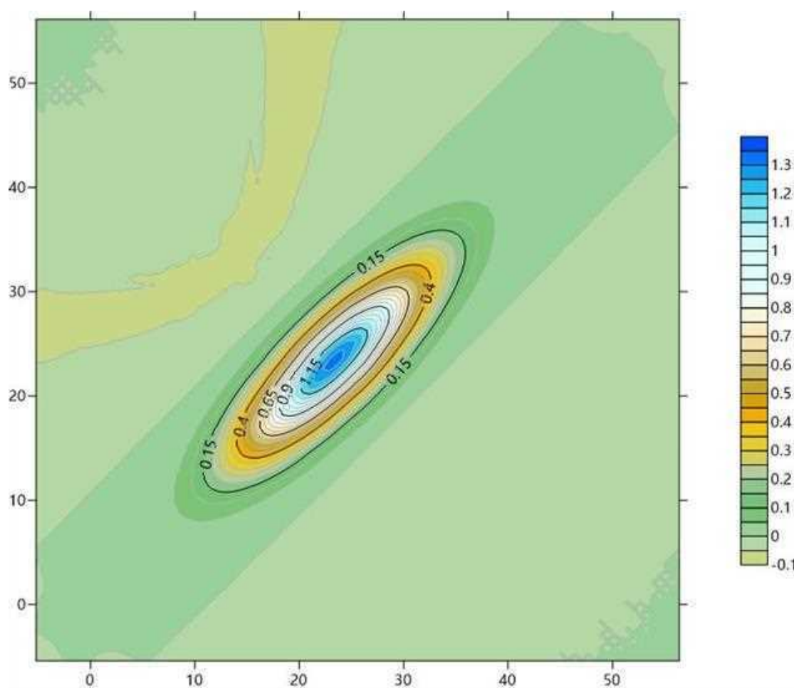
图 5.5-20 假定事故状态下地下水中污染物氨氮 1000d 的运移情况
