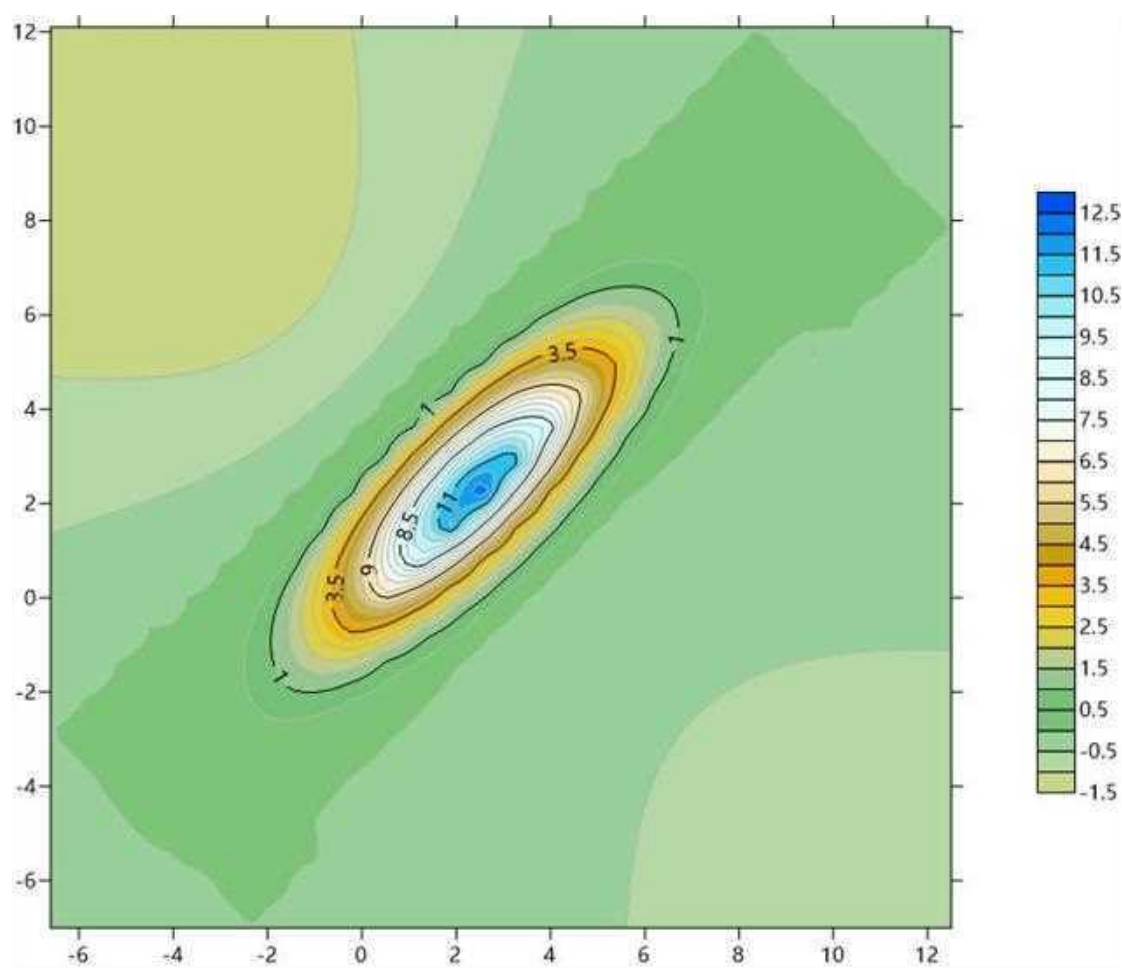
图 5.5-19 假定事故状态下地下水中污染物氨氮 100d 的运移情况
