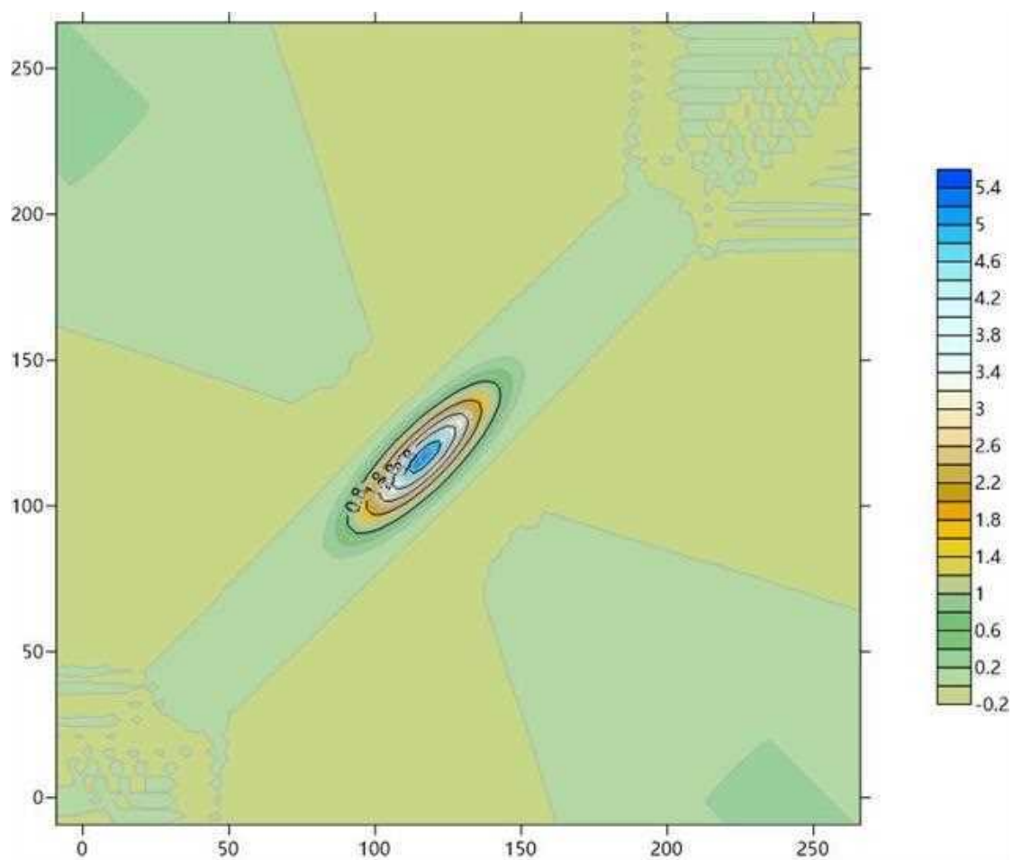
图 5.5-18 假定事故状态下地下水中污染物 COD Mn 5000d 的运移情况
