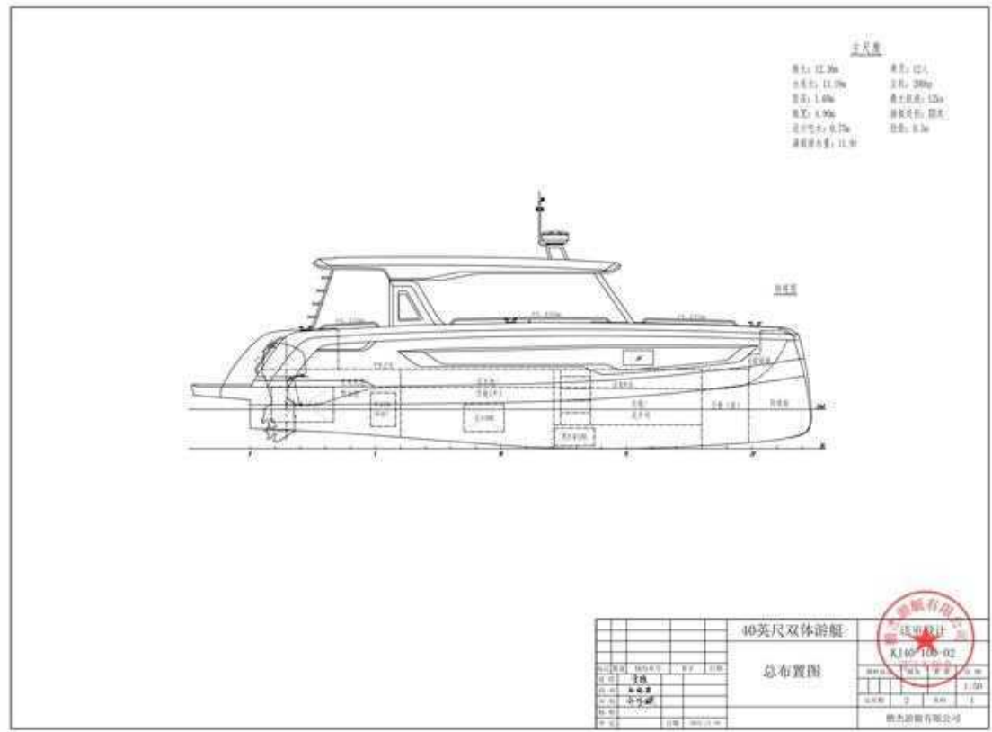
图 3.1-4 项目产品总布置图
