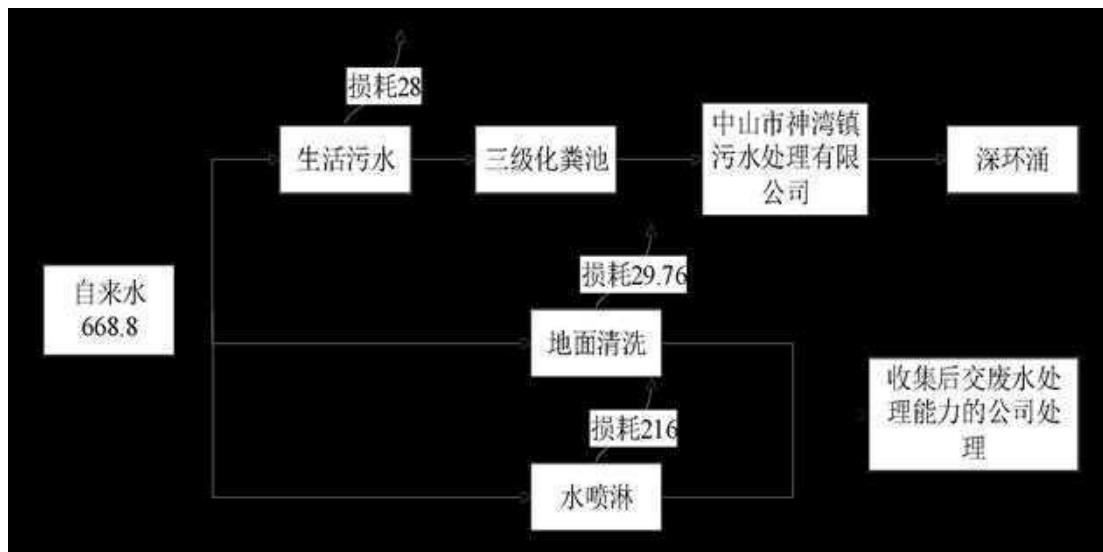
图 3.1-5 项目水平衡图
