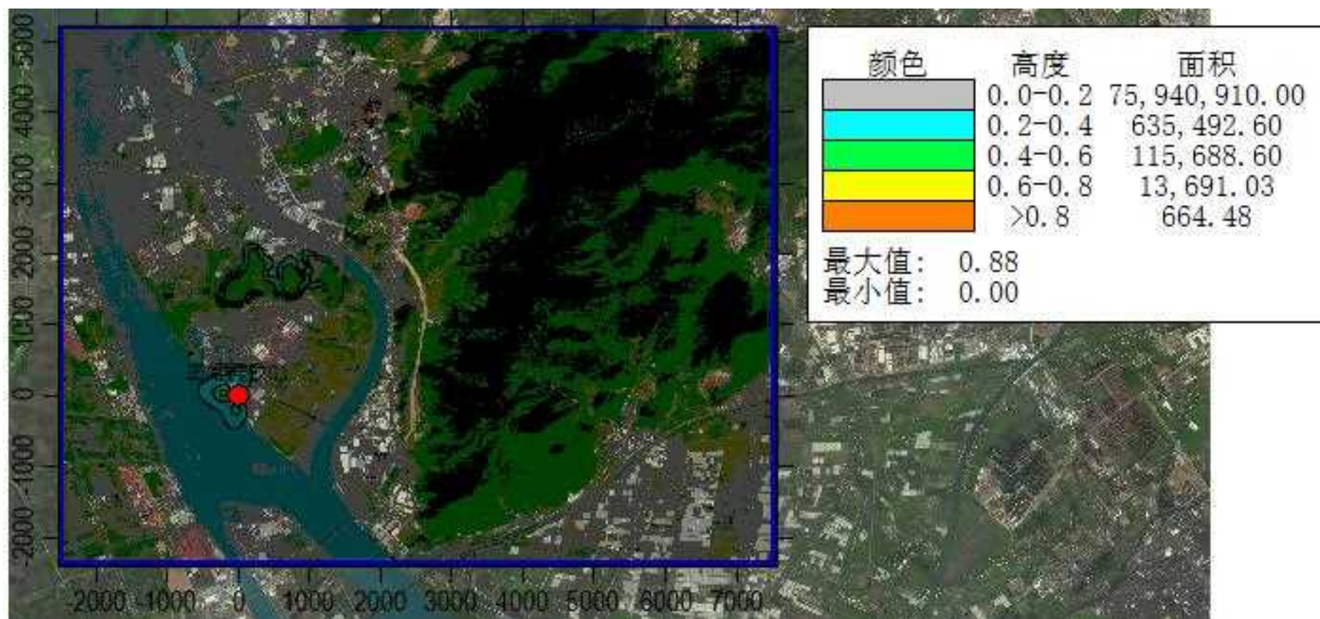
图 5.1-9 PM 10 年平均浓度贡献值分布图(单位: \mu\text{g}/\text{m}^3 )
