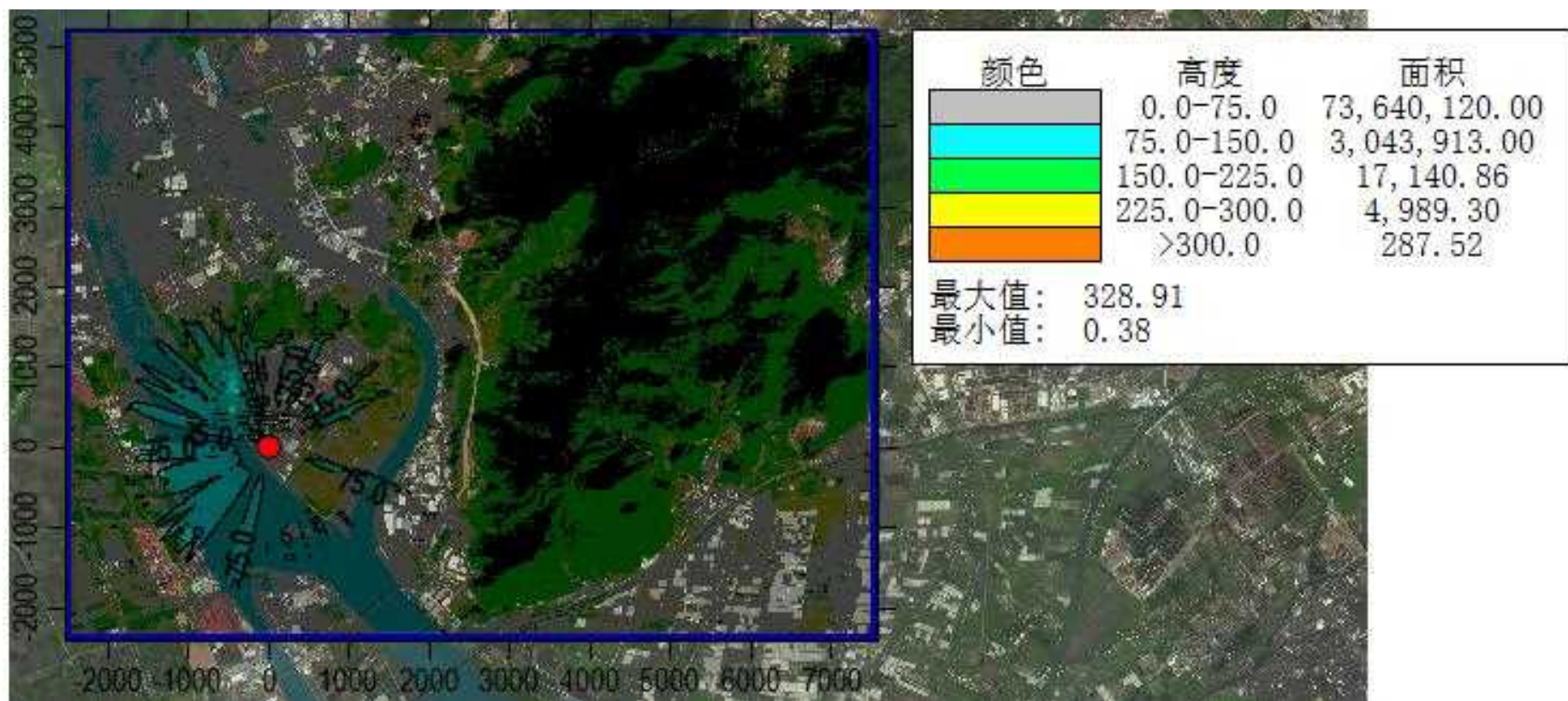
图 5.1-7 非甲烷总烃 1 小时平均浓度贡献值分布图(单位: \mu\text{g}/\text{m}^3 )
