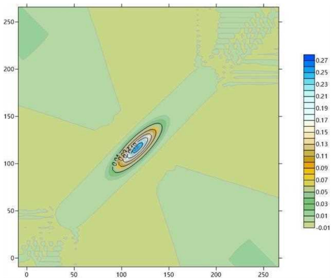
图 5.5-21 假定事故状态下地下水中污染物氨氮 5000d 的运移情况
