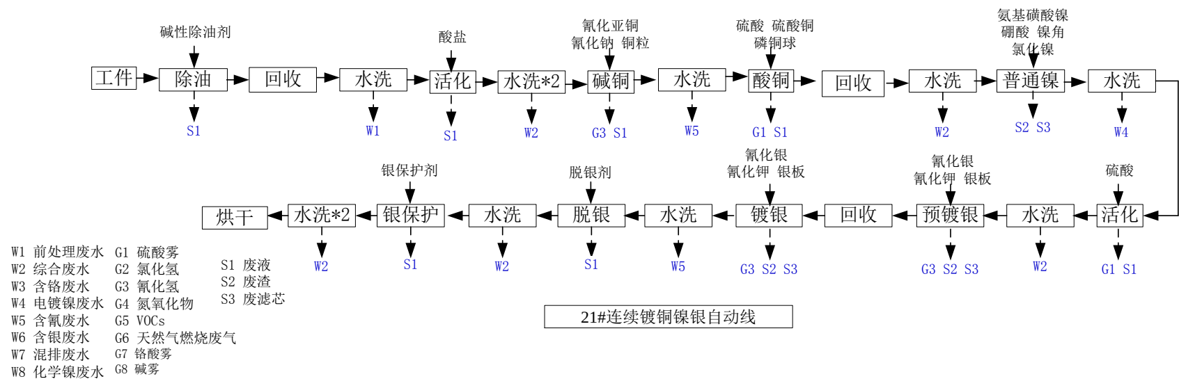
图 4.1- 30 21#端子连续镀铜镍银自动线生产工艺及产污环节
