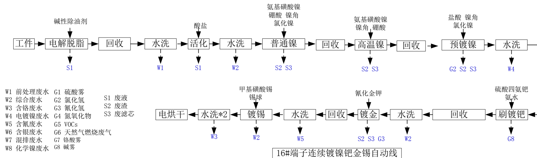
图 4.1-25 16#端子连续镀镍钯金锡自动线生产工艺及产污环节
