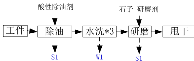
图 4.1- 37 C70 滚筒研磨手动线生产工艺及产污环节
