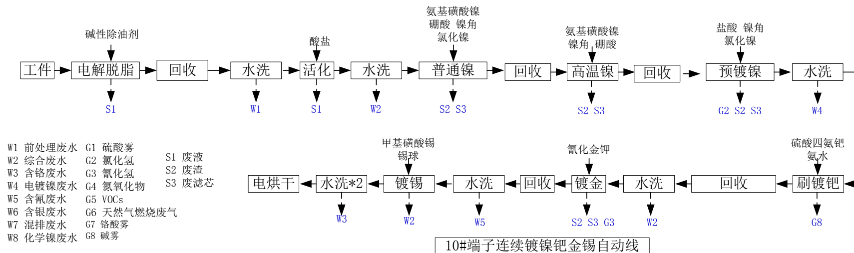
图 4.1-19 10#端子连续镀镍钯金锡自动线生产工艺及产污环节
