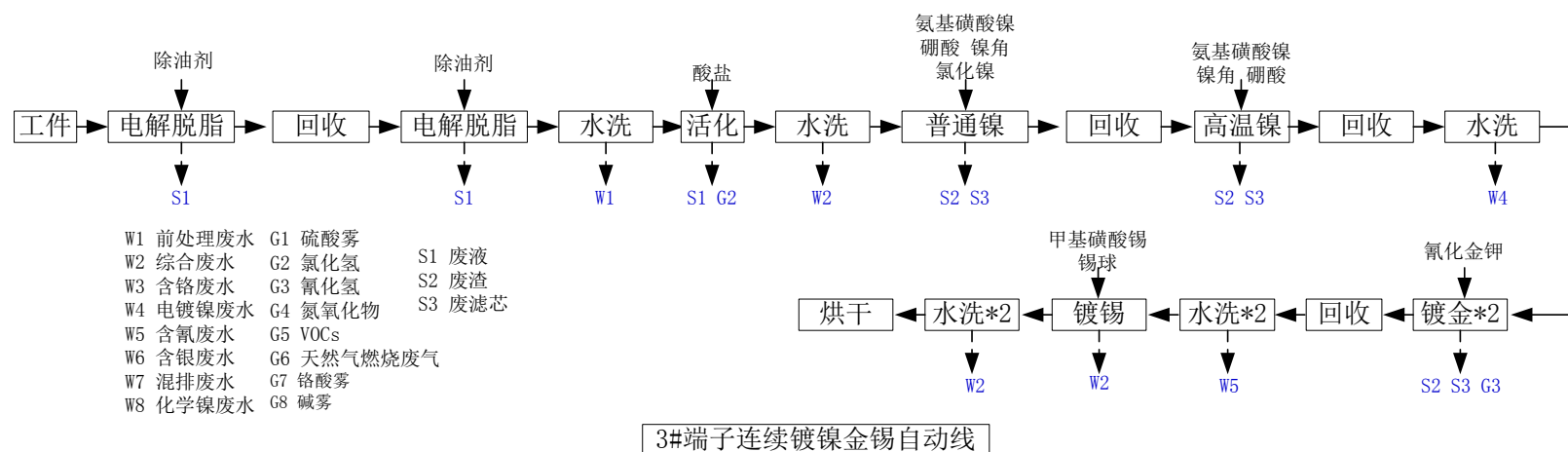
图 4.1-12 3#端子连续镀镍金锡自动线生产工艺及产污环节
