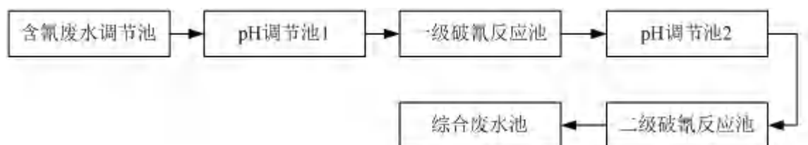
图 7.2-5 含氰废水处理工艺流程图
