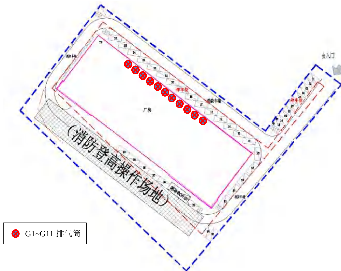
图 4.1-3 建设项目总体平面布置图
