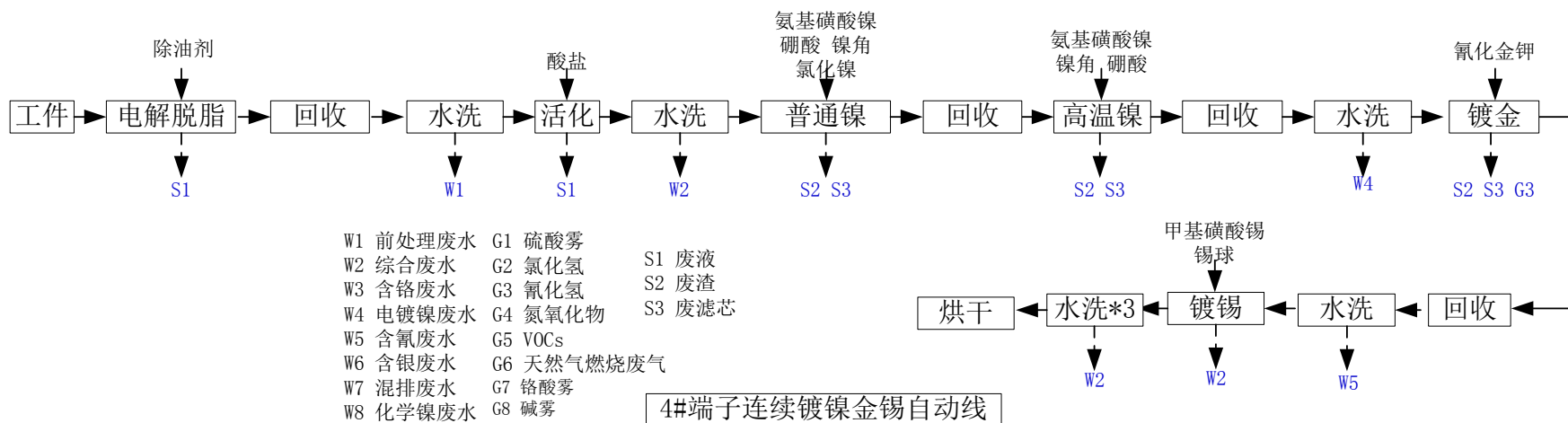
图 4.1-13 4#端子连续镀镍金锡自动线生产工艺及产污环节
