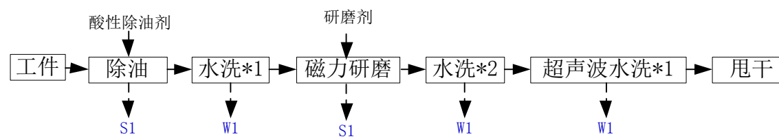
图 4.1- 39 磁力研磨手动线生产工艺及产污环节
