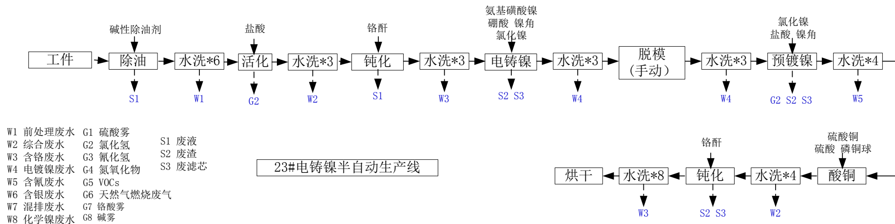
图 4.1-34 23#电铸镍半自动生产线生产工艺及产污环节
