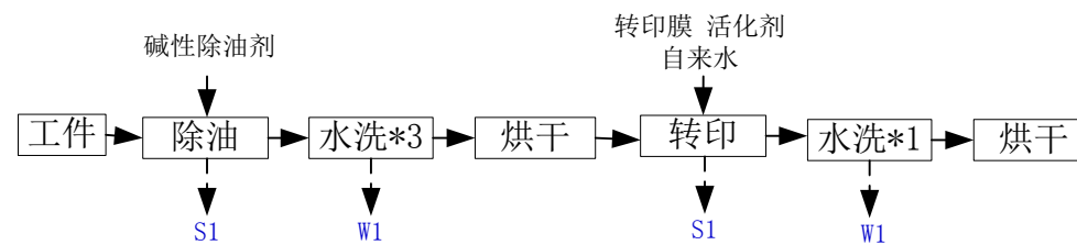
图 4.1-33 水转印线生产工艺及产污环节
