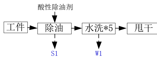
图 4.1-38 散件清洗手动线生产工艺及产污环节
