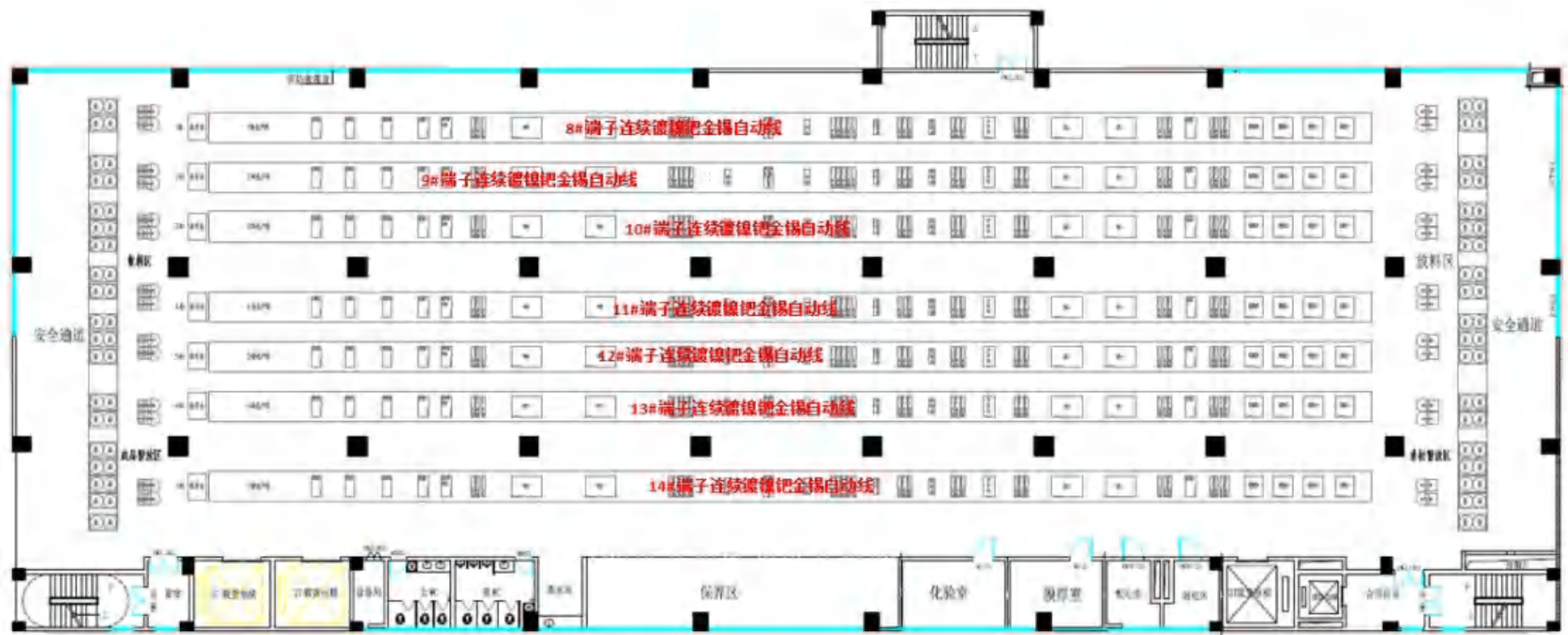
图 4.1-8 生产车间平面布置图（5层）
