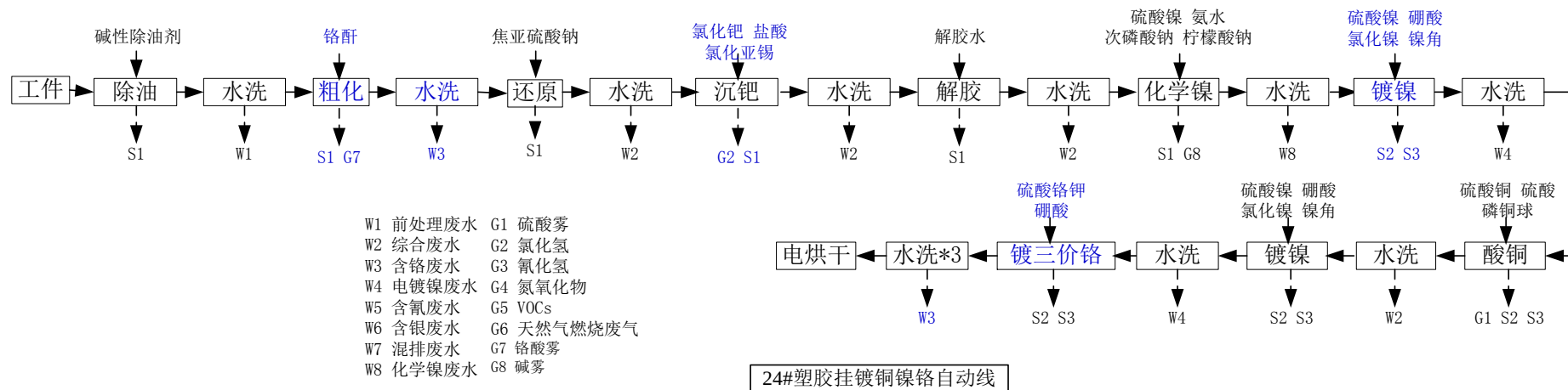
图 4.1- 35 24#塑胶挂镀铜镍铬自动线生产工艺及产污环节
