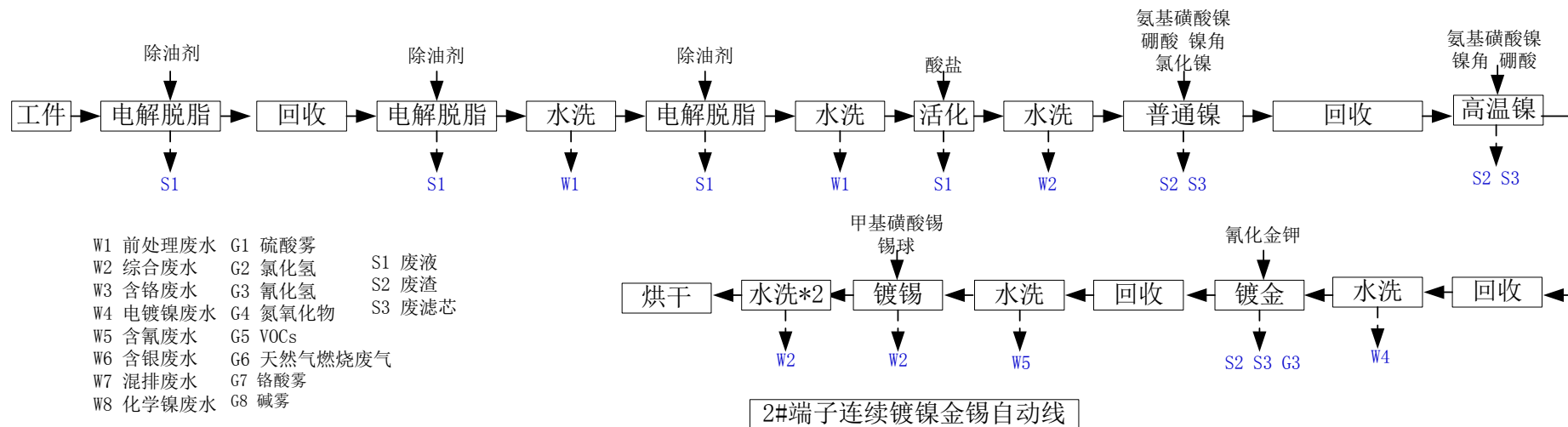
图 4.1-11 2#端子连续镀镍金锡自动线生产工艺及产污环节
