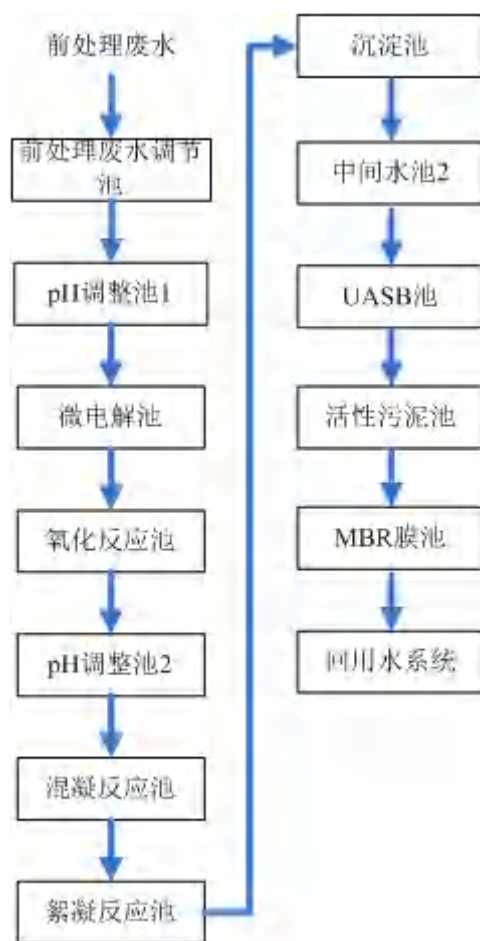
图 7.2-7 前处理废水处理工艺流程图
