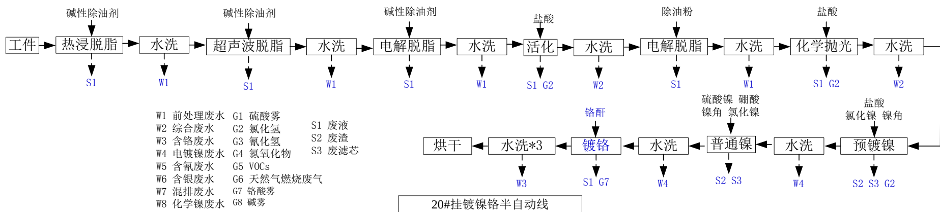
图 4.1-29 20#挂镀镍铬半自动线生产工艺及产污环节
