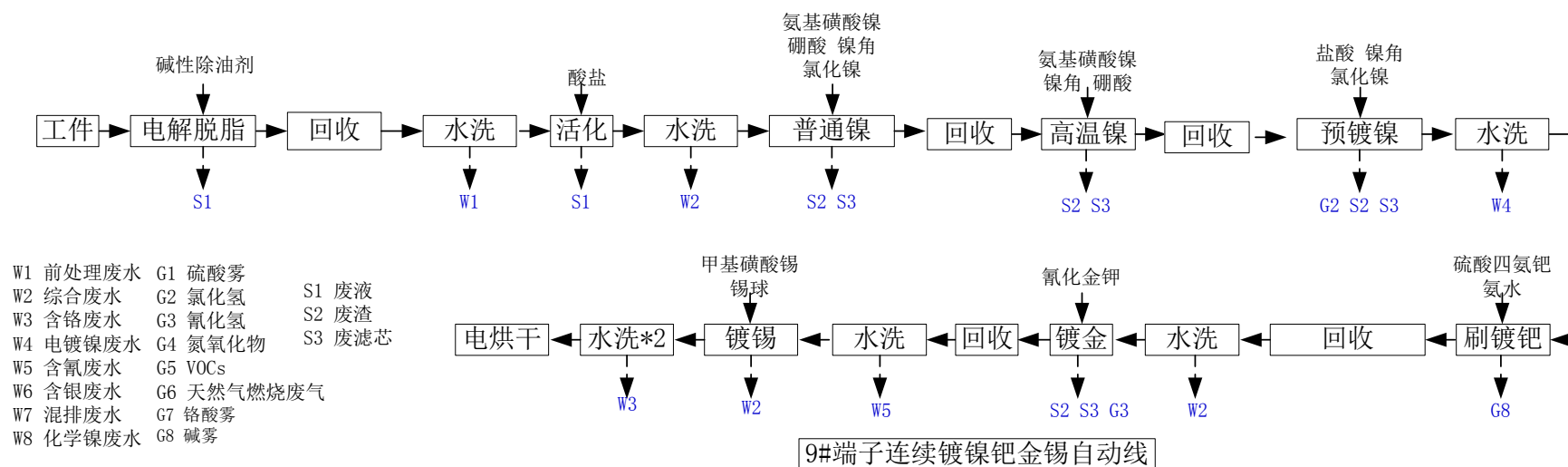
图 4.1-18 9#端子连续镀镍钯金锡自动线生产工艺及产污环节
