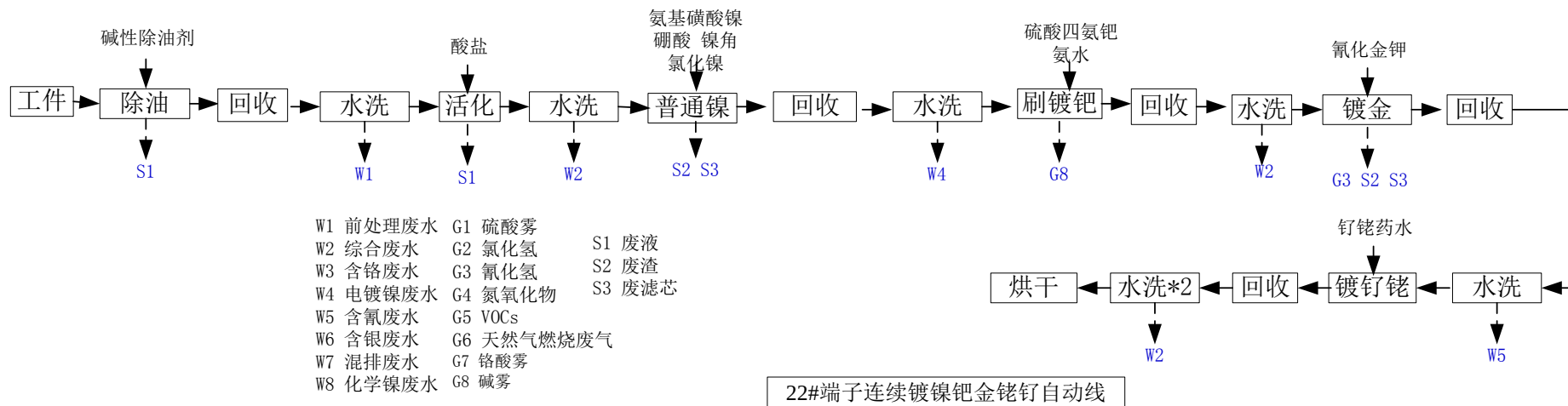
图 4.1- 31 22#端子连续镀镍钯金钌钉自动线生产工艺及产污环节
