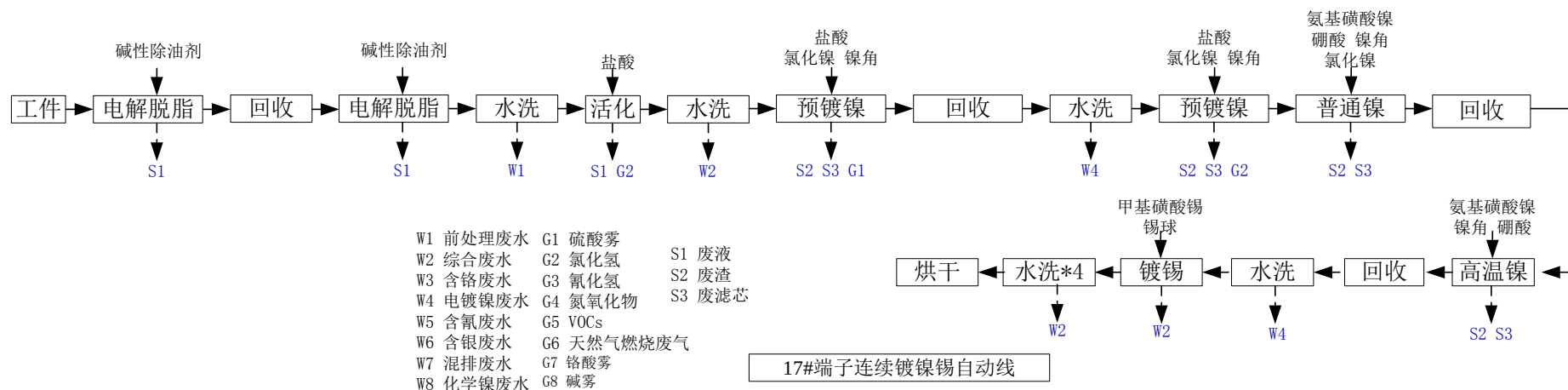
图 4.1-26 17-#端子连续镀镍锡自动线生产工艺及产污环节
