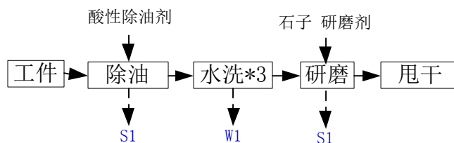
图 4.1-36 TypeC 滚筒研磨手动线生产工艺及产污环节
