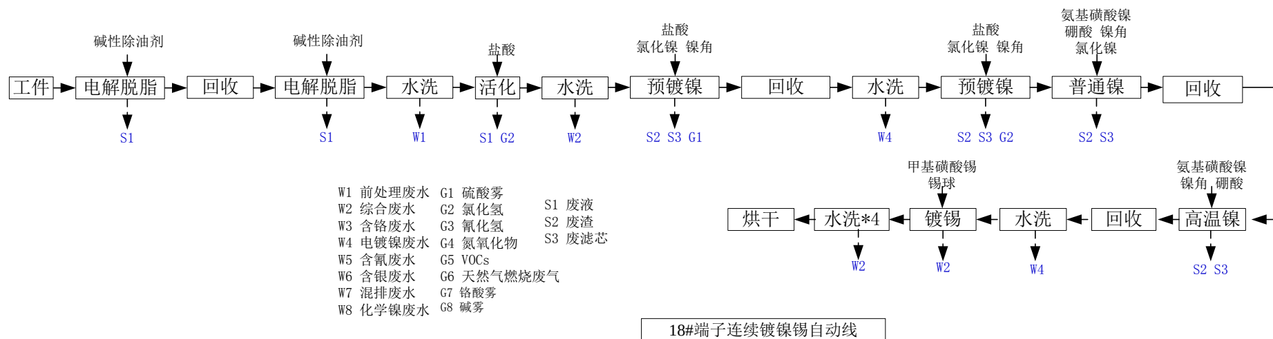
图 4.1-27 18#端子连续镀镍锡自动线生产工艺及产污环节
