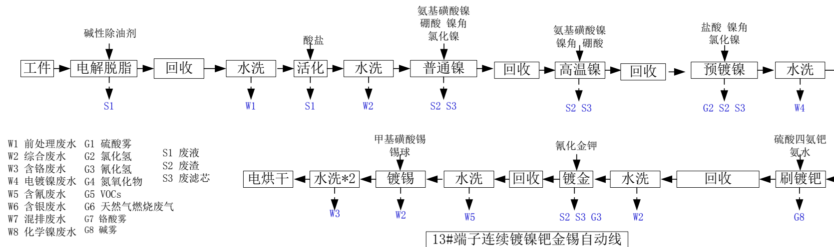
图 4.1-22 13#端子连续镀镍钯金锡自动线生产工艺及产污环节
