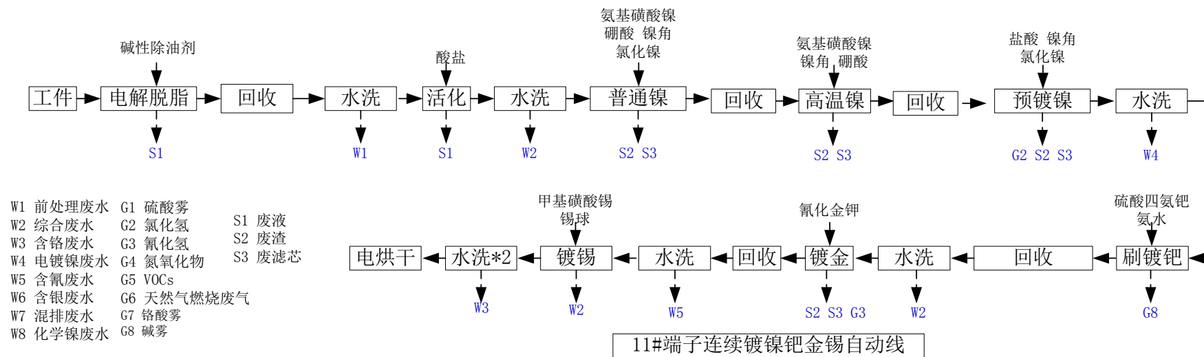
图 4.1-20 11#端子连续镀镍钯金锡自动线生产工艺及产污环节
