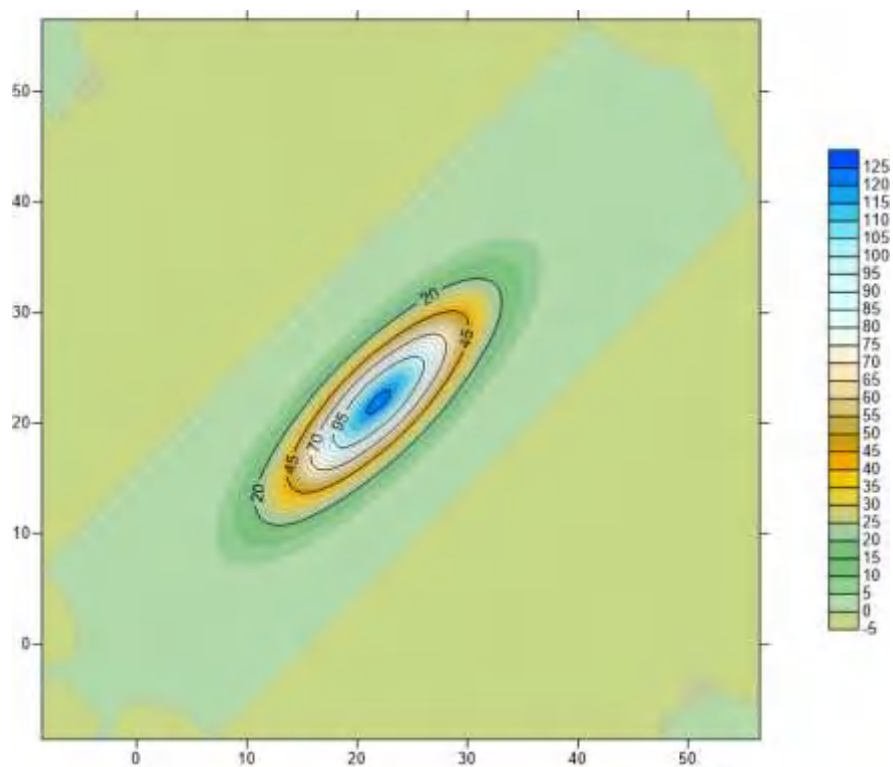
图 6.6-2 假定事故状态下地下水中污染物 \text{COD}_{\text{Mn}} 1000d 的运移情况
