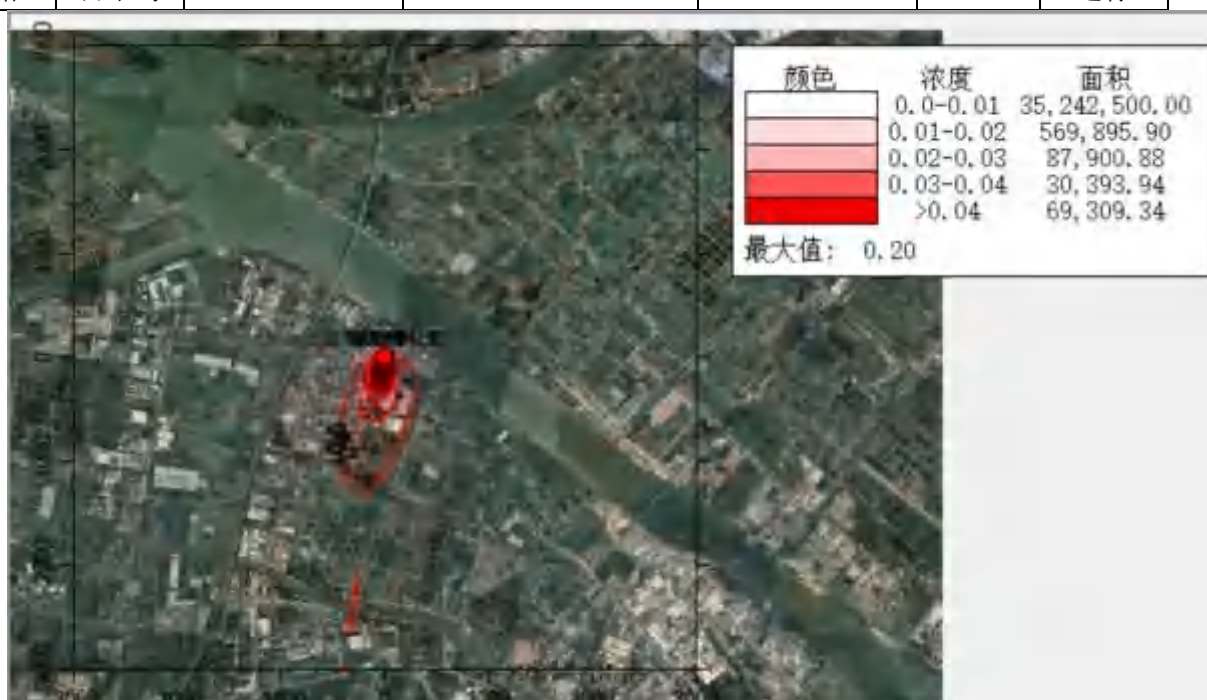
图 6.2-14 氰化氢日平均浓度贡献值分布图(单位: \mu\text{g}/\text{m}^3 )
