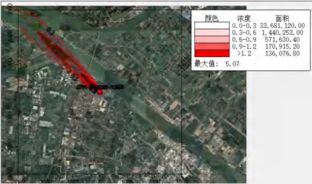
图 6.2-12 硫酸雾 1 小时平均浓度贡献值分布图(单位: \mu\text{g}/\text{m}^3 )
