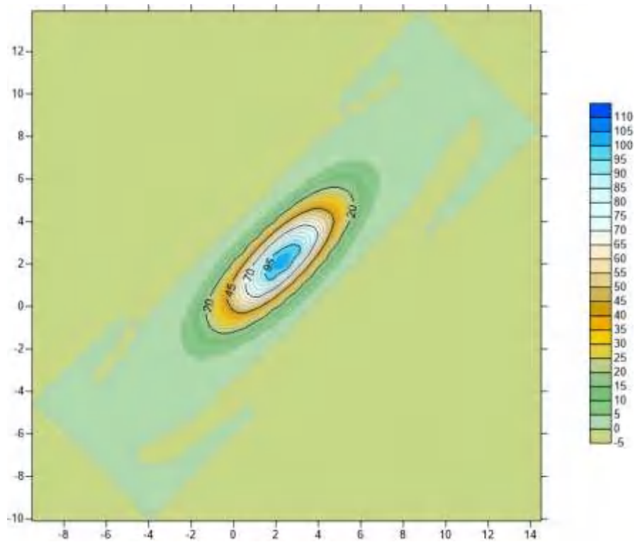
图 6.6-4 假定事故状态下地下水中污染物氰化物 100d 的运移情况
