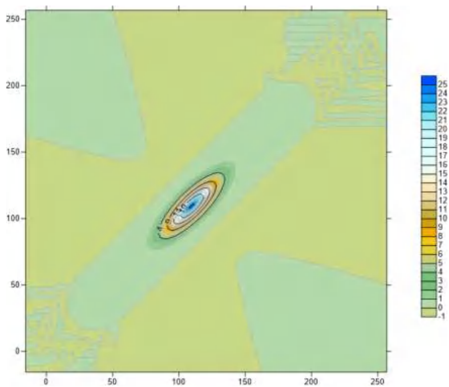
图 6.6-3 假定事故状态下地下水中污染物 \text{COD}_{\text{Mn}} 5000d 的运移情况
