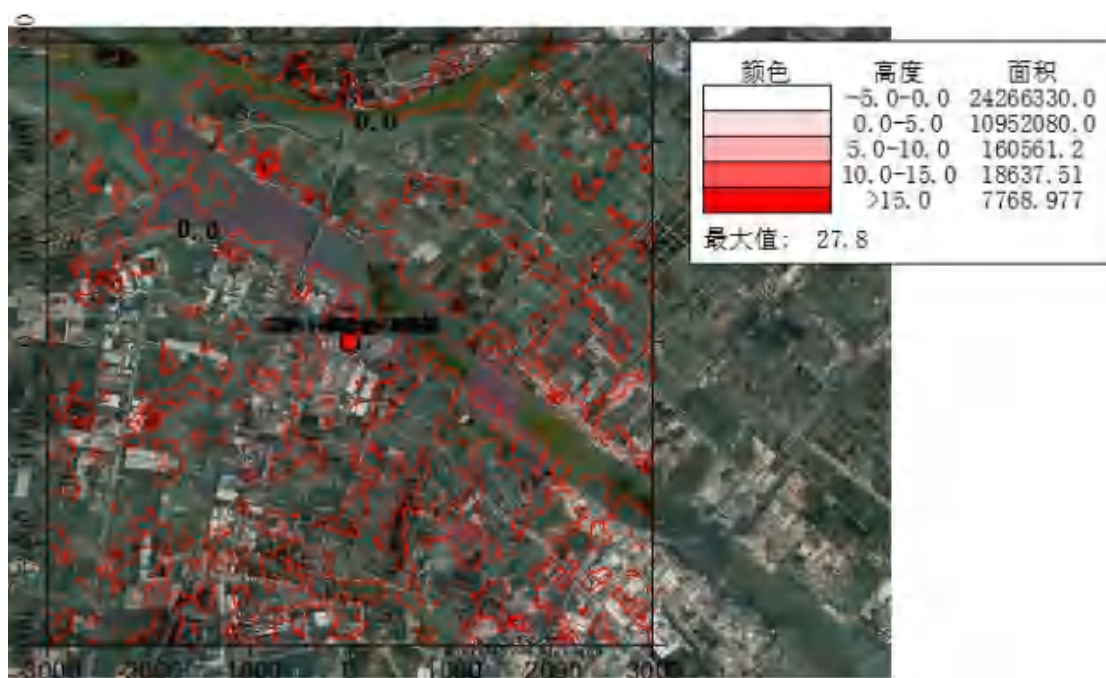
图 6.2-8 项目评价范围内的地形示意图
