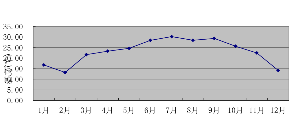
图 6.2-4 中山市 2022 年平均温度的月变化图
