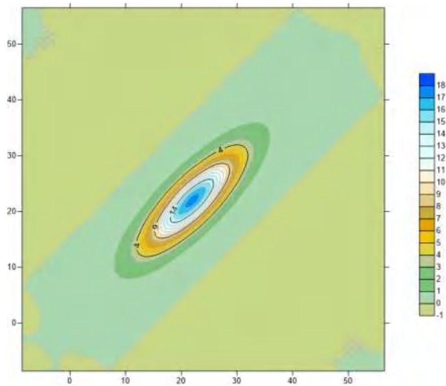
图 6.6-8 假定事故状态下地下水中污染物镍 1000d 的运移情况
