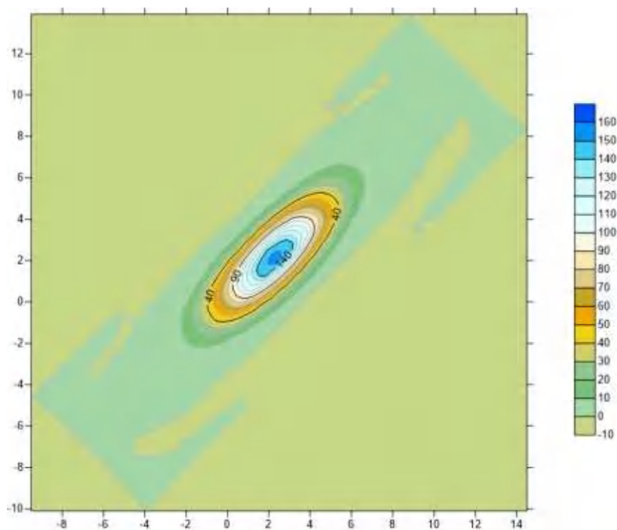
图 6.6-7 假定事故状态下地下水中污染物镍 100d 的运移情况
