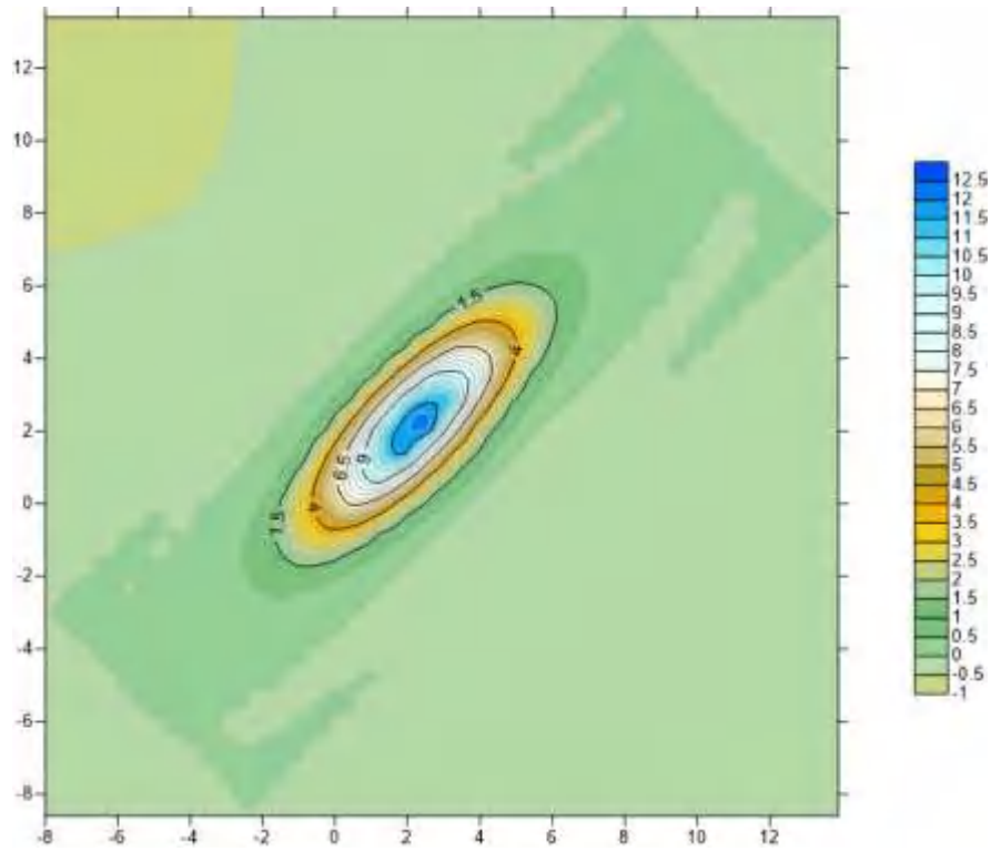
图 6.6-10 假定事故状态下地下水中污染物六价铬 100d 的运移情况
