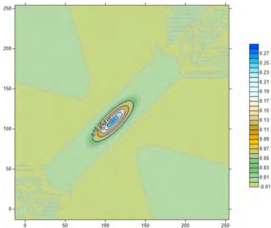
图 6.6-12 假定事故状态下地下水中污染物六价铬 5000d 的运移情况
