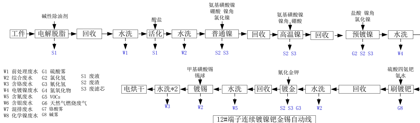
图 4.1-21 12#端子连续镀镍钯金锡自动线生产工艺及产污环节
