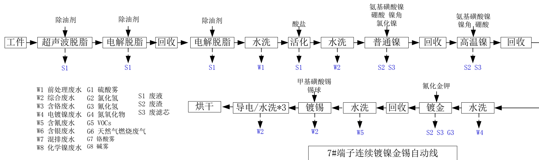
图 4.1-16 7#端子连续镀镍金锡自动线生产工艺及产污环节
