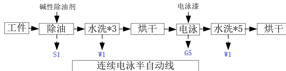
图 4.1-32 连续电泳半自动线生产工艺及产污环节
