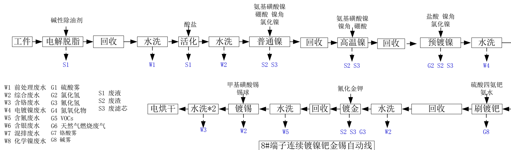
图 4.1-17 8#端子连续镀镍钯金锡自动线生产工艺及产污环节
