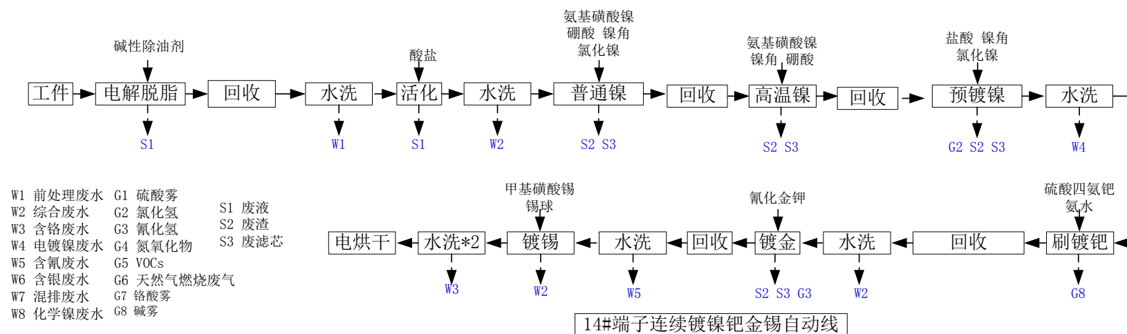
图 4.1 -23 14#端子连续镀镍钯金锡自动线生产工艺及产污环节
