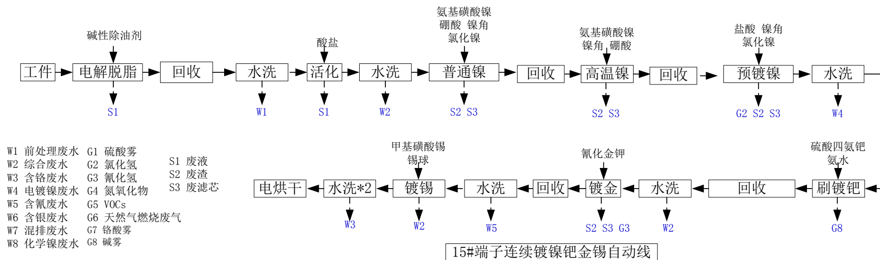
图 4.1-24 15#端子连续镀镍钯金锡自动线生产工艺及产污环节
