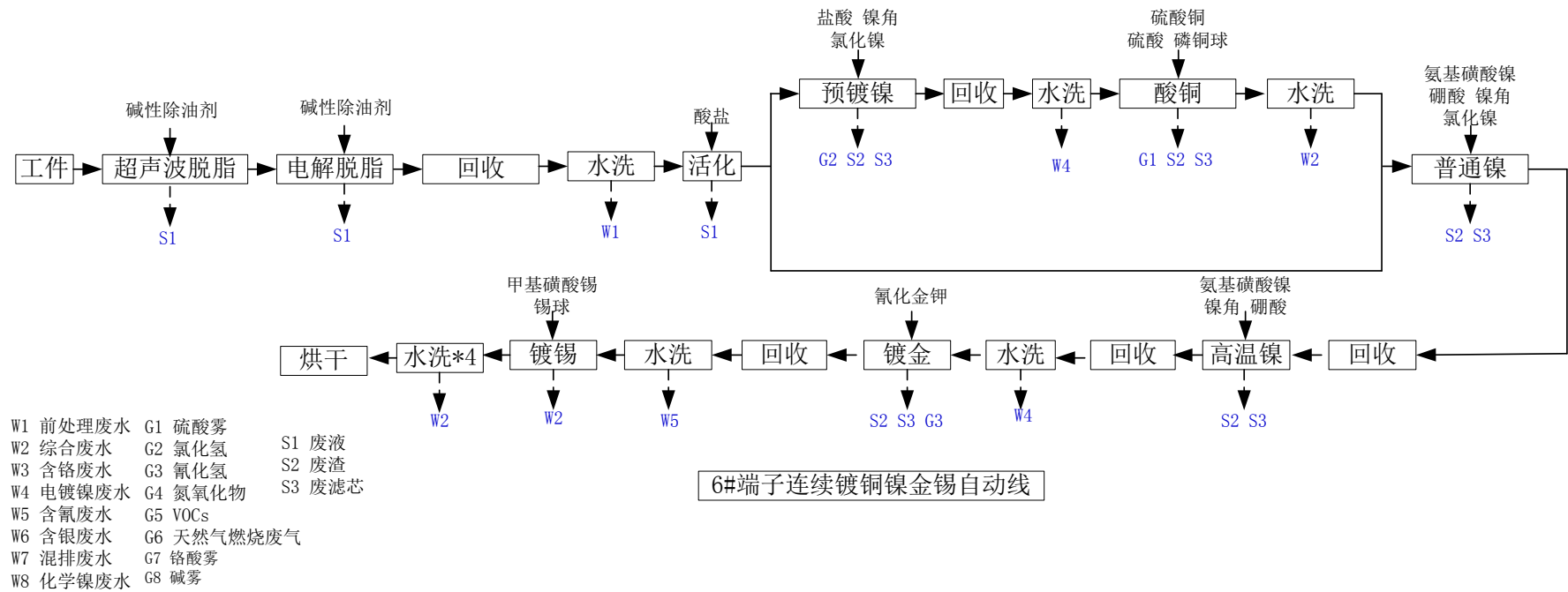
图 4.1-15 6#端子连续镀铜镍金锡自动线生产工艺及产污环节
