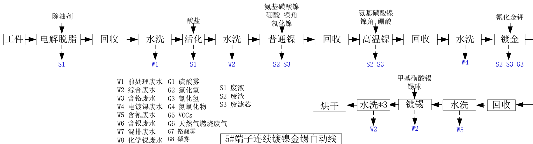
图 4.1-14 5#端子连续镀镍金锡自动线生产工艺及产污环节
