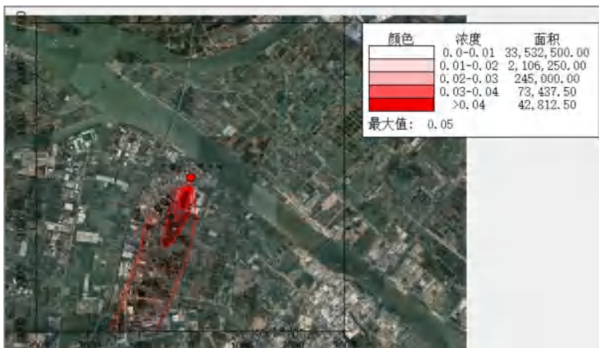
图 6.2-22 SO2 日均浓度贡献值分布图(单位: \mu\text{g}/\text{m}^3 )
