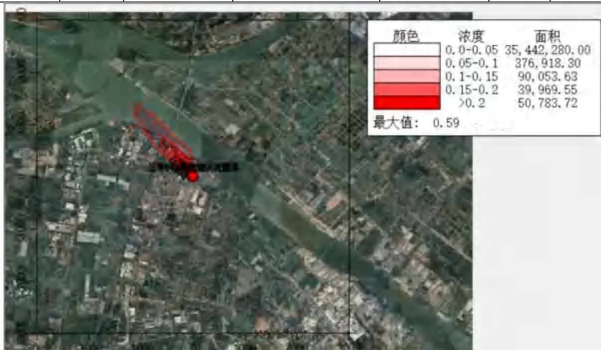
图 6.2-13 硫酸雾日平均浓度贡献值分布图(单位: \mu\text{g}/\text{m}^3 )
