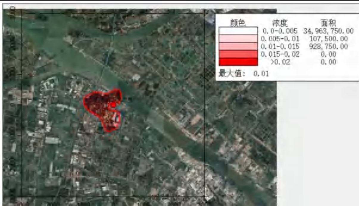
图 6.2-24 NO 2 年平均浓度贡献值分布图(单位: ug/m 3 )
