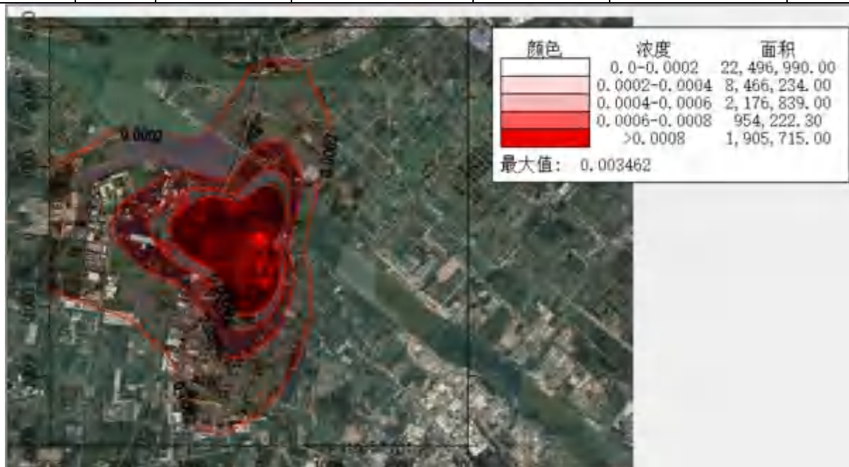
图 6.2-19 PM 10 年平均浓度贡献值分布图(单位: \mu\text{g}/\text{m}^3 )
