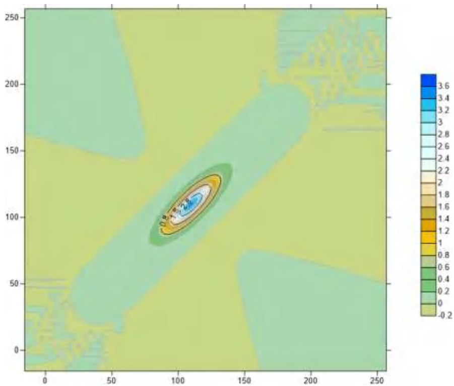
图 6.6-9 假定事故状态下地下水中污染物镍 5000d 的运移情况
