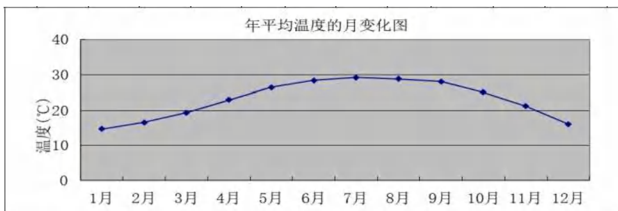
图 6.2-1 中山市 2003~2022 年逐月平均温度变化曲线
