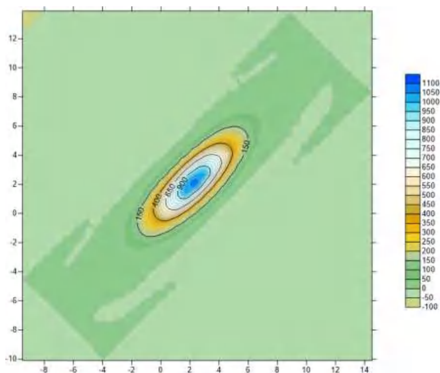
图 6.6-1 假定事故状态下地下水中污染物 \text{COD}_{\text{Mn}100\text{d}} 的运移情况
