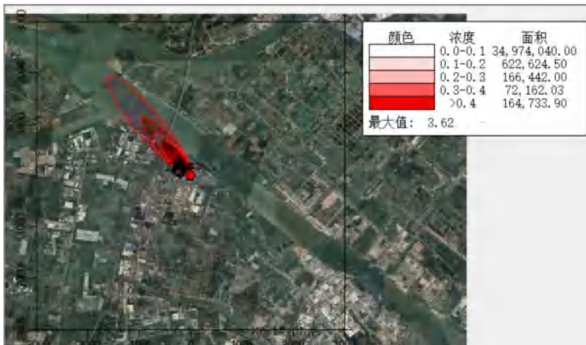
图 6.2-17 TVOC8 小时平均浓度贡献值分布图(单位: \mu\text{g}/\text{m}^3 )
