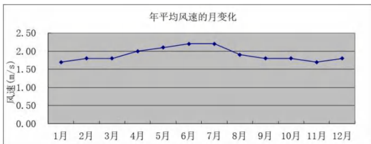
图 6.2-2 中山市 2003~2022 年逐月平均风速变化曲线
