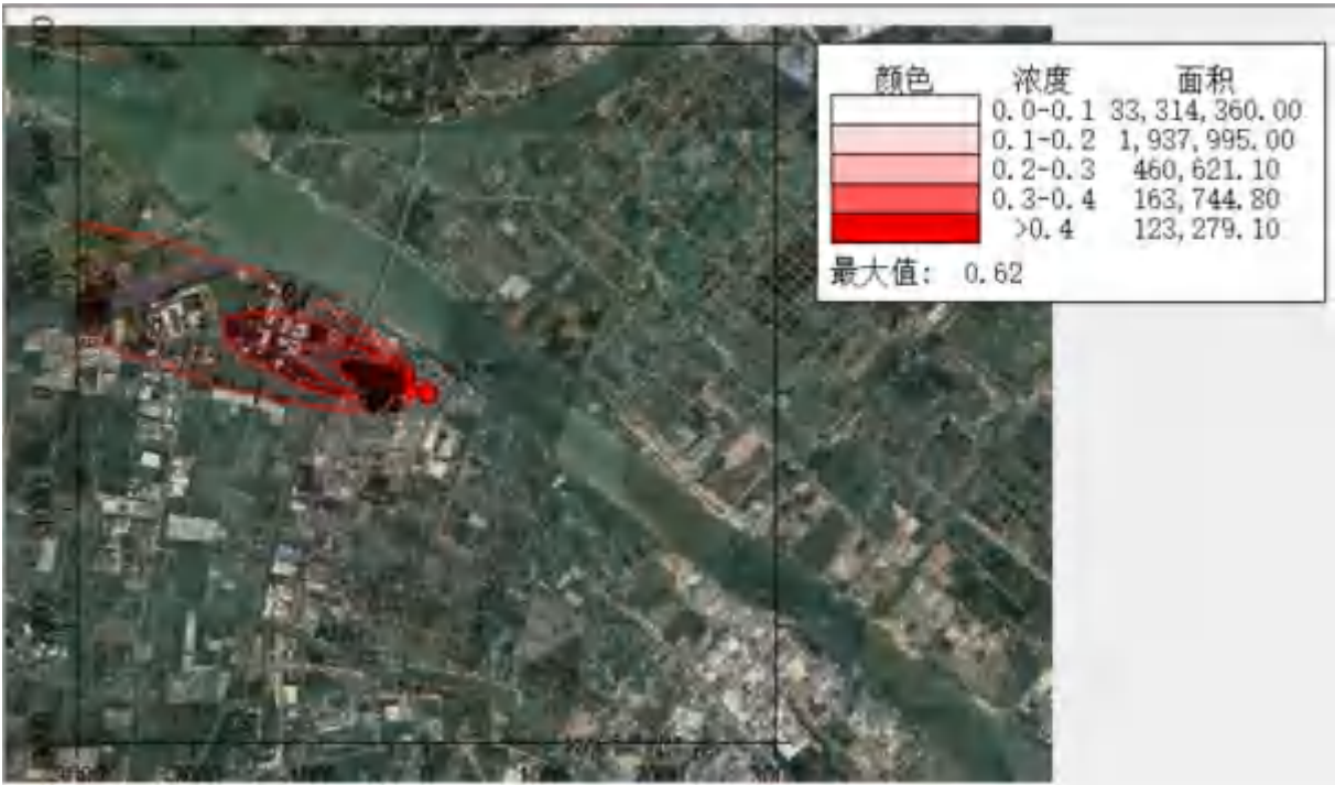
图 6.2-21 NO2 小时浓度贡献值分布图(单位：ug/m³)
