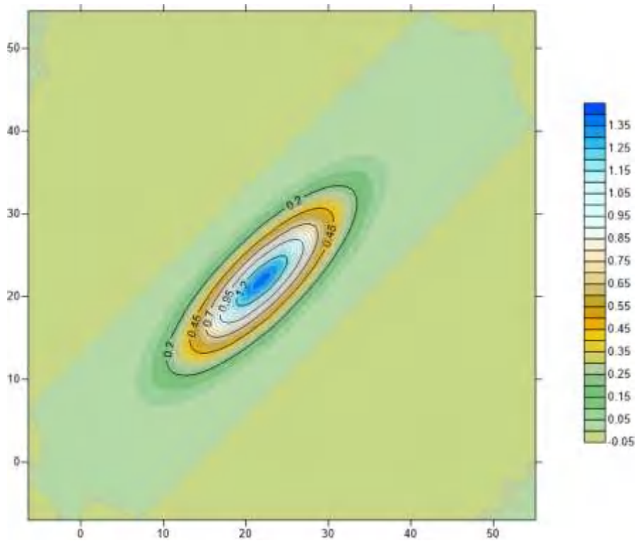
图 6.6-11 假定事故状态下地下水中污染物六价铬 1000d 的运移情况
