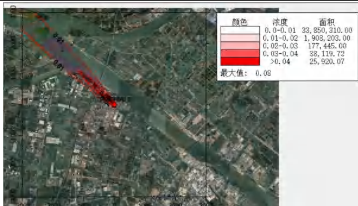
图 6.2-15 铬酸雾日平均浓度贡献值分布图(单位: \mu\text{g}/\text{m}^3 )
