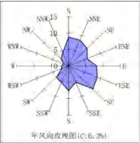
图 6.2-3 中山气象站风向玫瑰图（统计年限：2003~2022 年）
