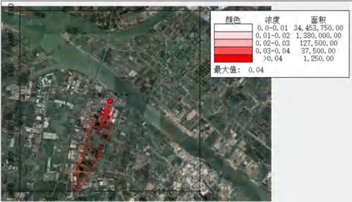
图 6.2-18 PM10 日均浓度贡献值分布图(单位: \mu\text{g}/\text{m}^3 )
