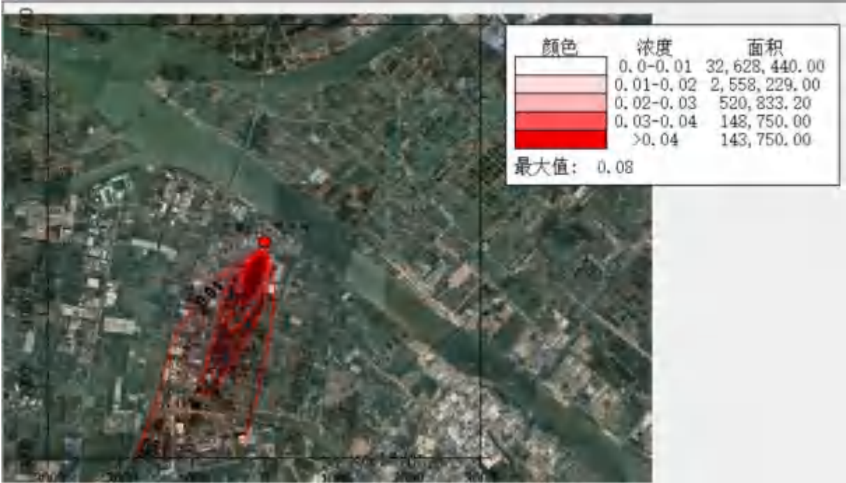
图 6.2-22 NO2 日均浓度贡献值分布图(单位: ug/m³)
