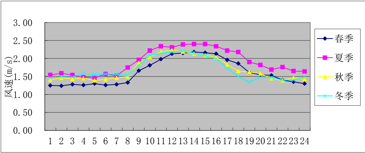
图 6.2-6 中山市 2022 年季小时平均风速的日变化图
