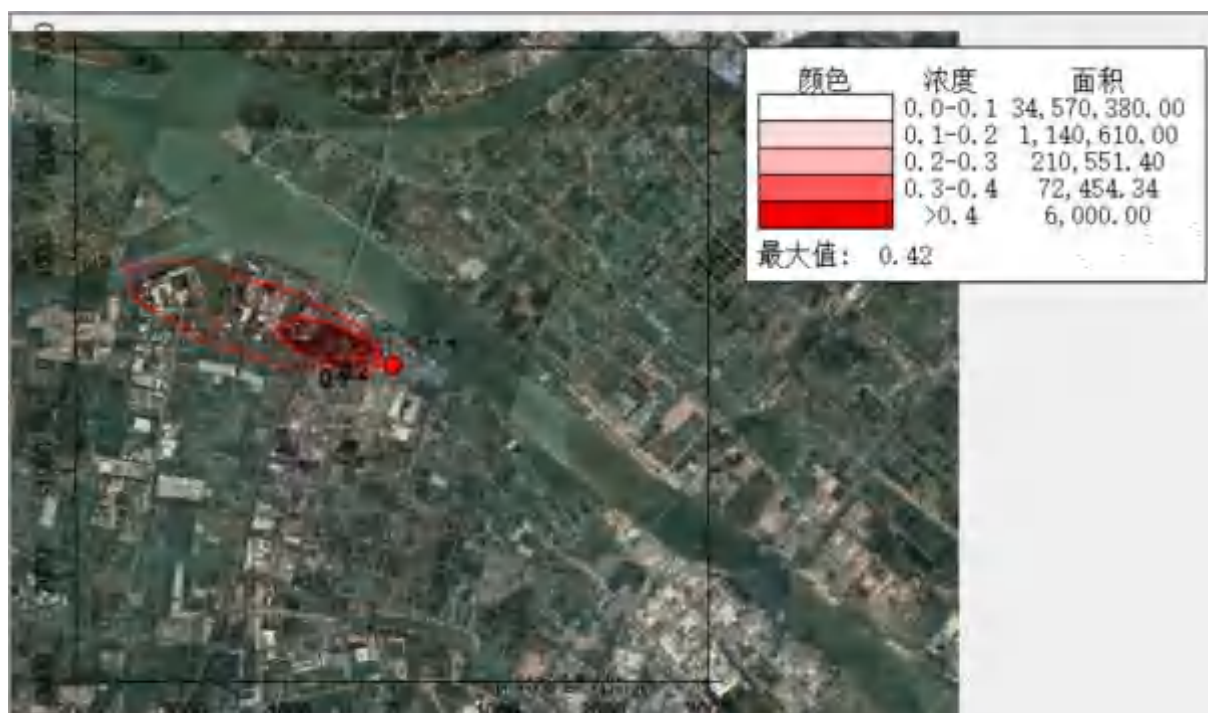
图 6.2-21 SO 2 小时浓度贡献值分布图(单位: \mu\text{g}/\text{m}^3 )
