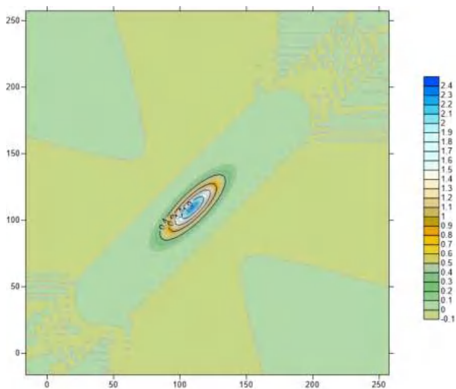
图 6.6-6 假定事故状态下地下水中污染物氰化物 5000d 的运移情况
