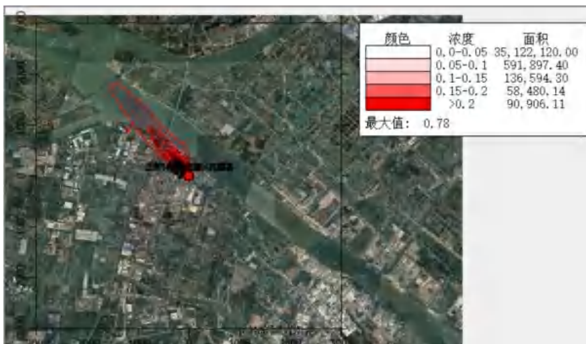
图 6.2-11 氯化氢日平均浓度贡献值分布图(单位: \mu\text{g}/\text{m}^3 )
