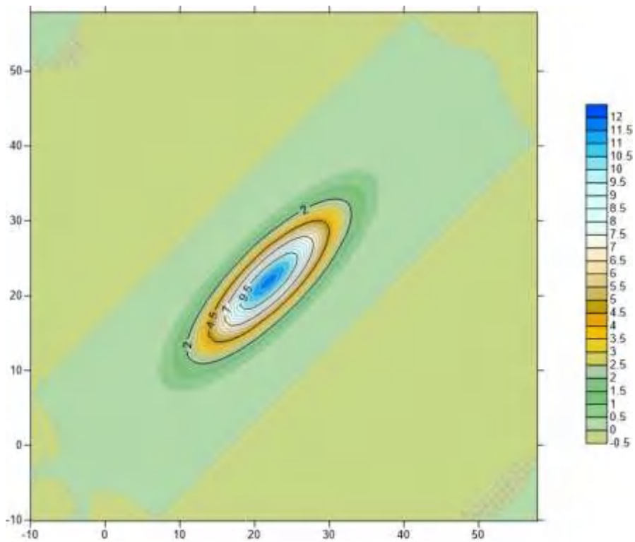
图 6.6-5 假定事故状态下地下水中污染物氰化物 1000d 的运移情况
