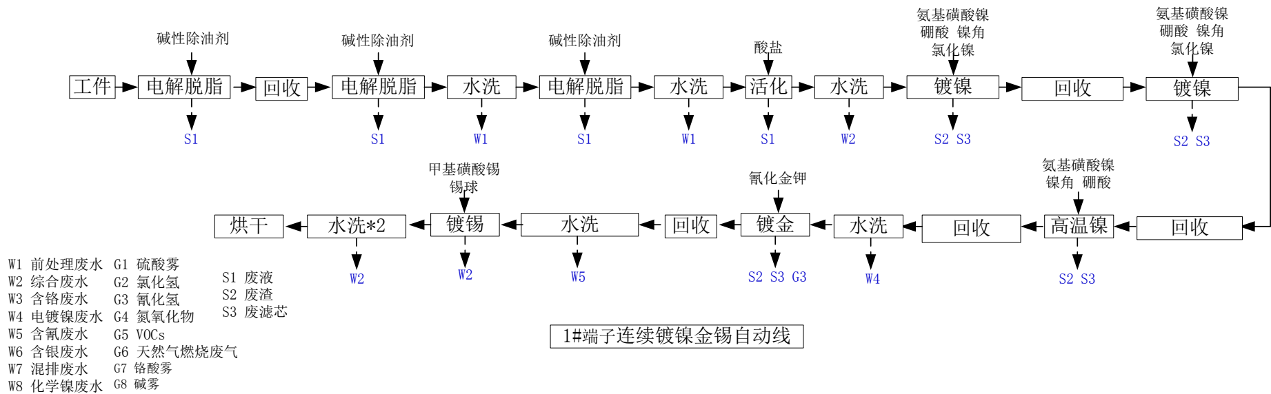
图 4.1-10 1#端子连续镀镍金锡自动线生产工艺及产污环节
