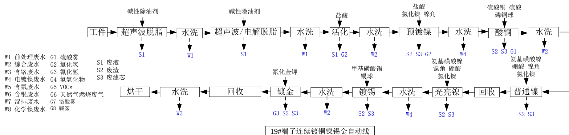
图 4.1-28 19#端子连续镀铜镍锡金自动线生产工艺及产污环节
