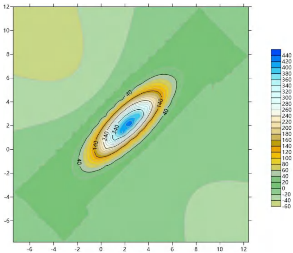
图 6.5-7 假定事故状态下地下水中污染物 \text{COD}_{\text{Mn}100\text{d}} 的运移情况
