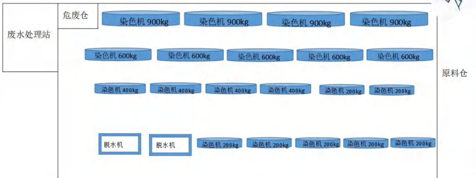
图 4.1-4 项目厂房平面布置图 (1F)
