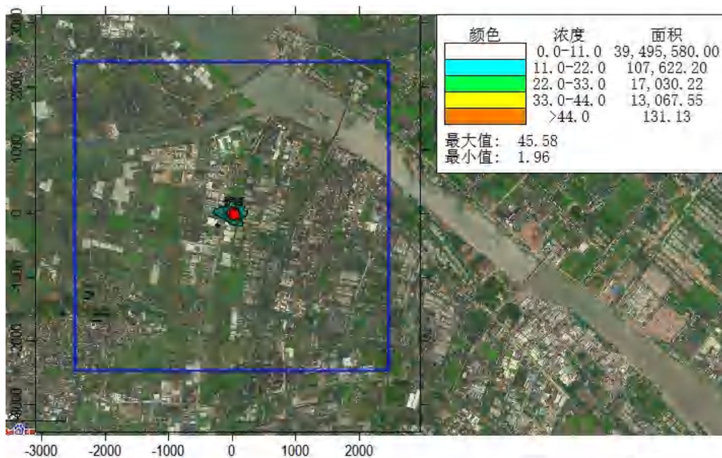
图 6.1-10 NO 2 1 小时平均浓度贡献值分布图(单位: \mu\text{g}/\text{m}^3 )
