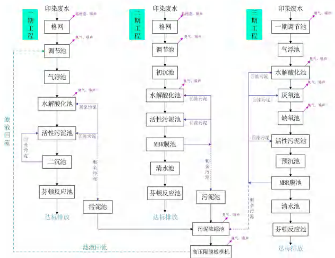
图 7.2-4 一期、二期、三期工程生产工艺及产污环节
