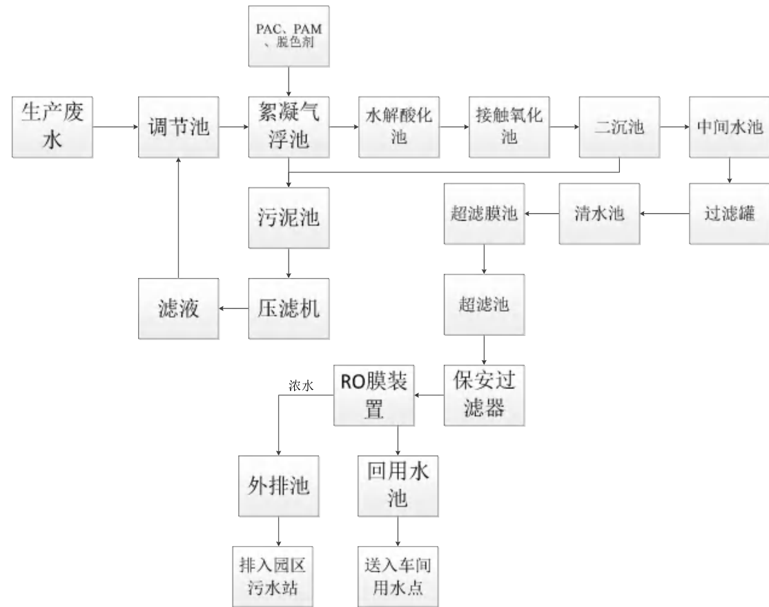
图 7.2-3 废水处理工艺图
