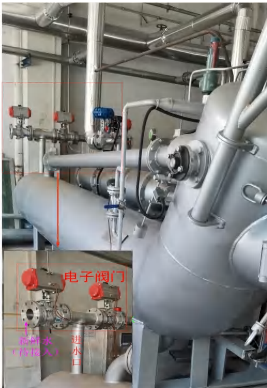
图 6.2-2 染色机进水口示意图
