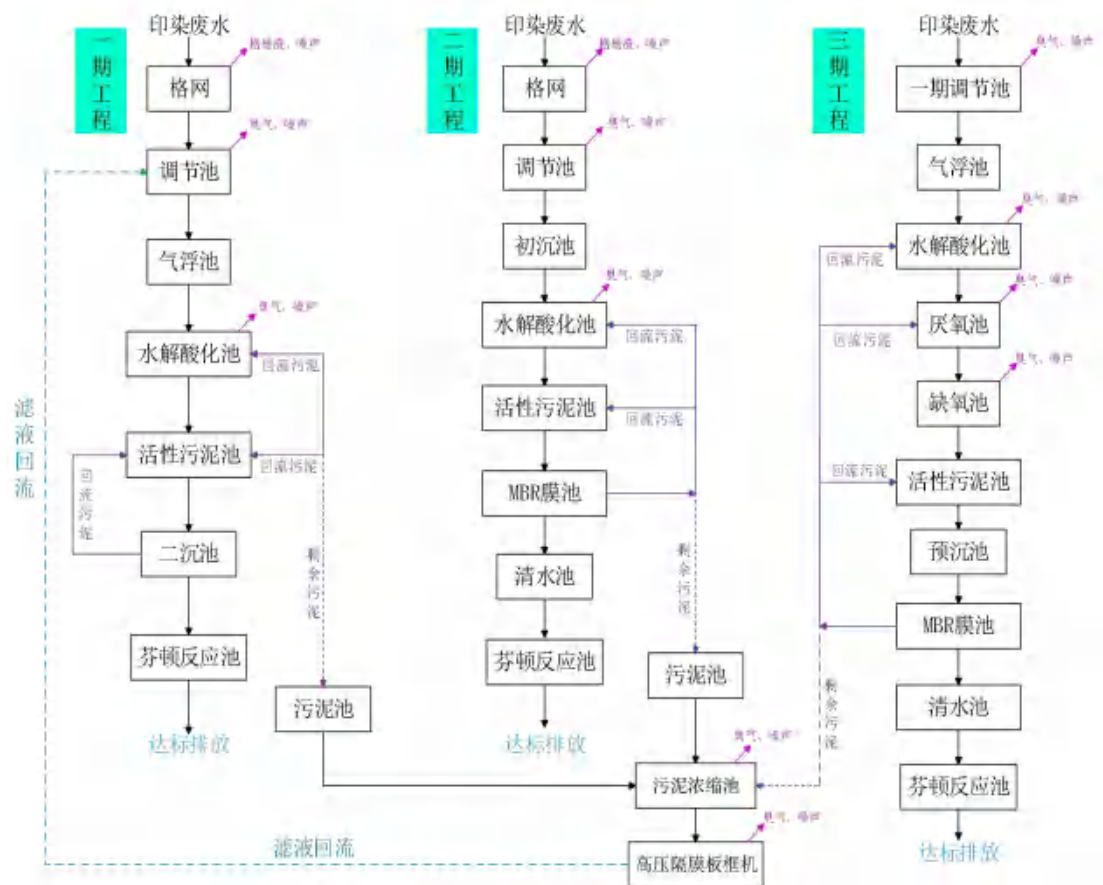
图 6.2-4 一期、二期、三期工程生产工艺及产污环节
