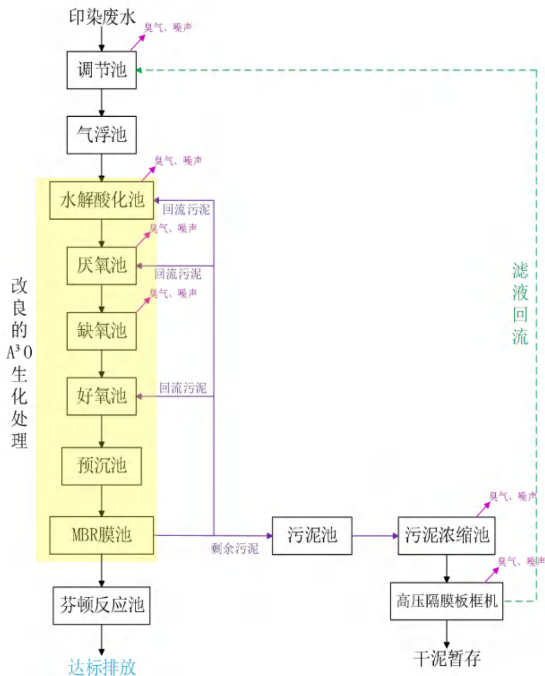
图 7.2-5 四期工程生产工艺及产污环节
