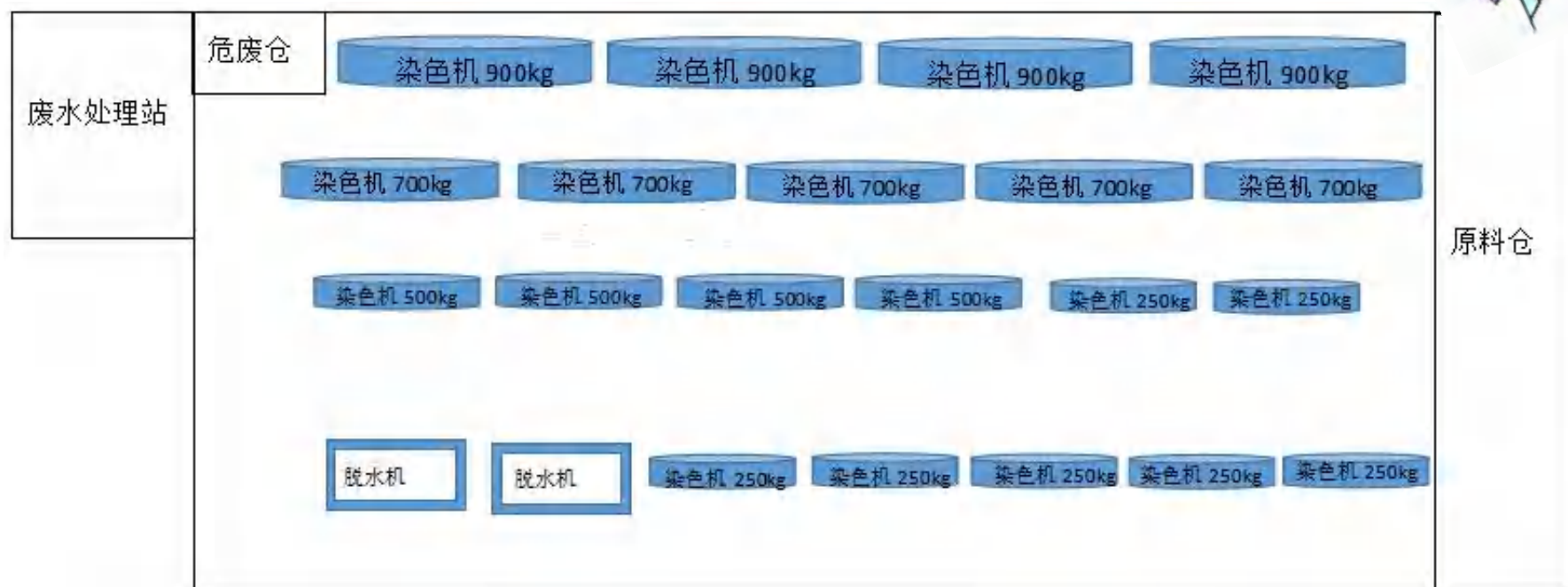
图 4.1-4 项目厂房平面布置图 (1F)
