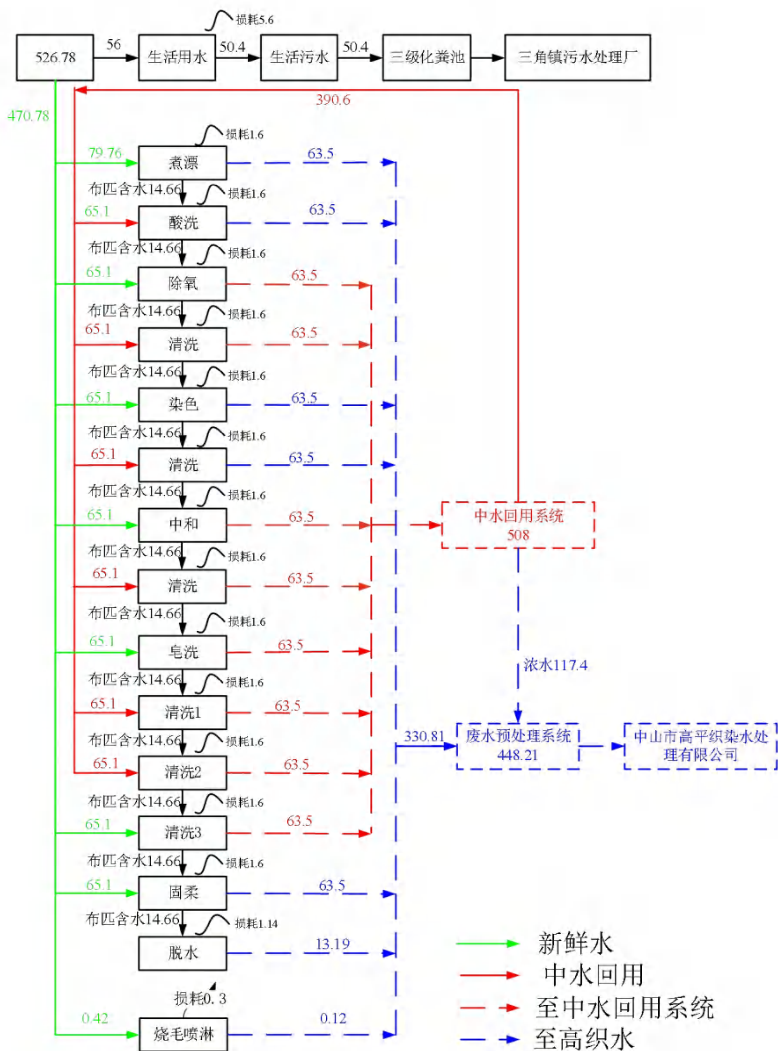
图 4.1-7 项目水平衡图
