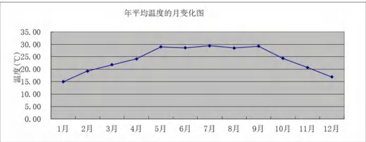
图 6.1-2 中山市 2021 年平均气温月变化曲线
