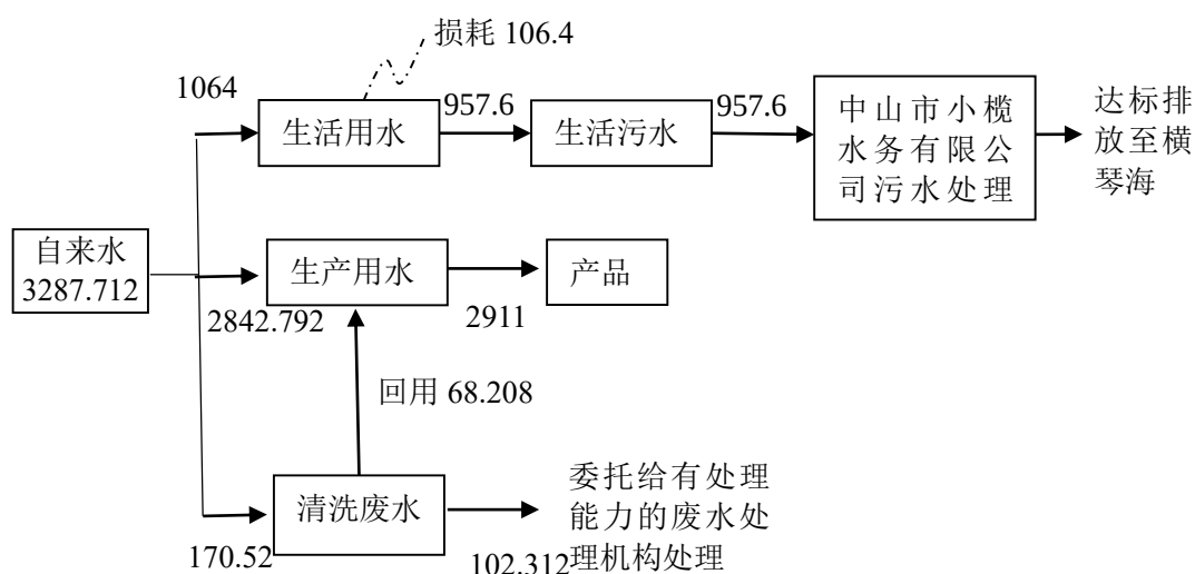
图 1 全厂水平衡图（单位：t/a）
