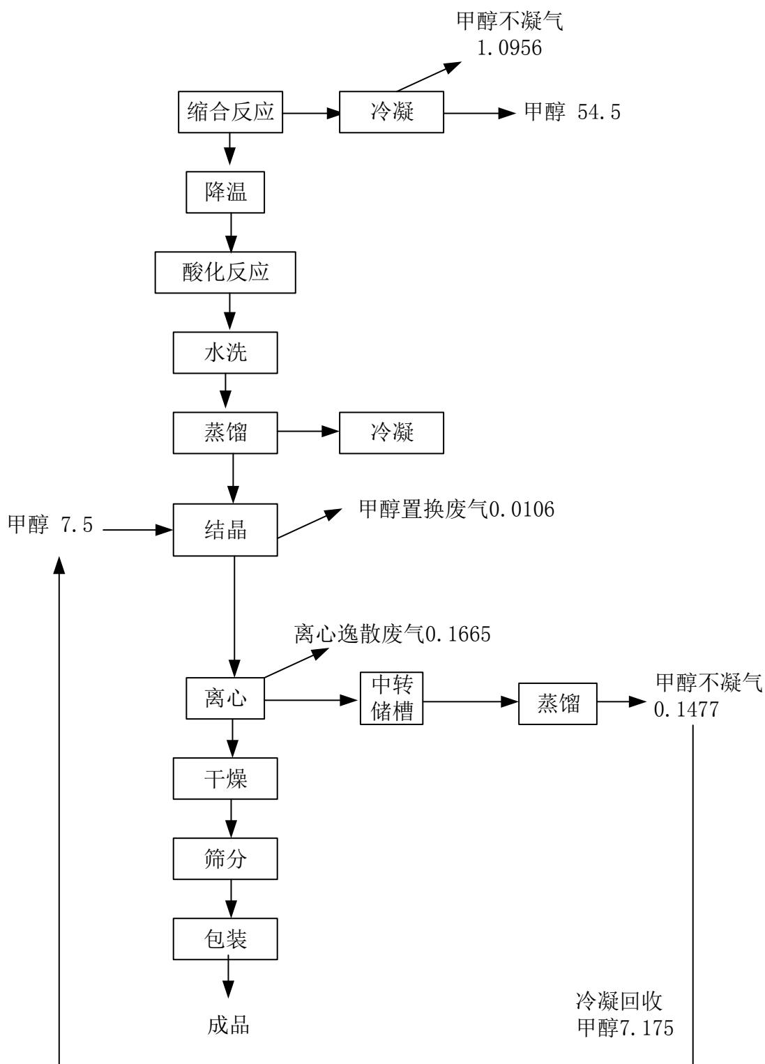
图 4.3-2 全厂甲醇平衡图 (t/a)
