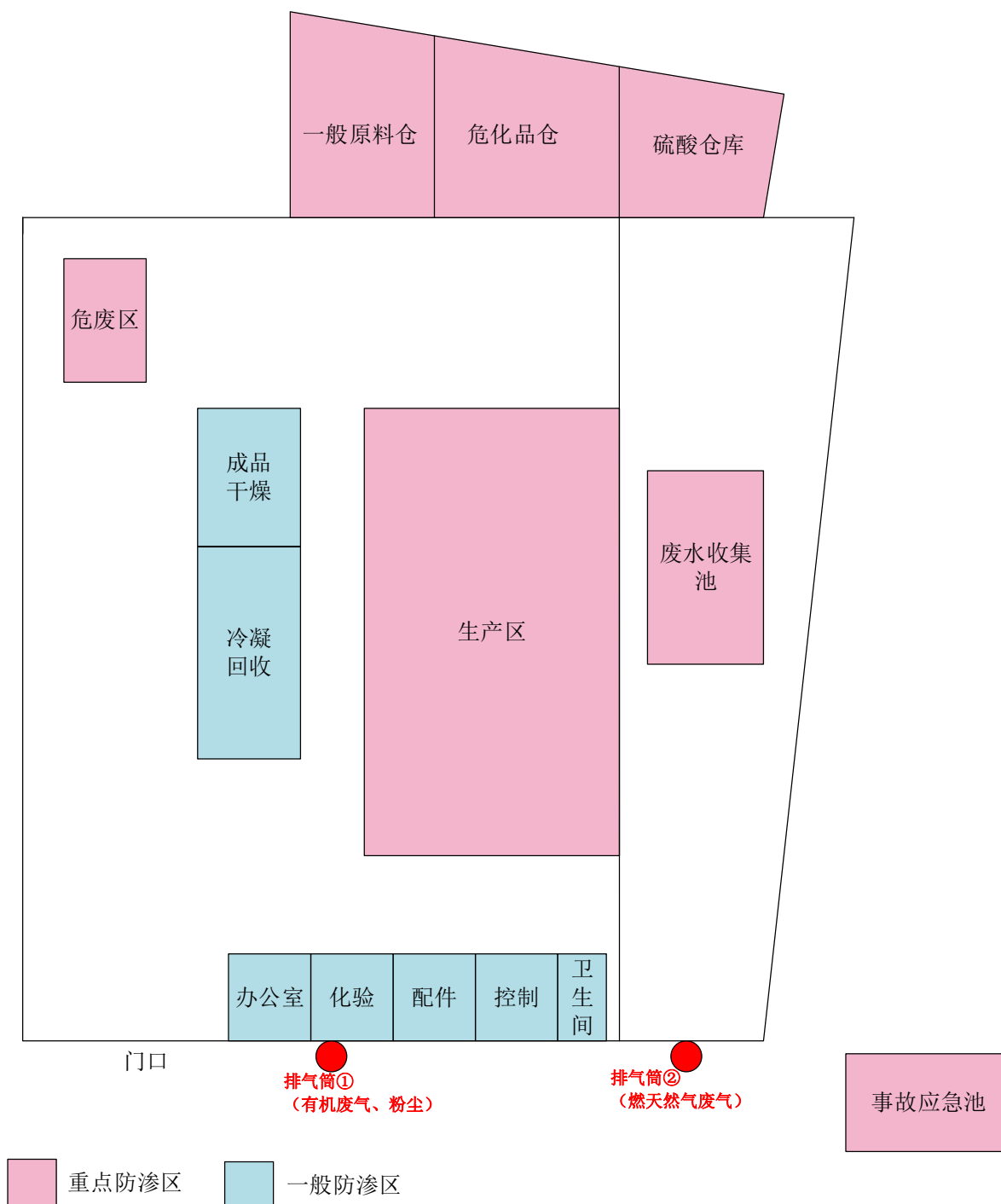
图 6.5-1 项目地下水分区防渗图
