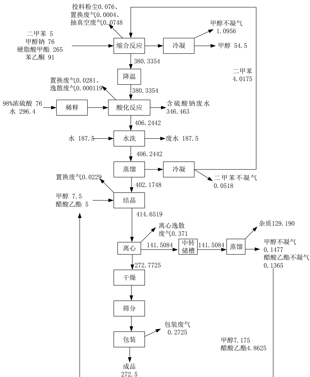
图 4.3-1 全厂物料平衡图 (t/a)
