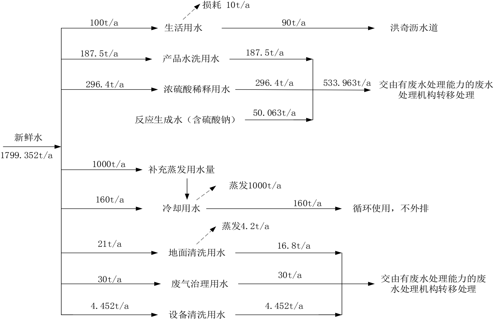
图 4.3-4 水平衡图 (单位 t/a)
