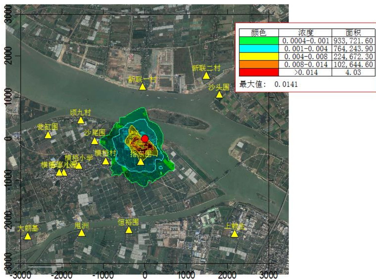
图 6.1-22 PM_{2.5} 1 小时平均浓度贡献值等值线图(单位: mg/m^3 )
