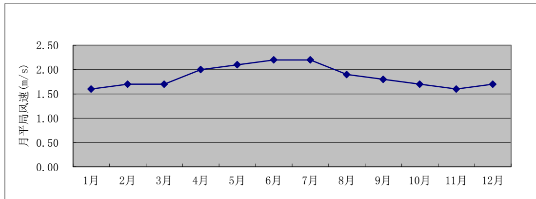
图 6.1-2 中山市 1999~2018 年逐月平均风速变化曲线
