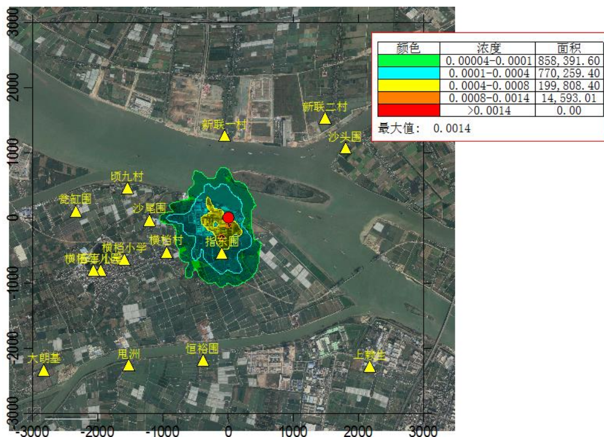
图 6.1-23 PM 2.5 日平均浓度贡献值等值线图(单位: mg/m 3 )
