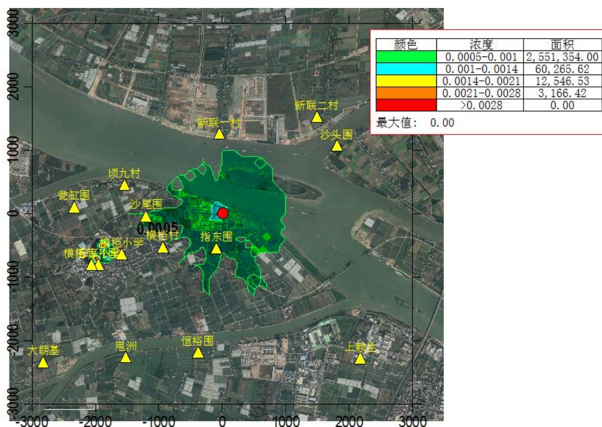
图 6.1-16 二氧化硫 1 小时平均浓度贡献值等值线图(单位: mg/m 3 )
