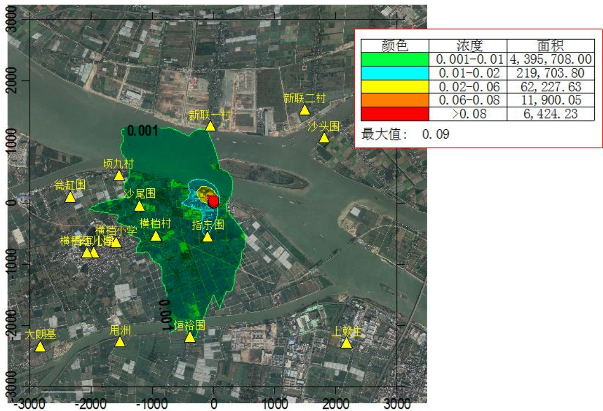
图 6.1-12 PM 10 年均浓度贡献值等值线图(单位: mg/m3)
