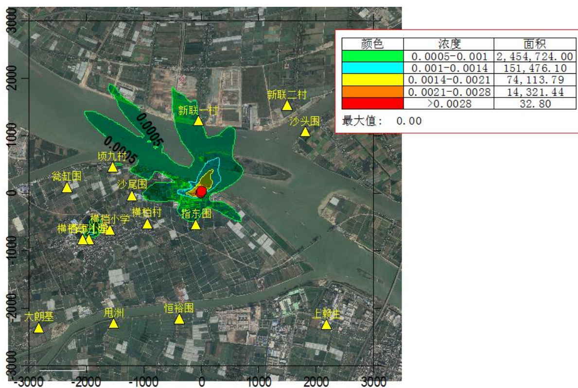
图 6.1-15 硫酸雾日平均浓度贡献值等值线图(单位: mg/m 3 )
