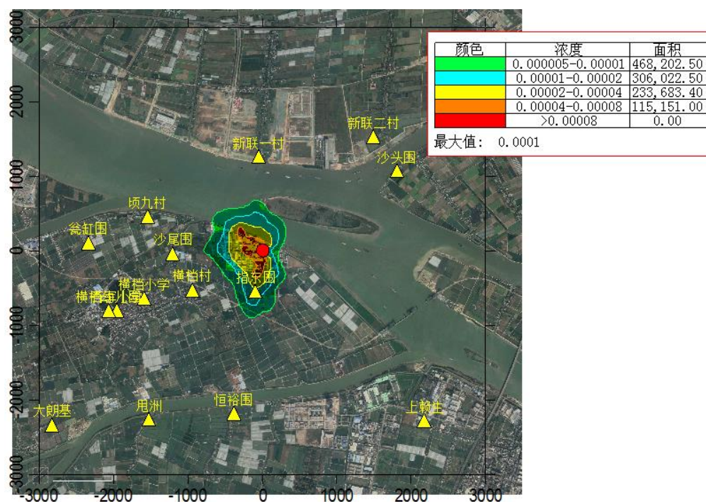
图 6.1-24 PM_{2.5} 年平均浓度贡献值等值线图(单位: mg/m^3 )
