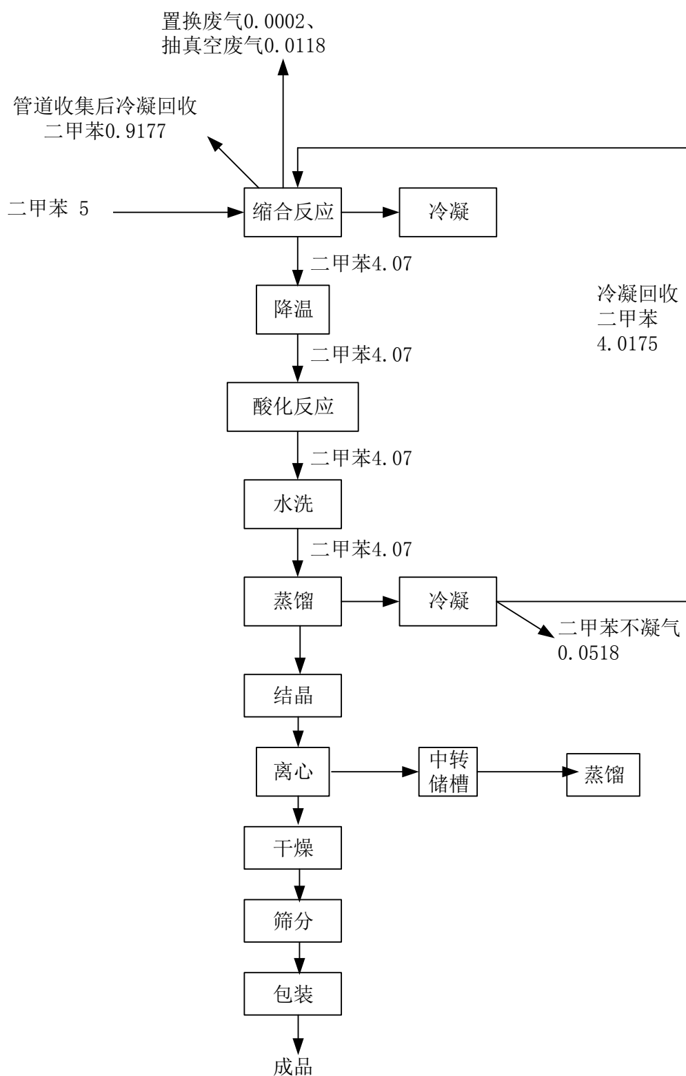
图 4.3-3 全厂二甲苯平衡图 (t/a)
