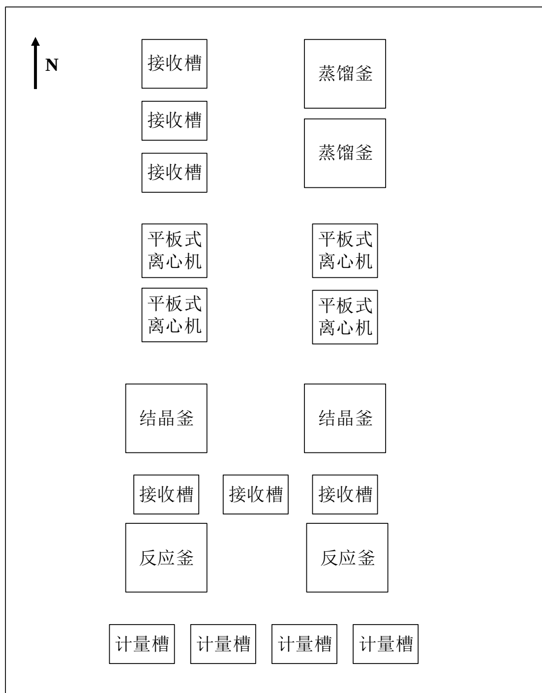
图 3.1-4 生产区平面布置图
