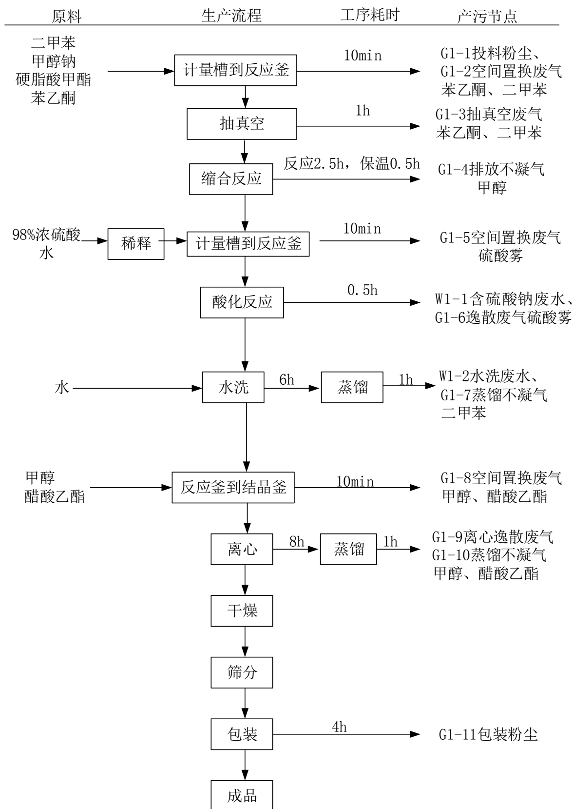
图 4.1-1 硬脂酰苯甲酰甲烷产污环节图
