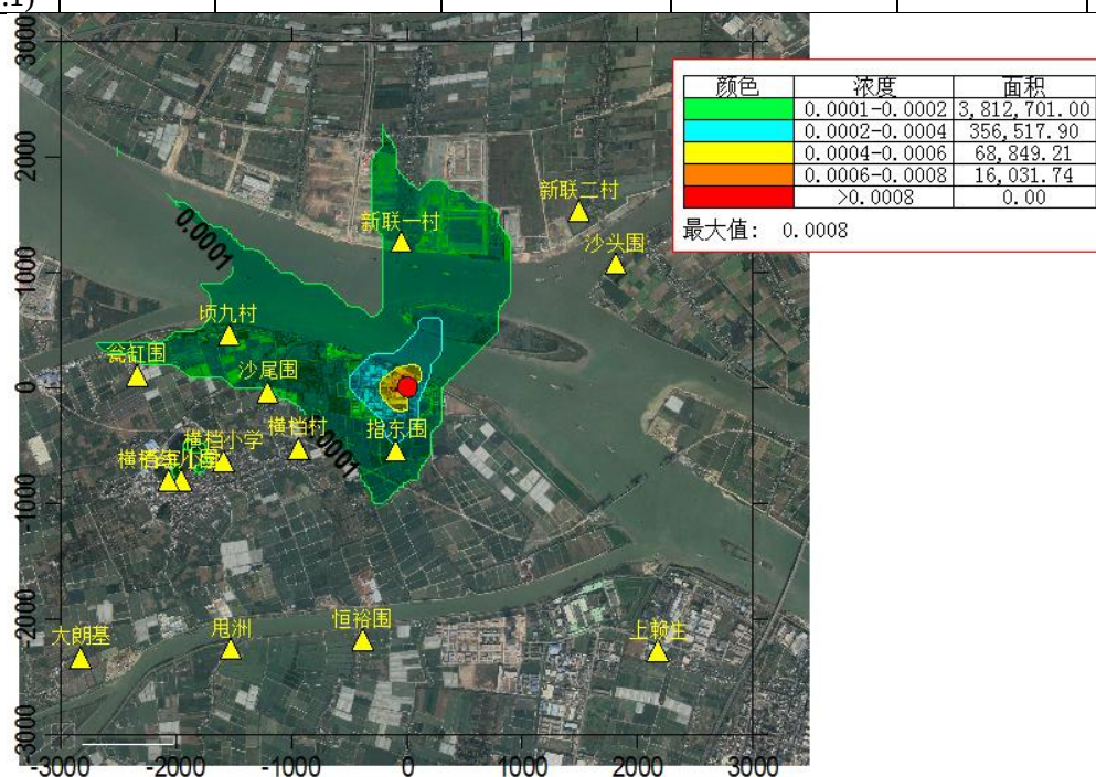
图 6.1-18 二氧化硫年平均浓度贡献值等值线图(单位: mg/m 3 )
