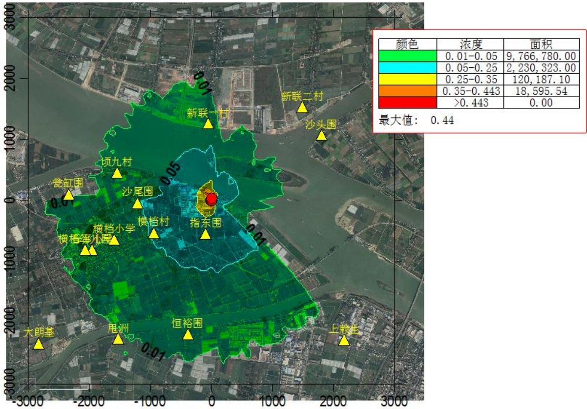
图 6.1-10 PM 10 1 小时均浓度贡献值等值线图(单位: mg/m3)
