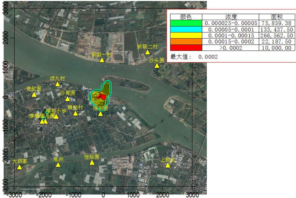
图 6.1-21 氮氧化物年平均浓度贡献值等值线图(单位: mg/m 3 )
