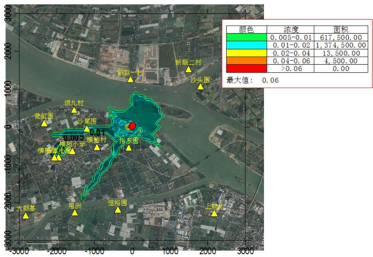
图 6.1-14 硫酸雾 1 小时平均浓度贡献值等值线图(单位: mg/m3)
