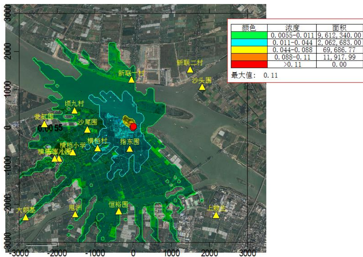
图 6.1-9 TVOC 8 小时均浓度贡献值等值线图(单位: mg/m 3 )
