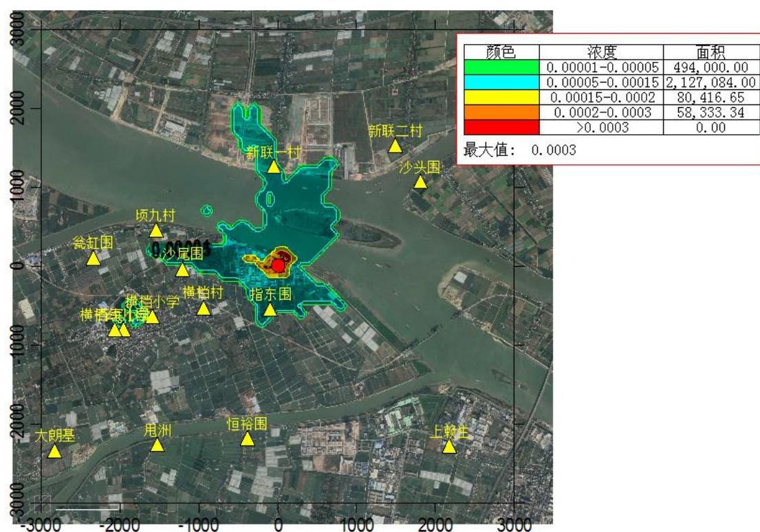
图 6.1-17 二氧化硫日平均浓度贡献值等值线图(单位: mg/m3)
