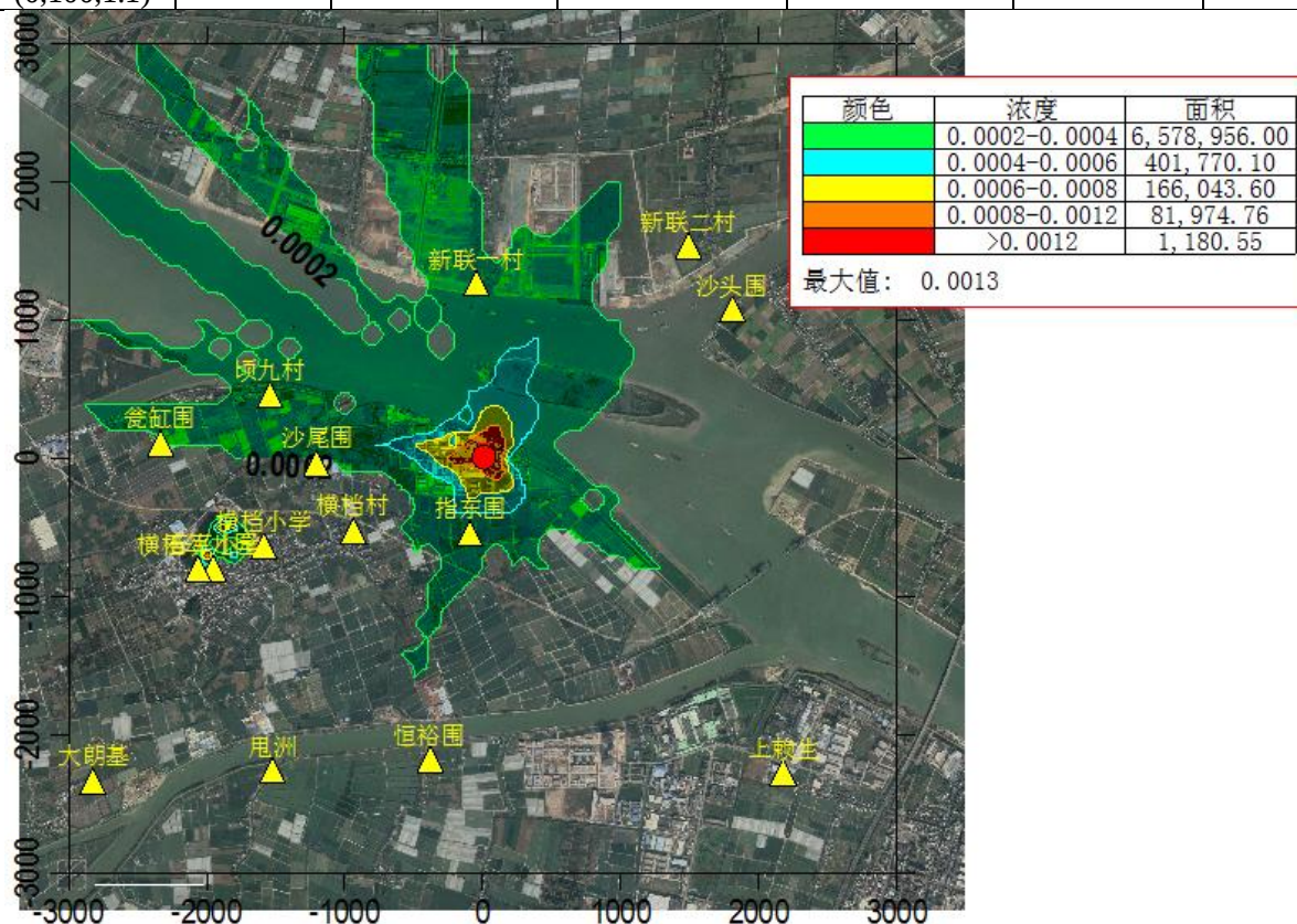
图 6.1-20 氮氧化物日平均浓度贡献值等值线图(单位: mg/m³)
