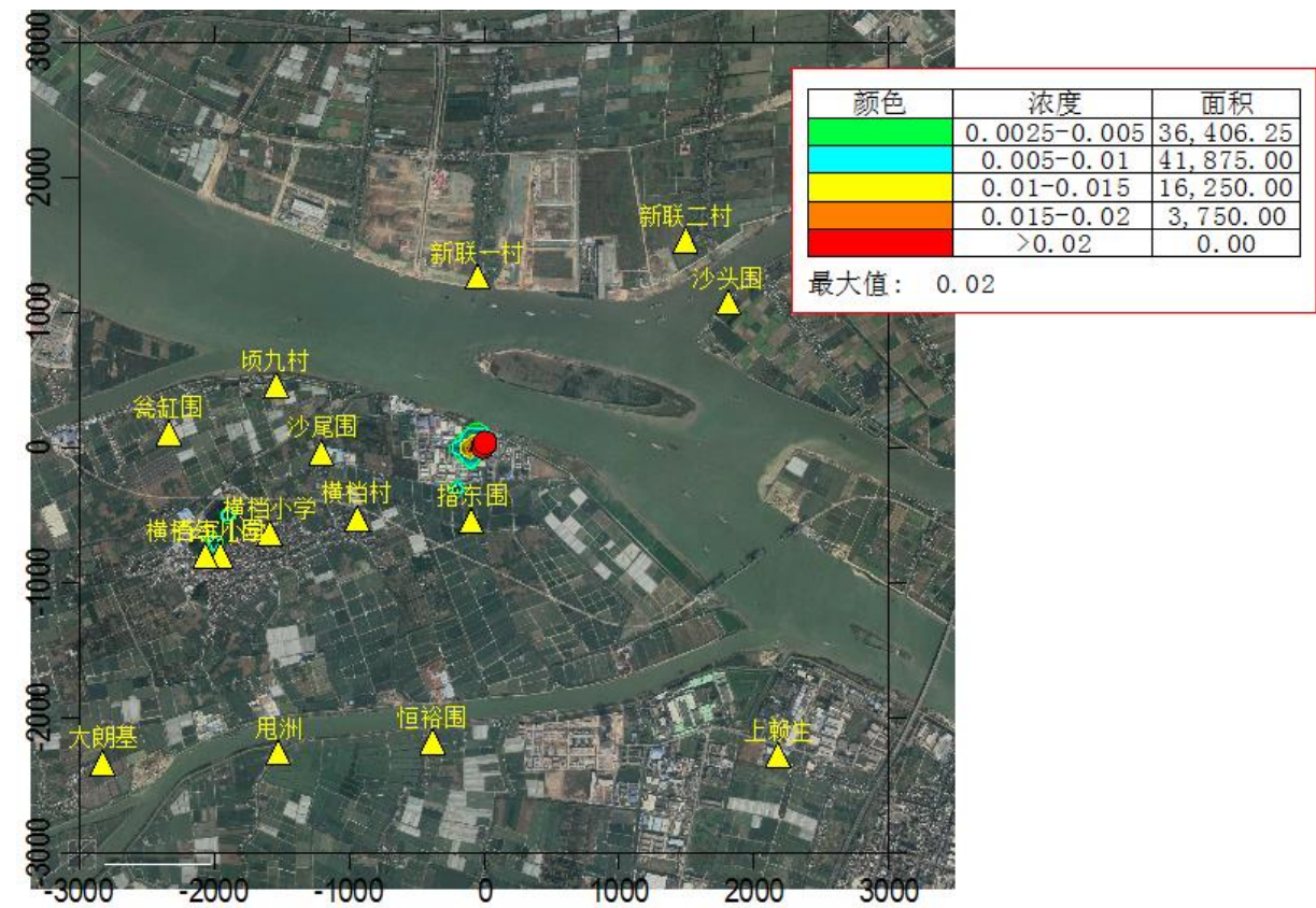
图 6.1-13 二甲苯 1 小时平均浓度贡献值等值线图(单位: mg/m 3 )
