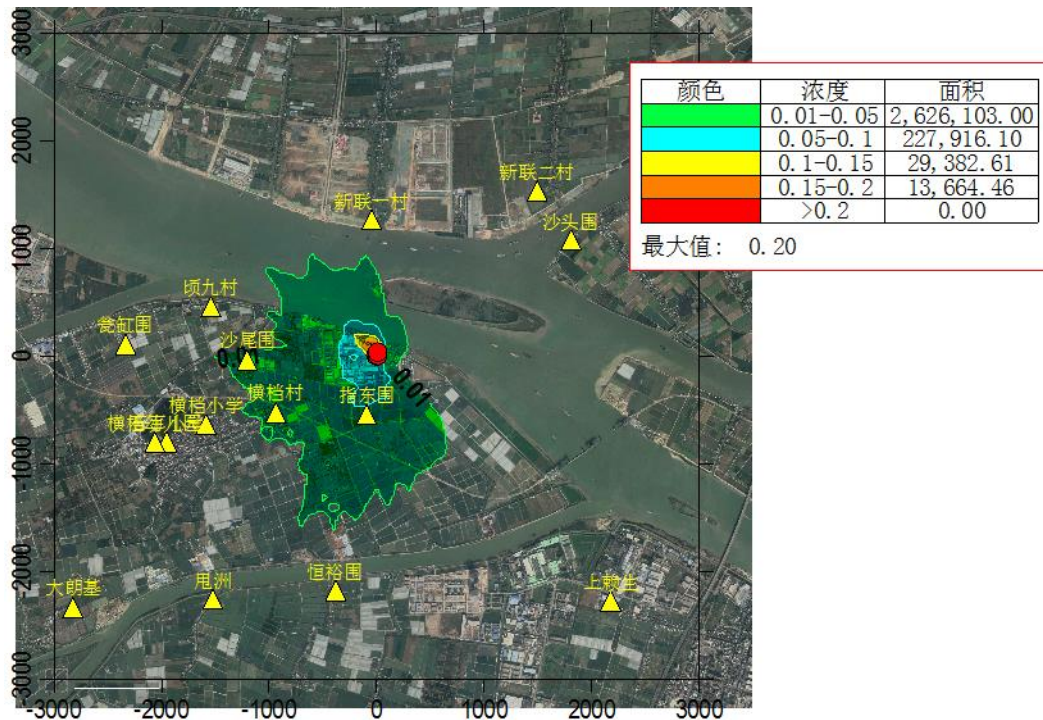
图 6.1-11 PM_{10} 日均浓度贡献值等值线图(单位: mg/m^3 )
