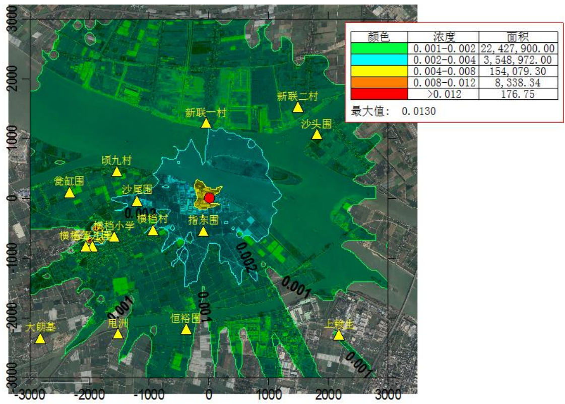
图 6.1-19 氮氧化物 1 小时平均浓度贡献值等值线图(单位: mg/m3)
