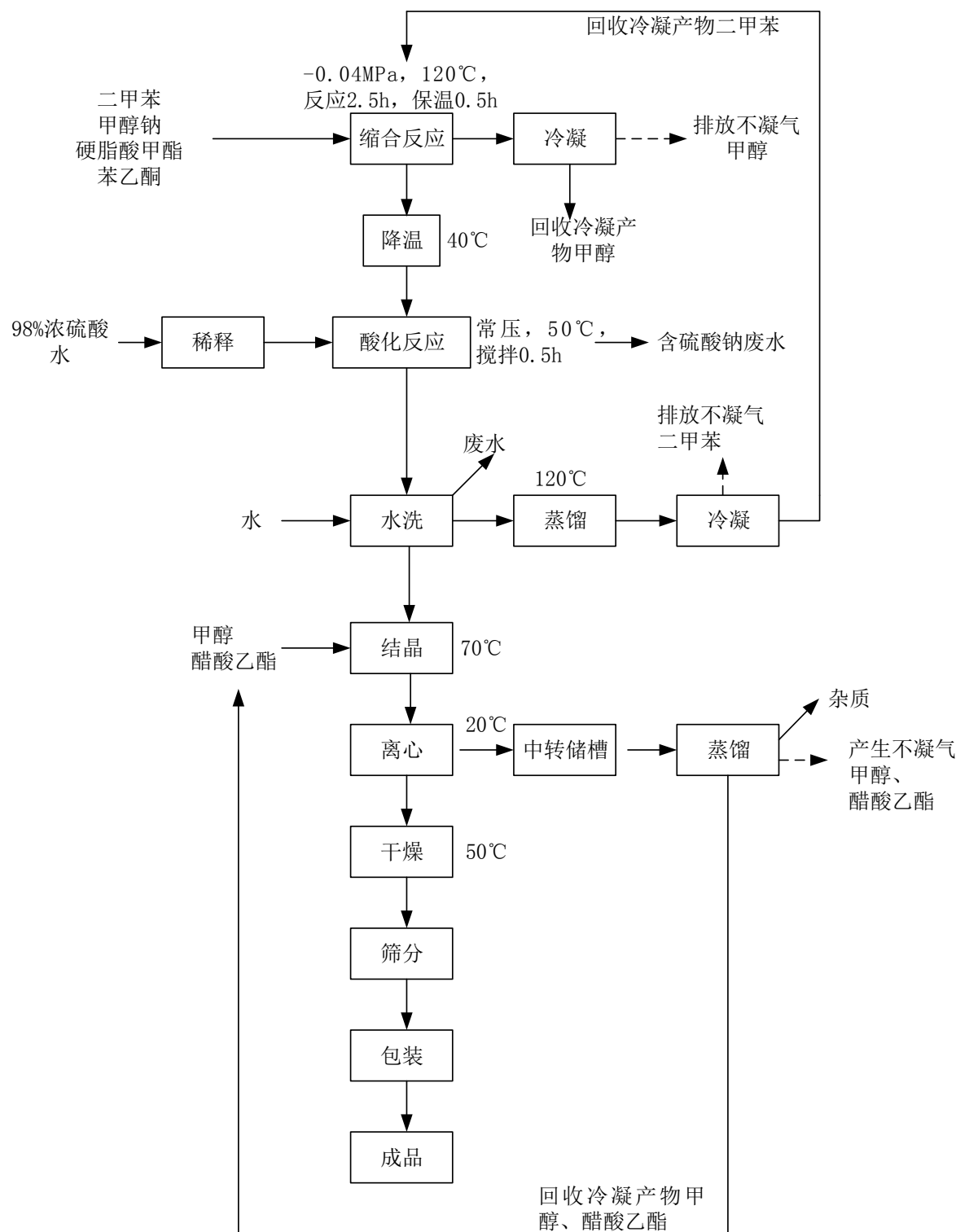
图 3.5-1 硬脂酰苯甲酰甲烷的生产流程图
