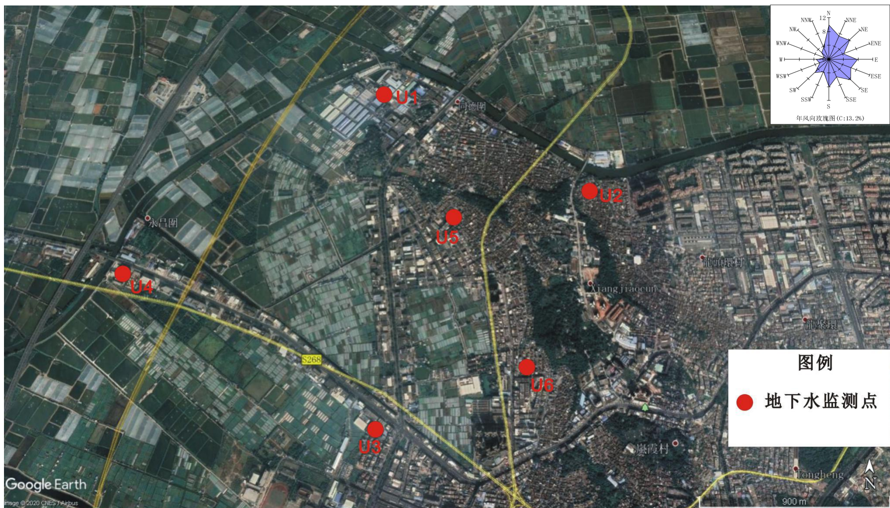
图 4.5-1 项目地下水环境监测布点图
