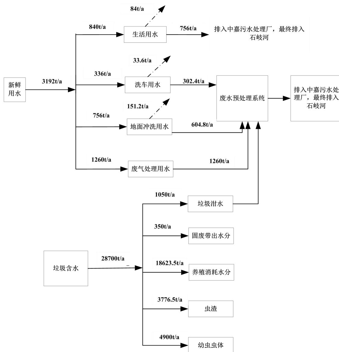
3.4-5 项目二期工程建成后水平衡图
