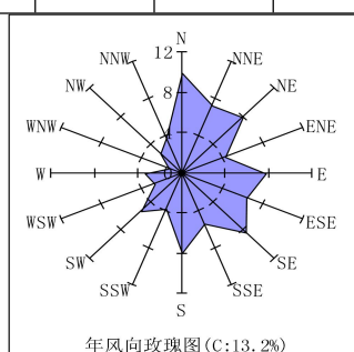
图 5.1-3 中山气象站风向玫瑰图 (1999~2018 年)
