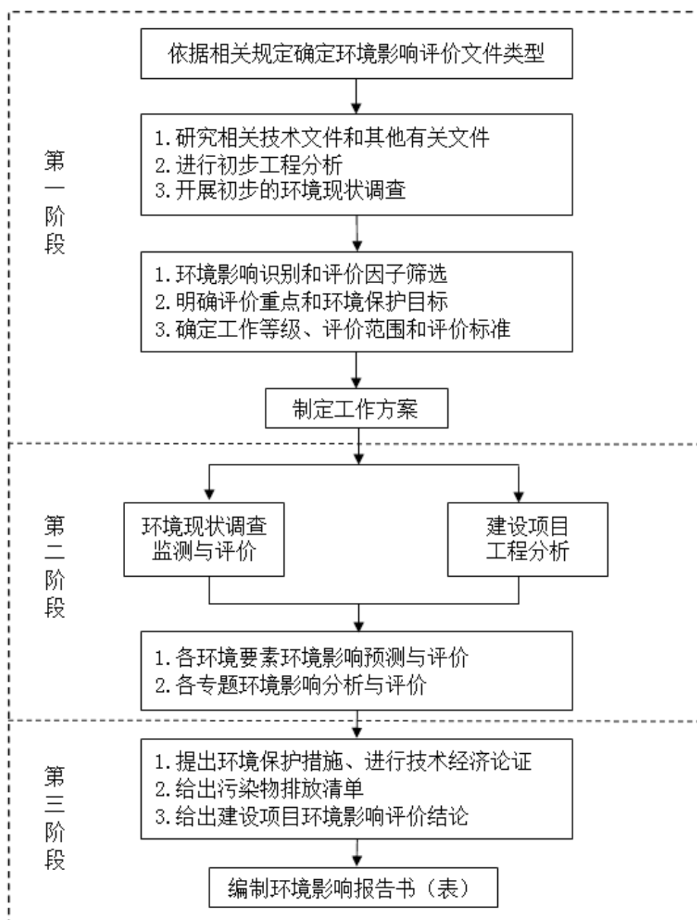
图 1.4-1 本项目环评工作流程图
