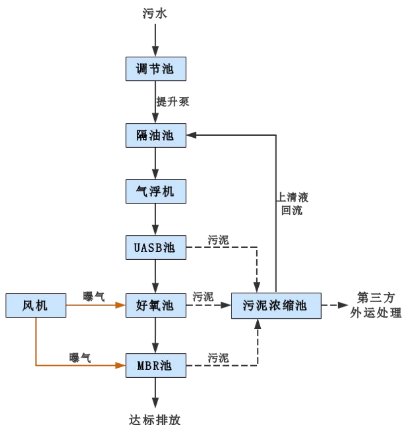
图7.1-3生产废水预处理工艺流程图
