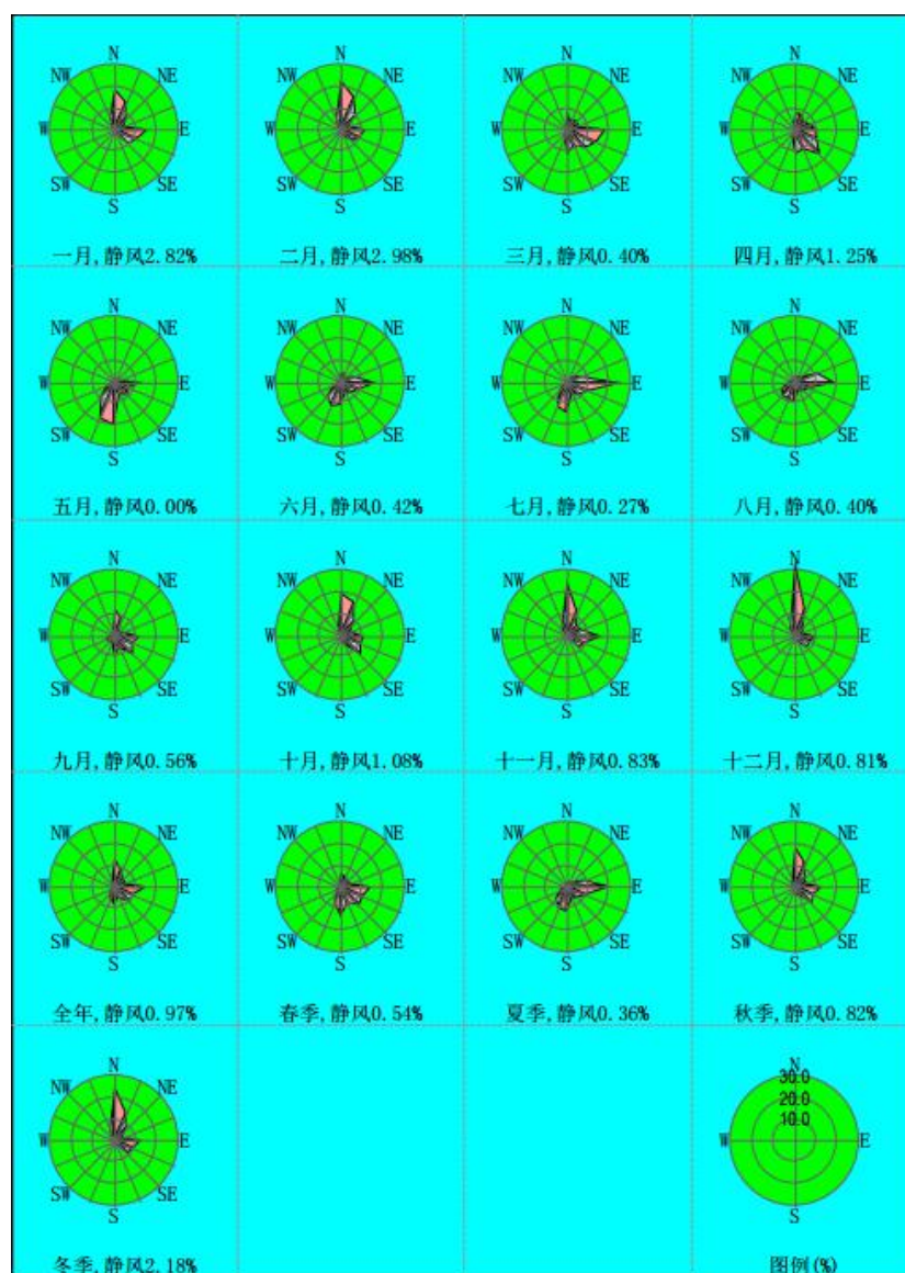
图 5.1-7 中山市 2018 年风频玫瑰图
