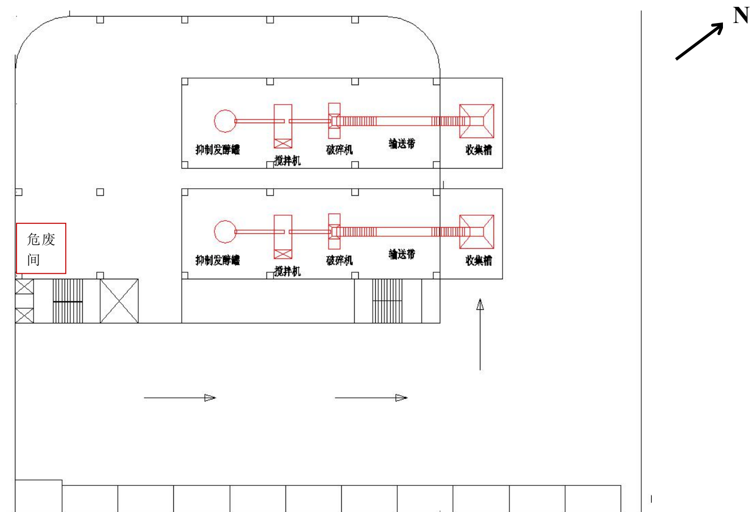
图 3.4-3a 项目平面布置图（首层前处理车间）
