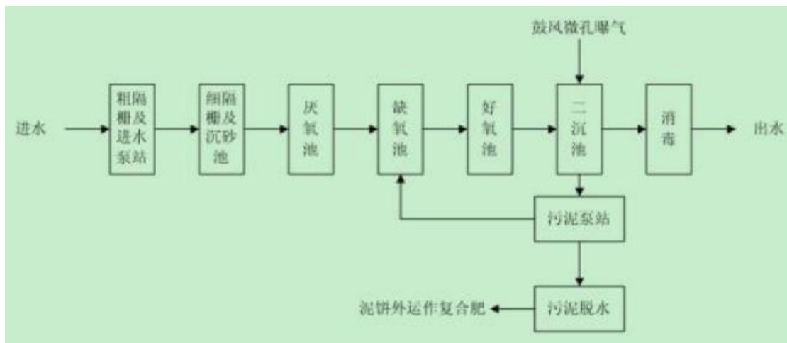
图 7.1-2 中山市中嘉污水处理厂污水处理工艺
