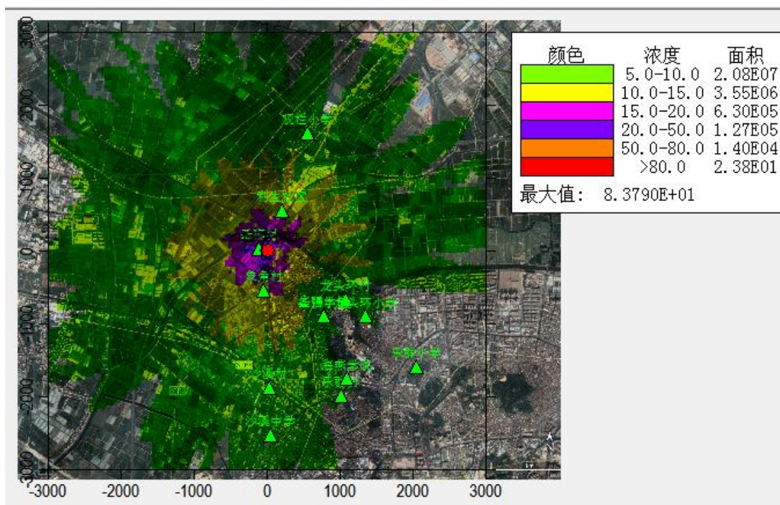
图 6.1-9 氨 1 小时平均浓度贡献值等值线图(单位: \mu\text{g}/\text{m}^3 )
