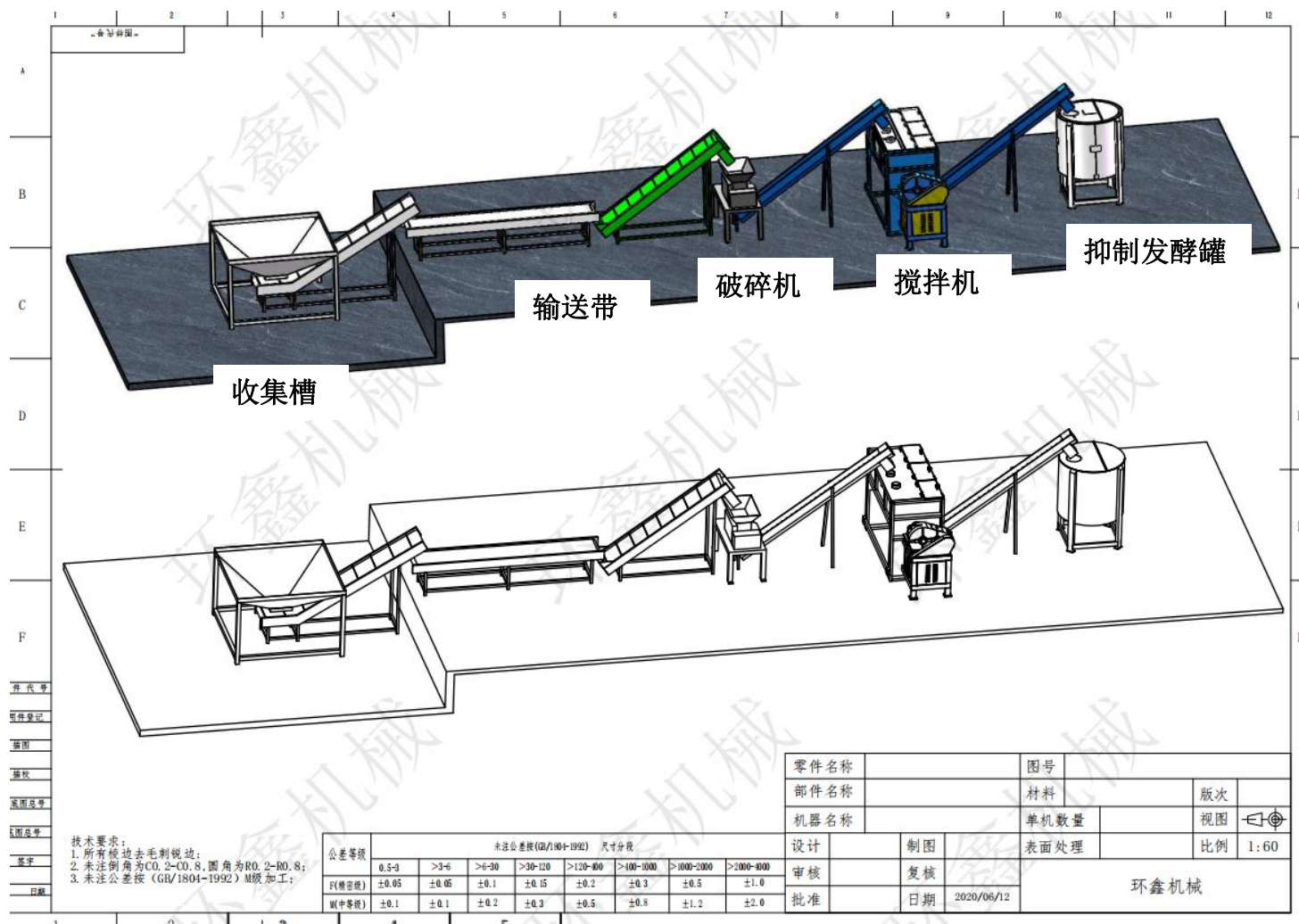
图 3.4-3b 前处理车间三维图
