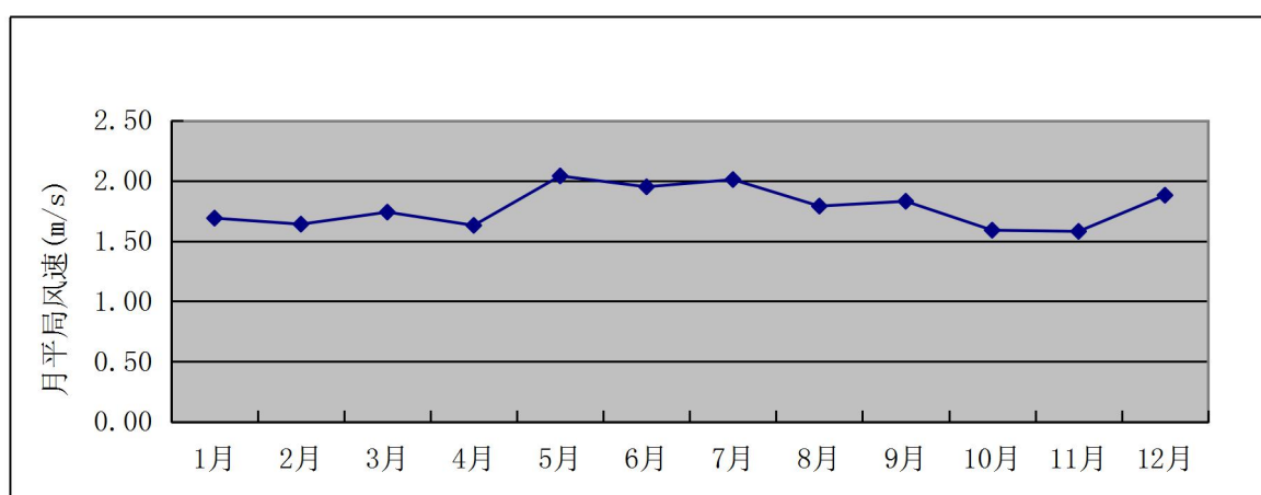
图 5.1-5 中山市 2018 年平均风速的月变化图
