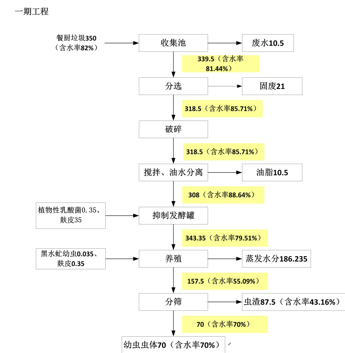
3.4-6 项目一期工程建成后物料衡图 (单位: t)
