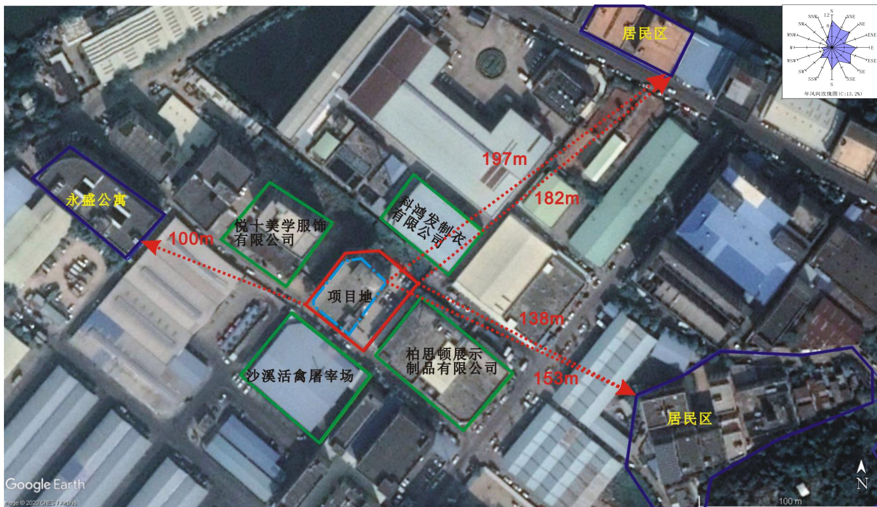
图 3.4-1 项目四至图
