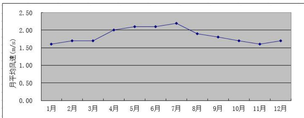
图 5.1-2 1999~2018 年逐月平均风速变化曲线
