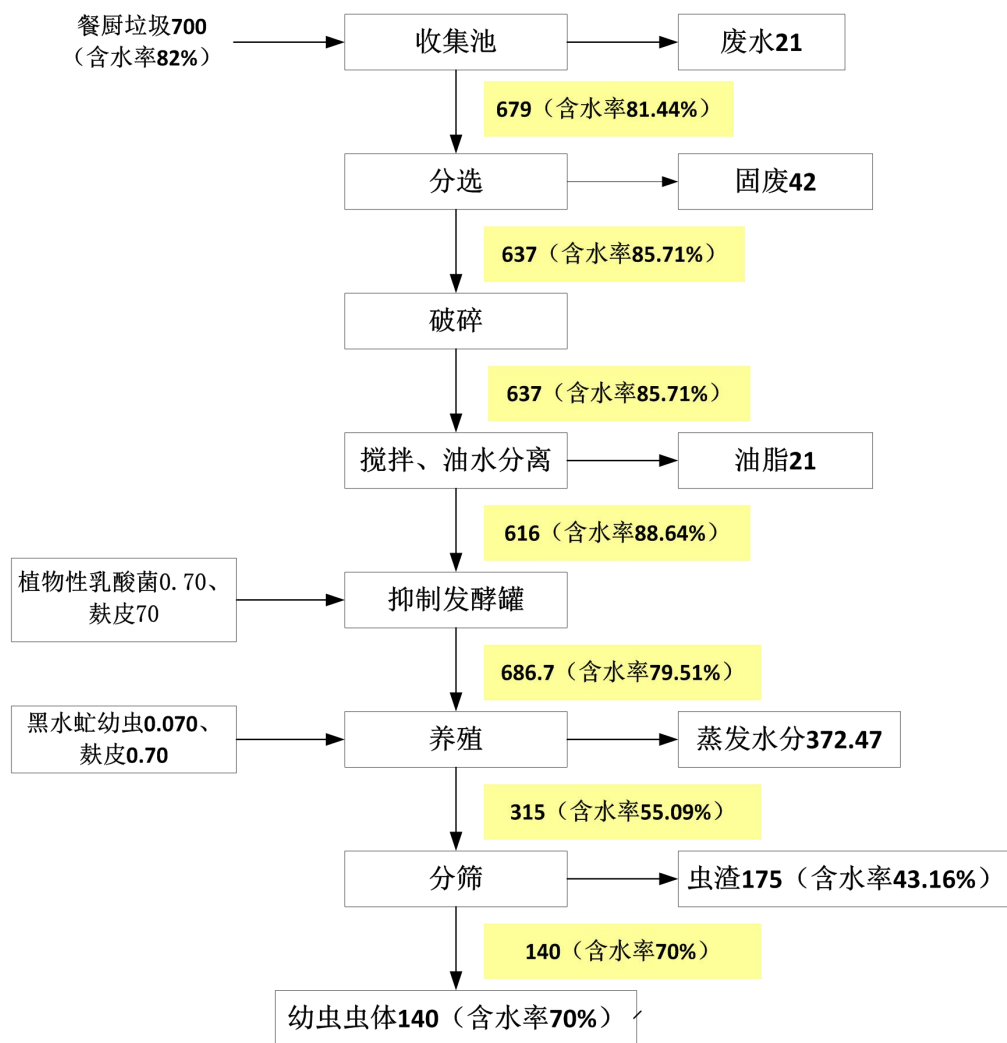
图 3.4-7 项目二期工程建成后物料平衡图（单位：t）
