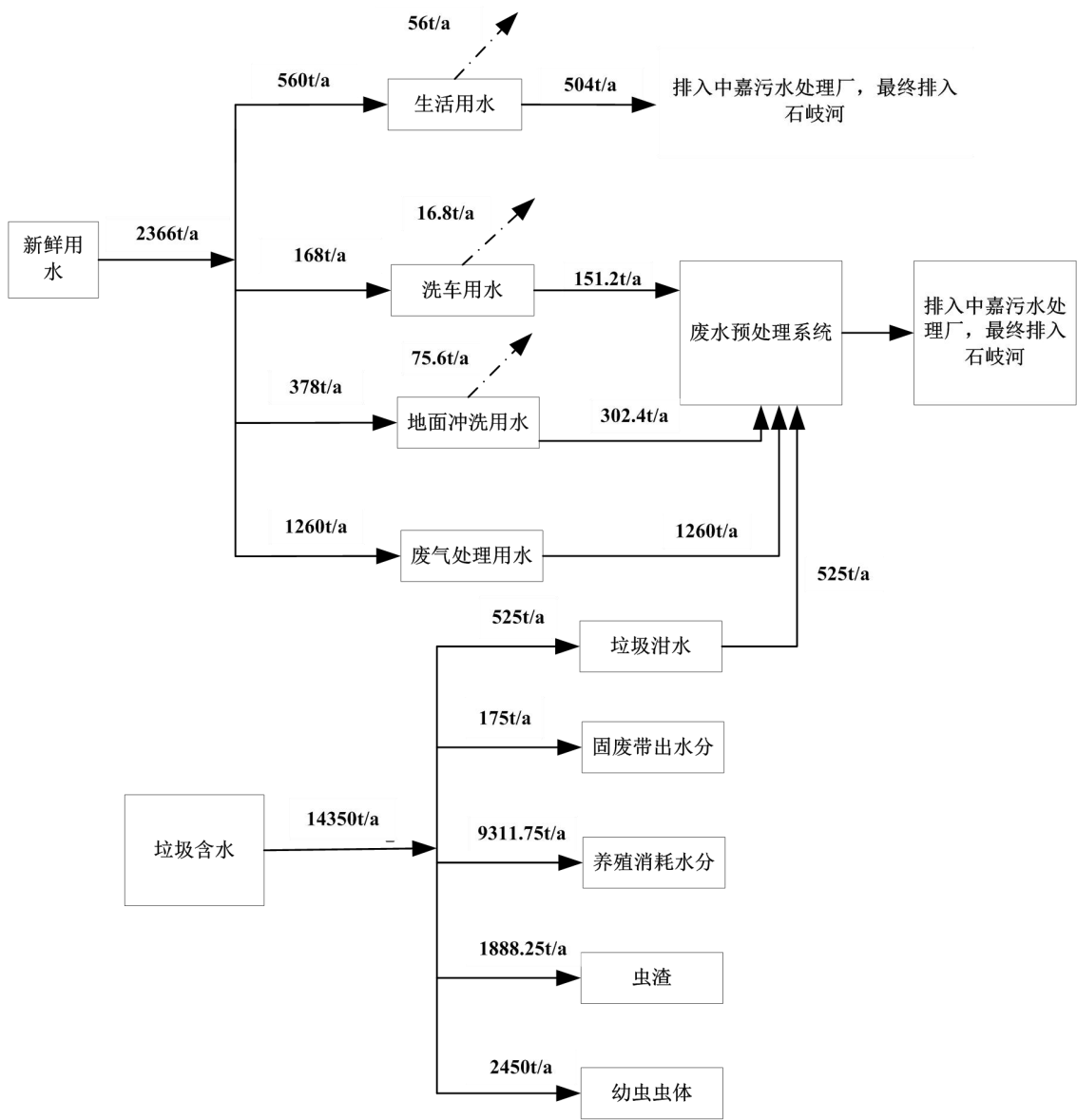
图 3.4-4 项目一期工程建成后水平衡图
