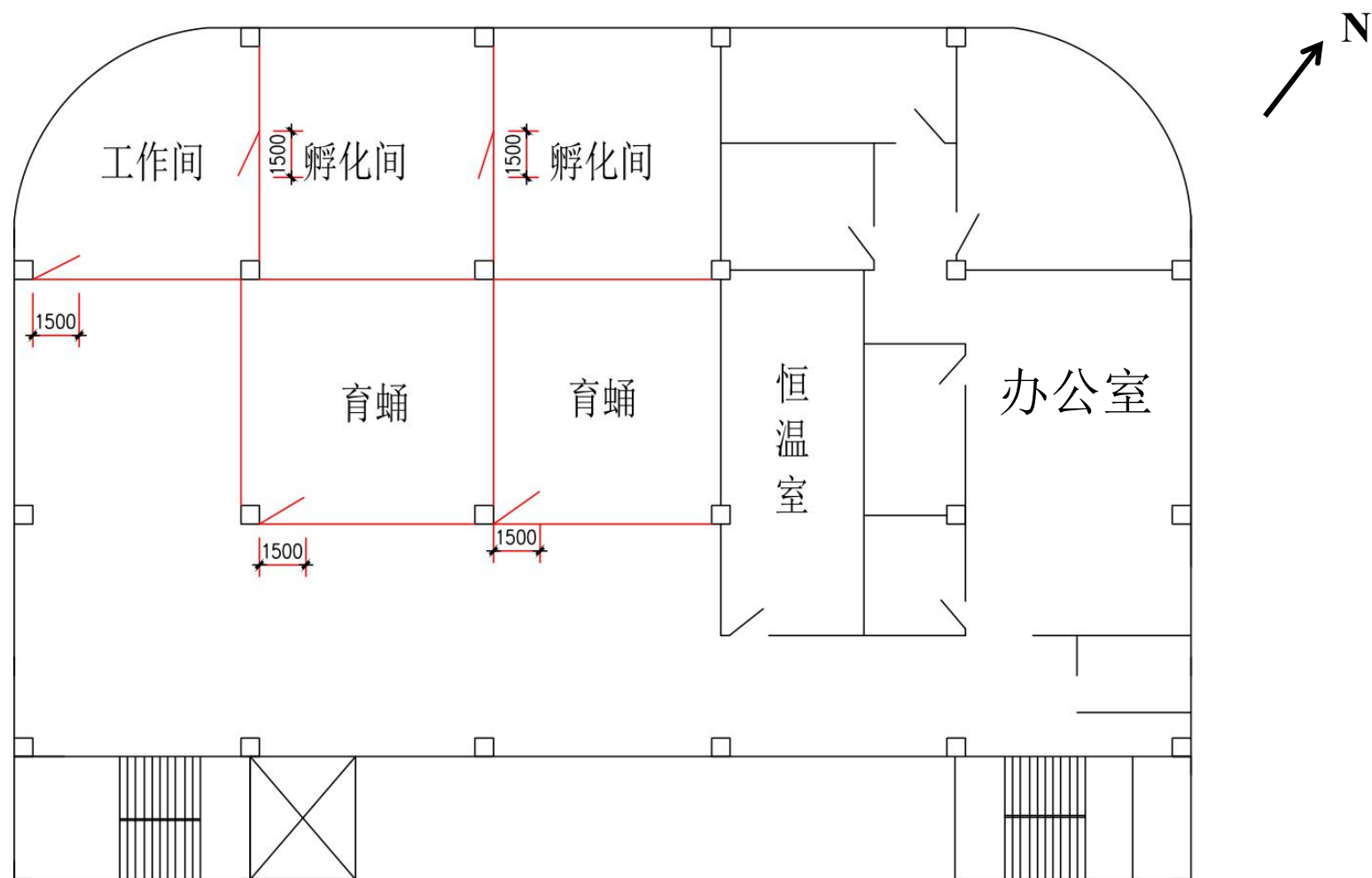
图 3.4-3c 项目平面布置图（二层孵化、育蛹车间、办公室）
