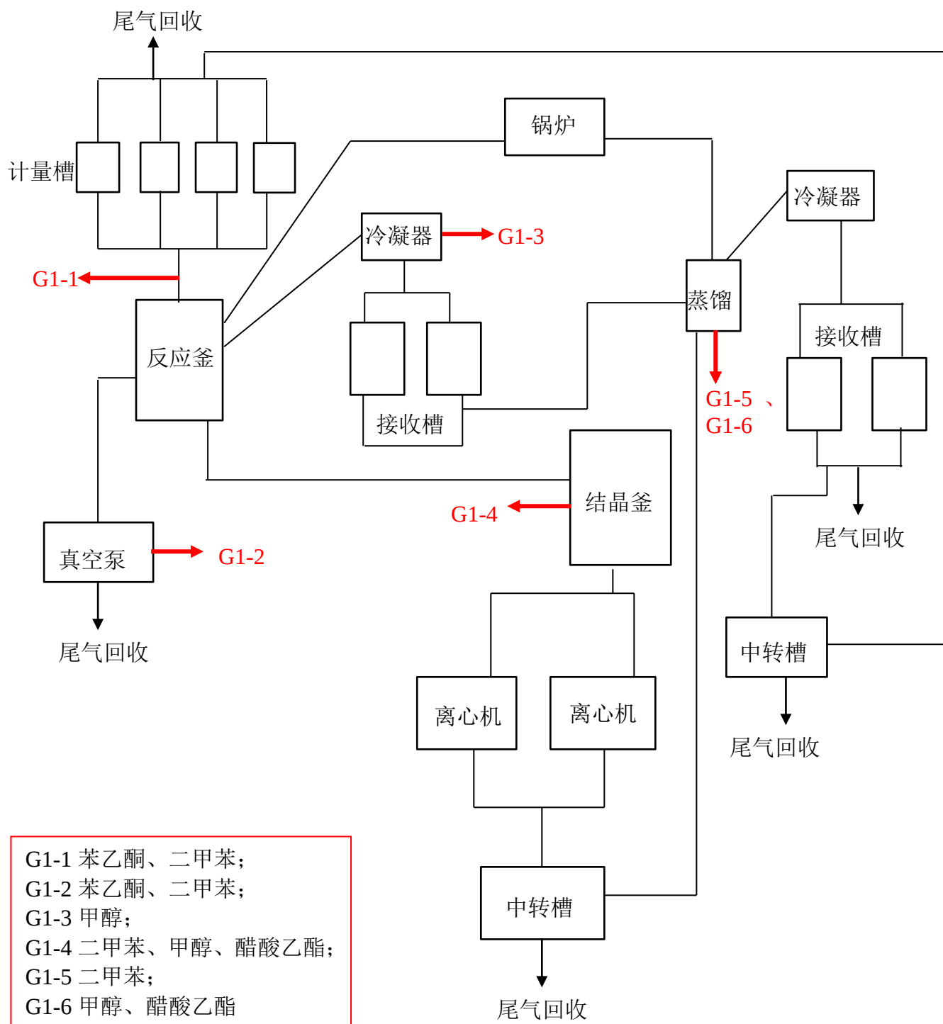
图 4.1-1 硬脂酰苯甲酰甲烷产污环节图
