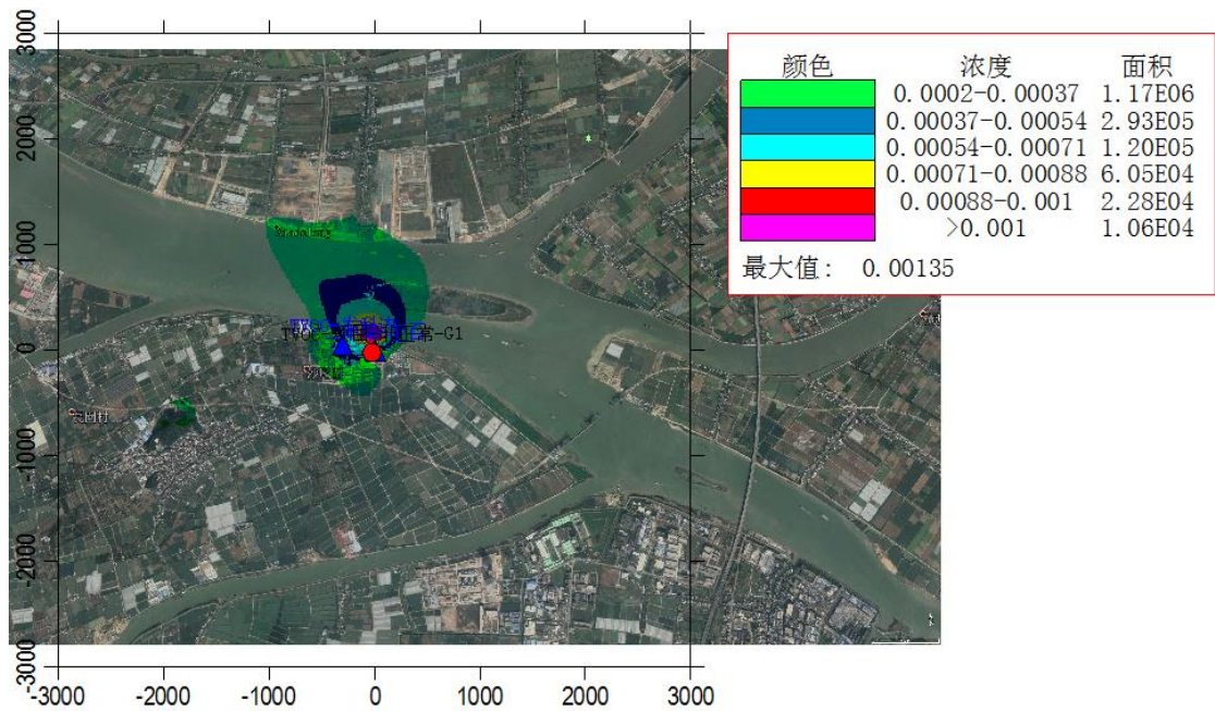
图 6.1-16 TVOC 时均浓度贡献值等值线图(单位: mg/m 3 )
