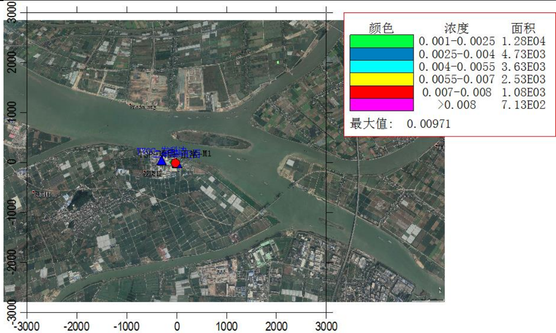
图 6.1-13 TSP 日均浓度贡献值等值线图(单位：mg/m3)
