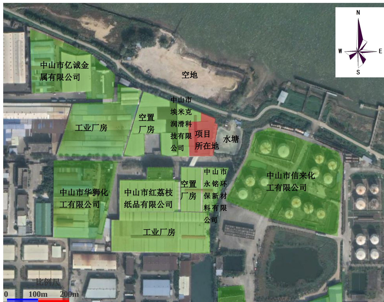
图 3.1-2 建设项目四至图
