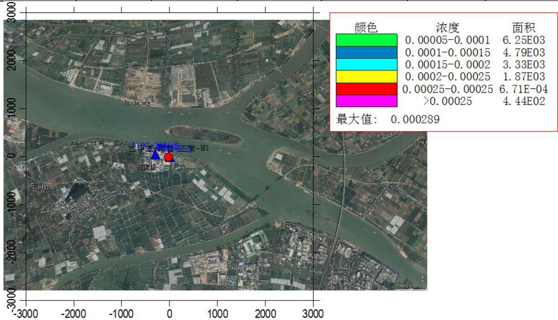
图 6.1-11 二甲苯 1 小时均浓度贡献值等值线图(单位：mg/m3)
