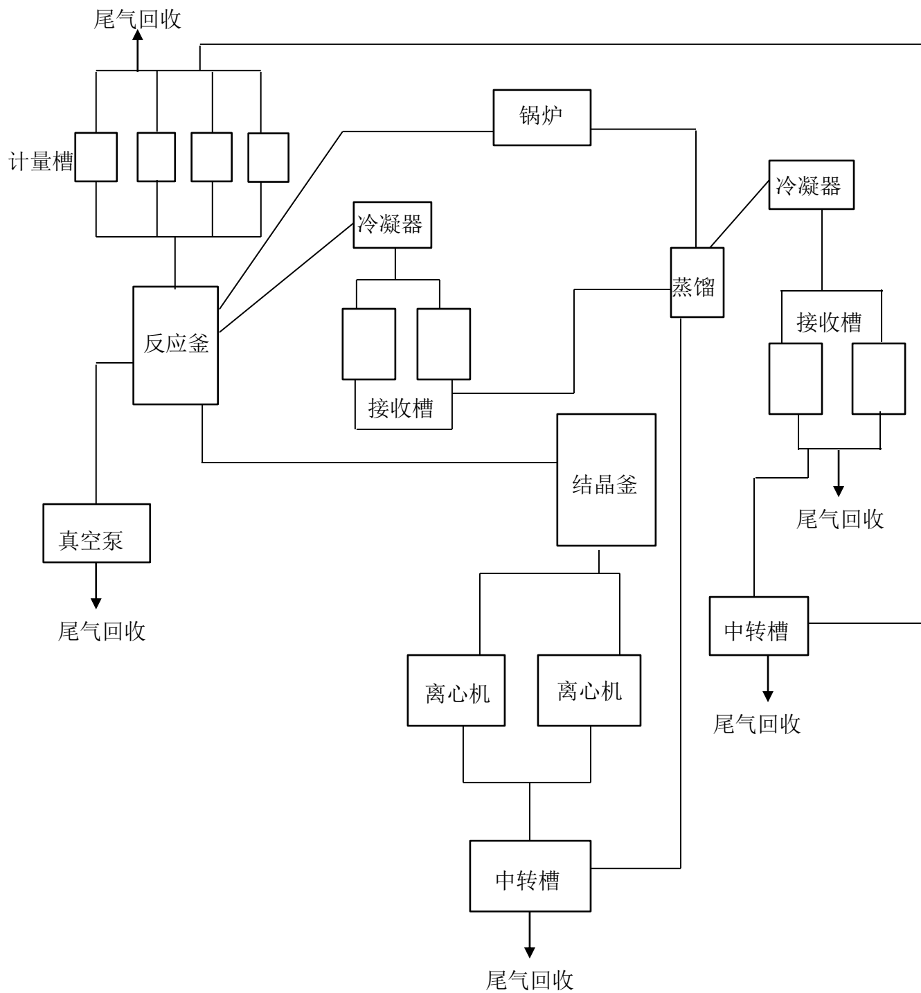
图 3.5-2 设备联接示意图
