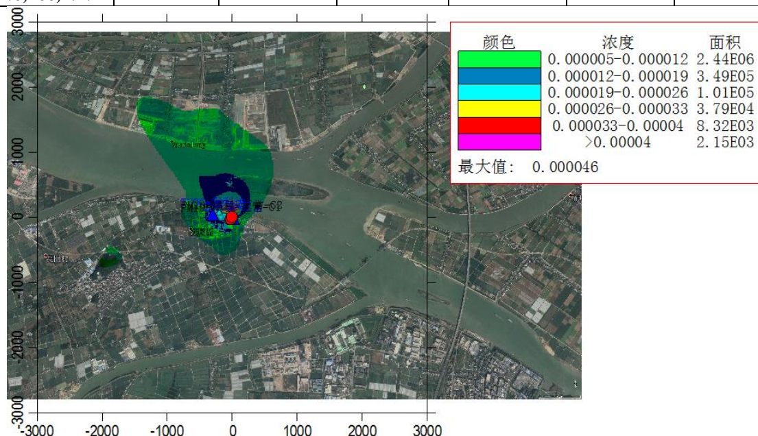
图 6.1-12 PM10 日均浓度贡献值等值线图(单位: mg/m 3 )
