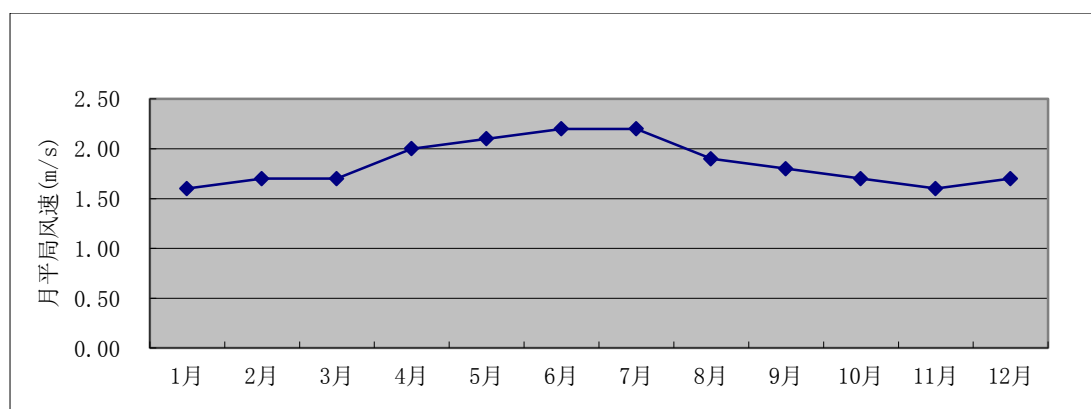
图 6.1-2 中山市 1997~2016 年逐月平均风速变化曲线
