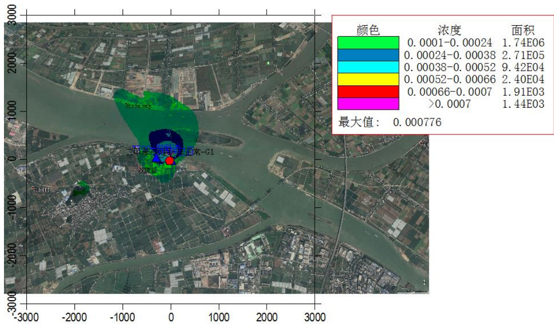
图 6.1-17 二甲苯时均浓度贡献值等值线图(单位: mg/m 3 )
