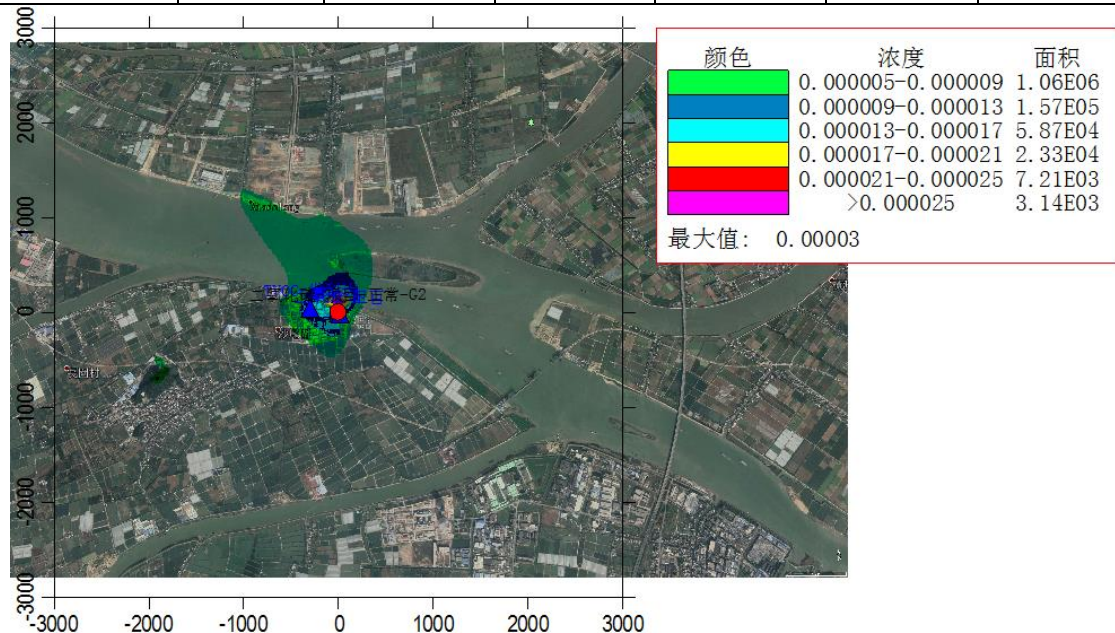
图 6.1-14 二氧化硫时均浓度贡献值等值线图(单位: mg/m 3 )
