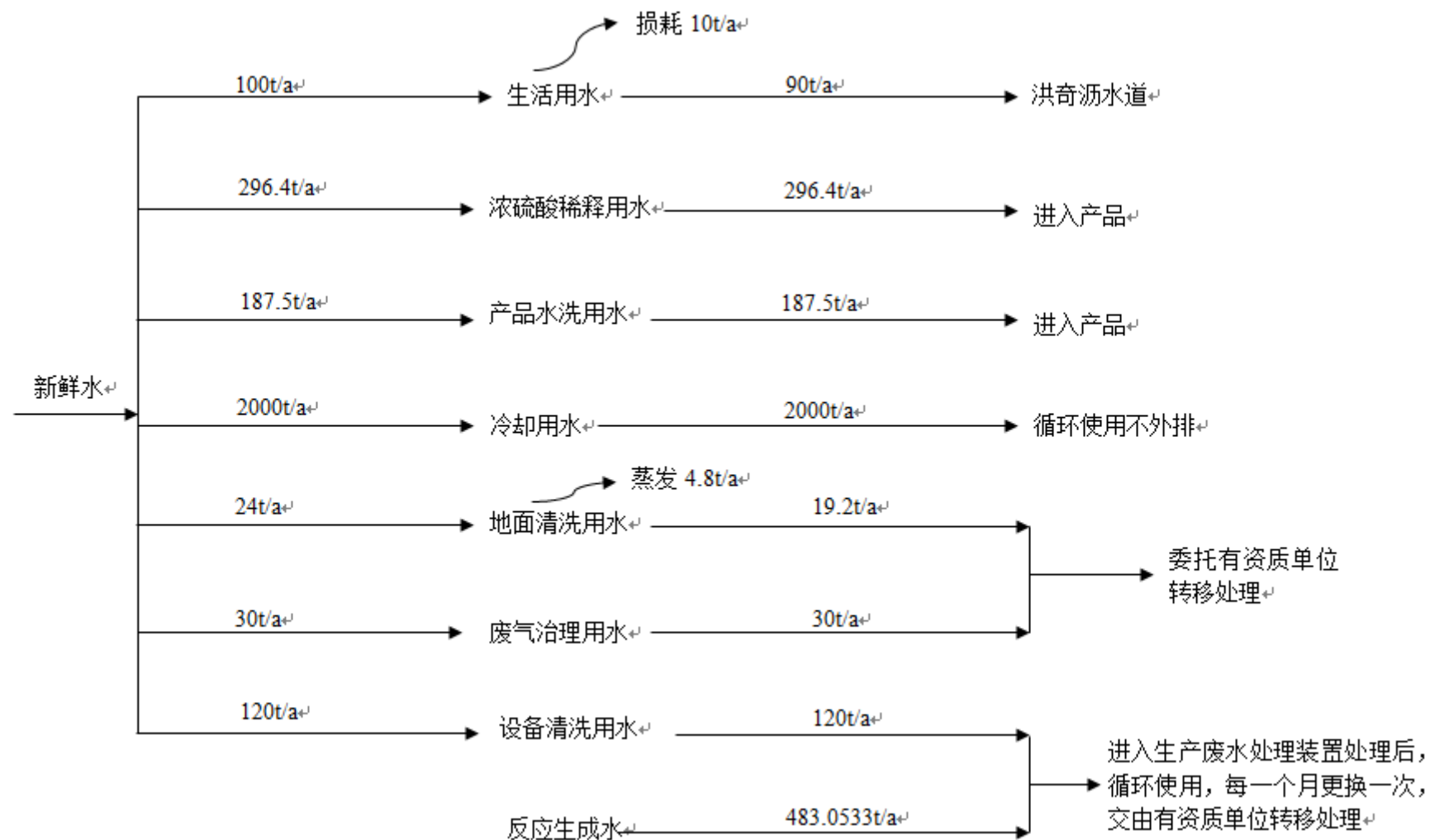
图 4.3-1 水平衡图 (单位 t/a)
