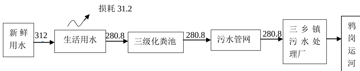
扩建后项目水平衡图（t/a）
